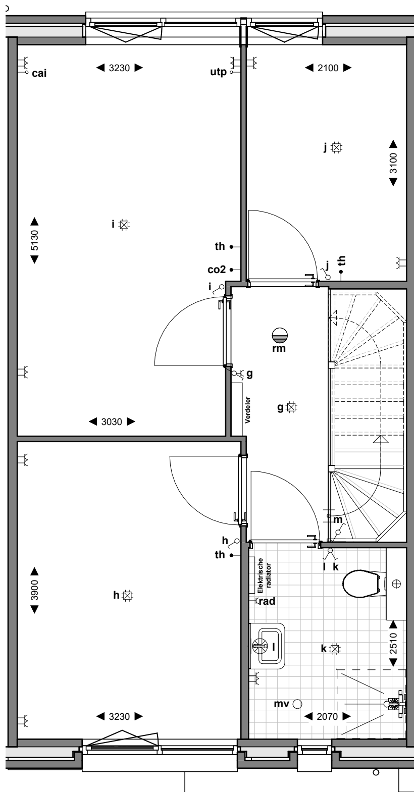
eerste verdieping
