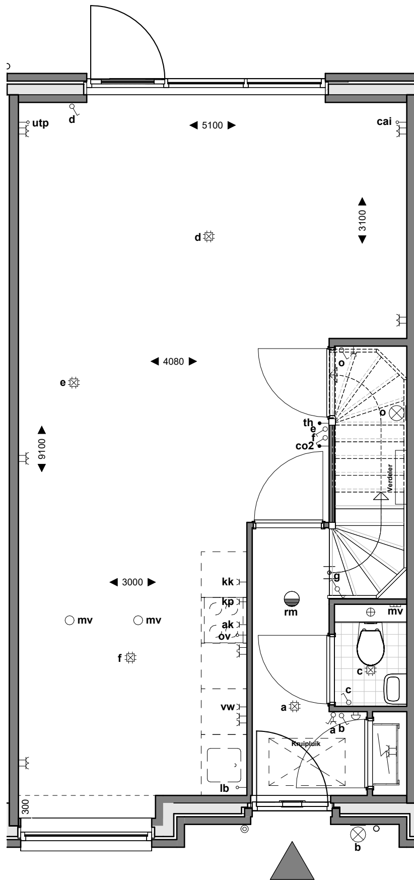
begane grond
