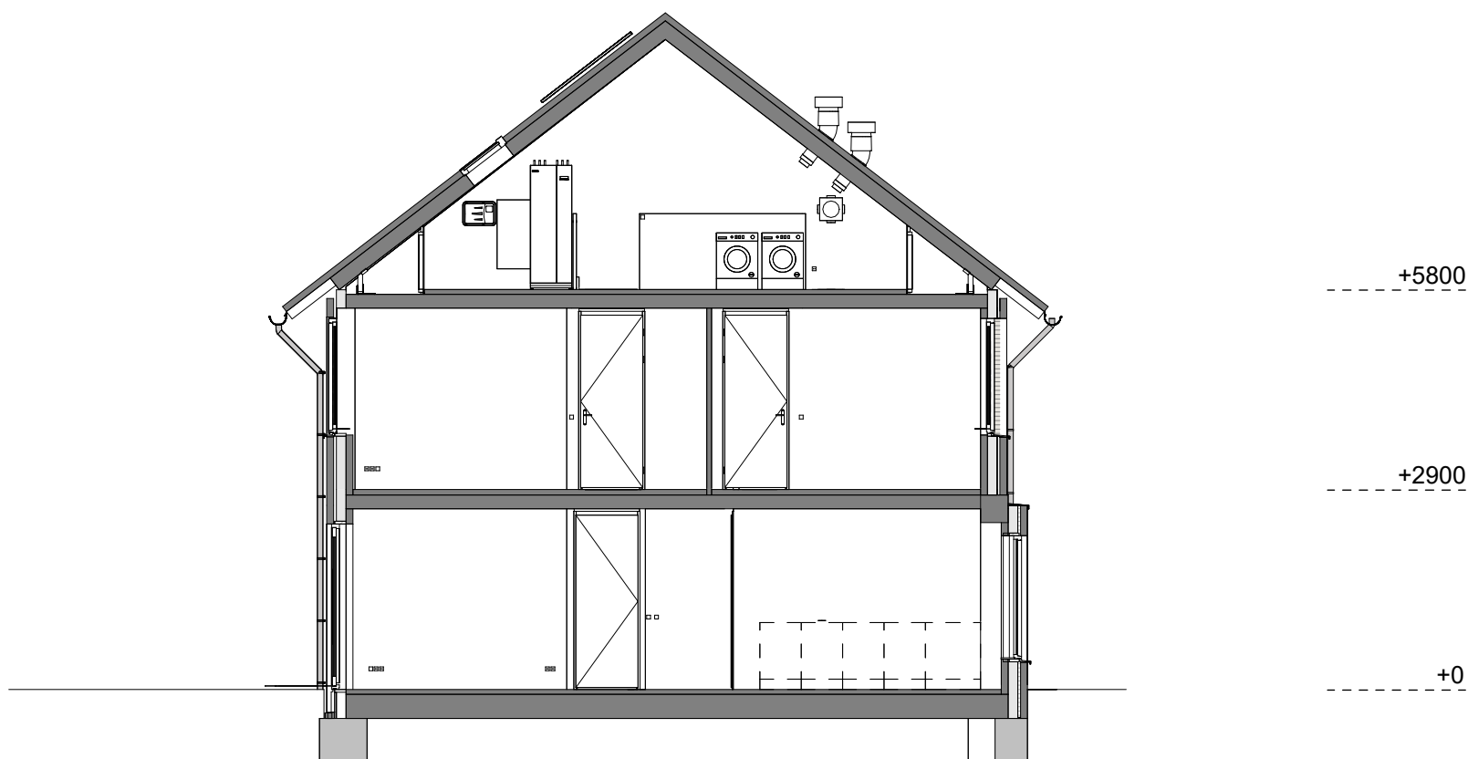
Doorsnede
