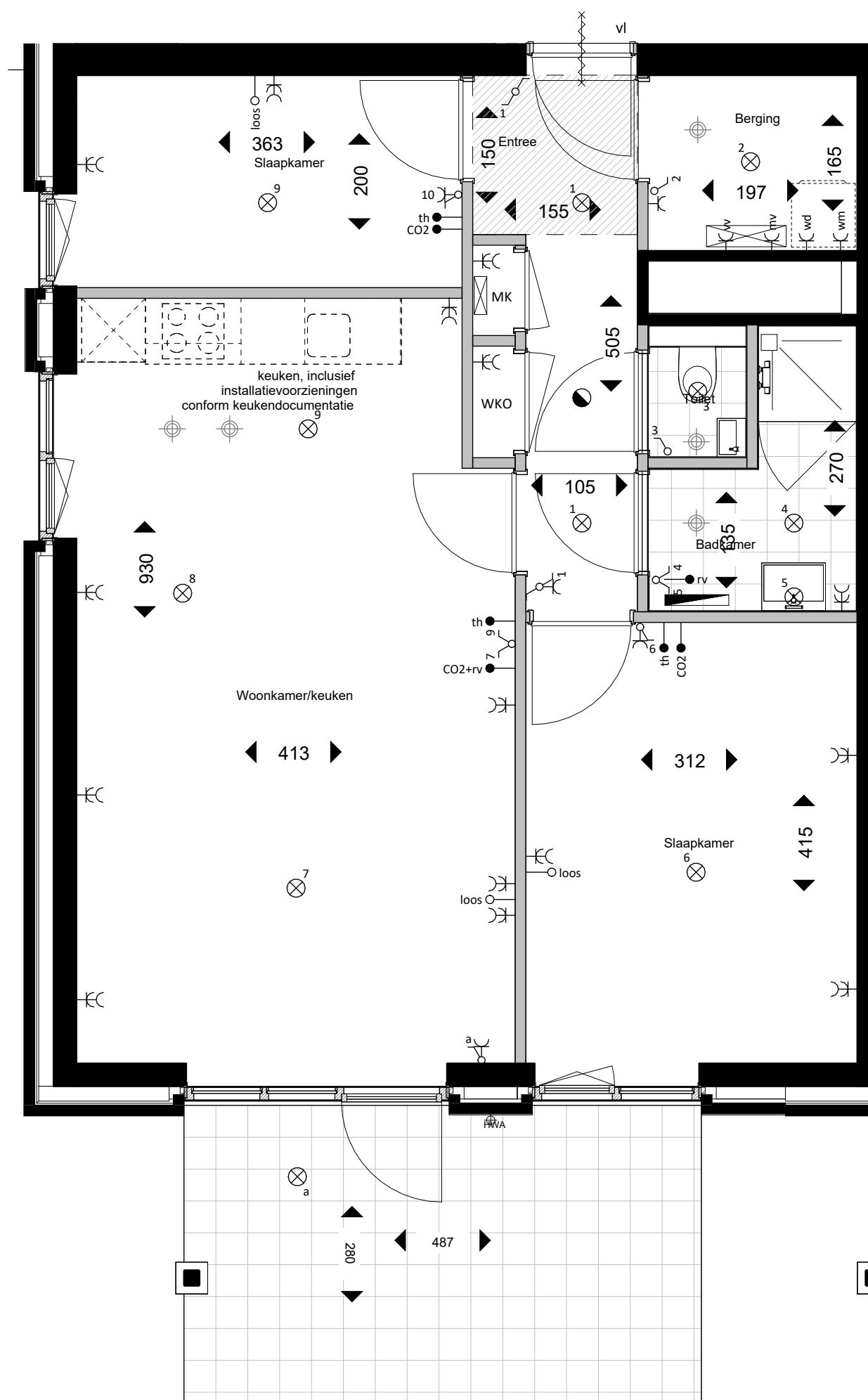
Plattegrond 1:50
