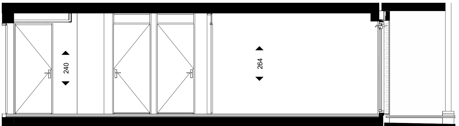
lengtedoorsnede 1:50
