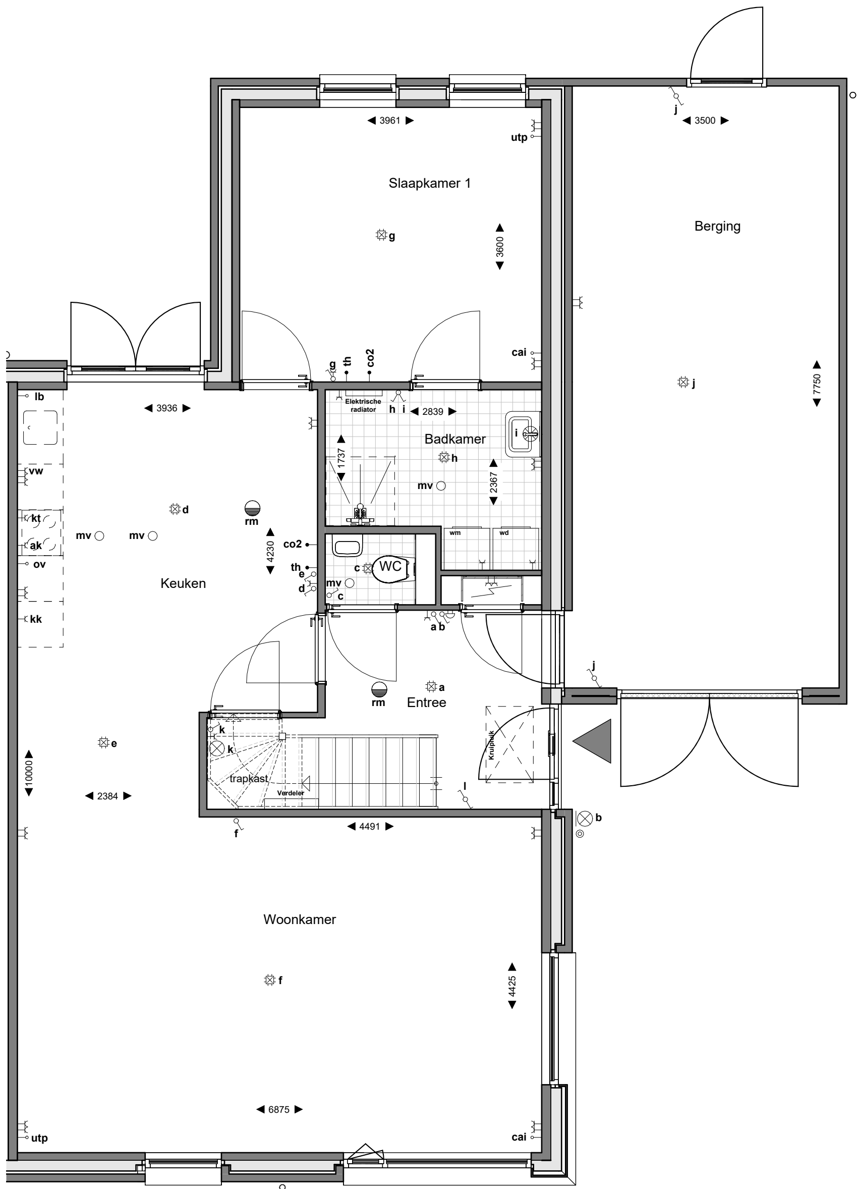
begane grond
