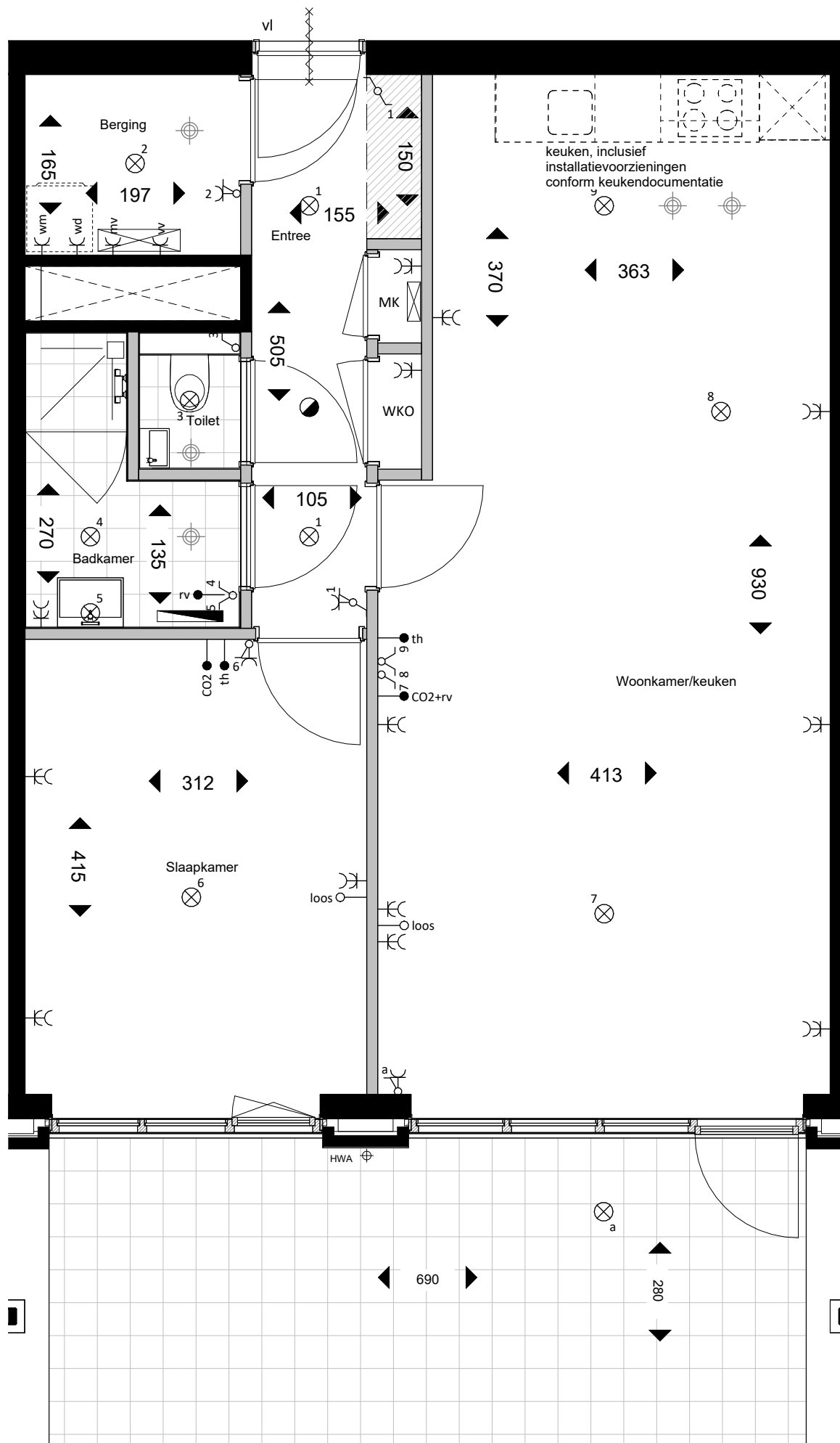
Plattegrond 1:50
