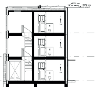
Doorsnede
