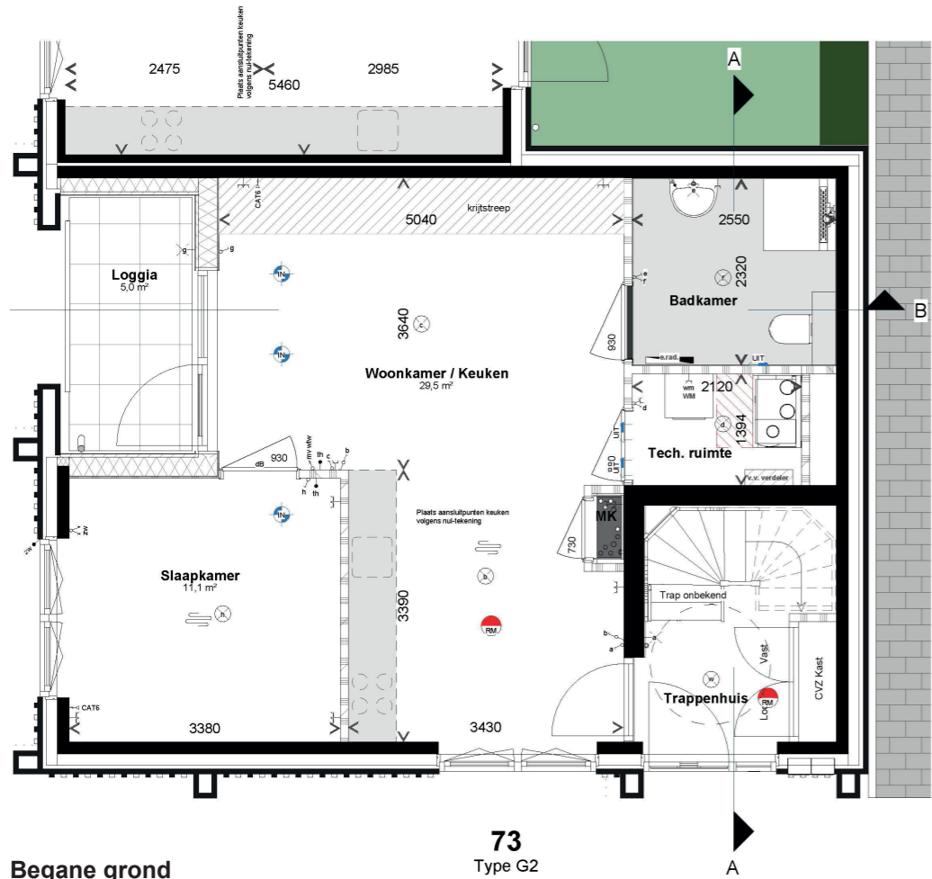
Begane grond
