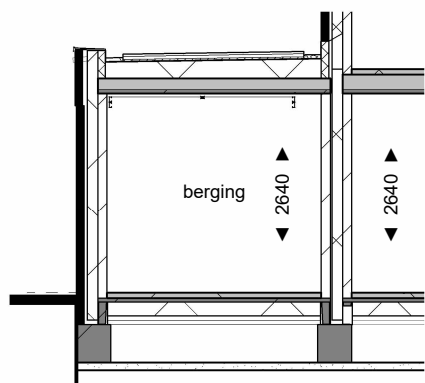
Doorsnede C-C
