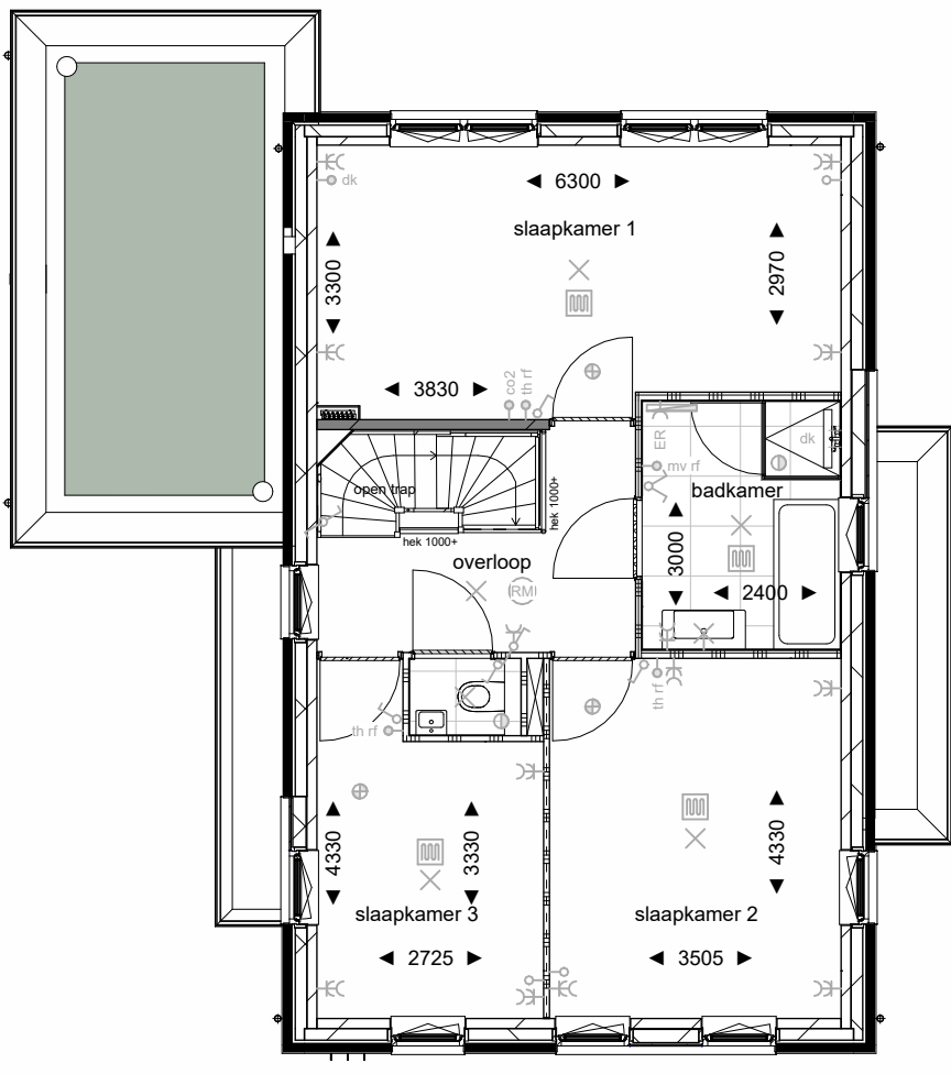
Eerste verdieping
