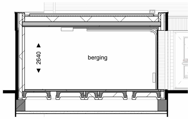
Doorsnede D-D
