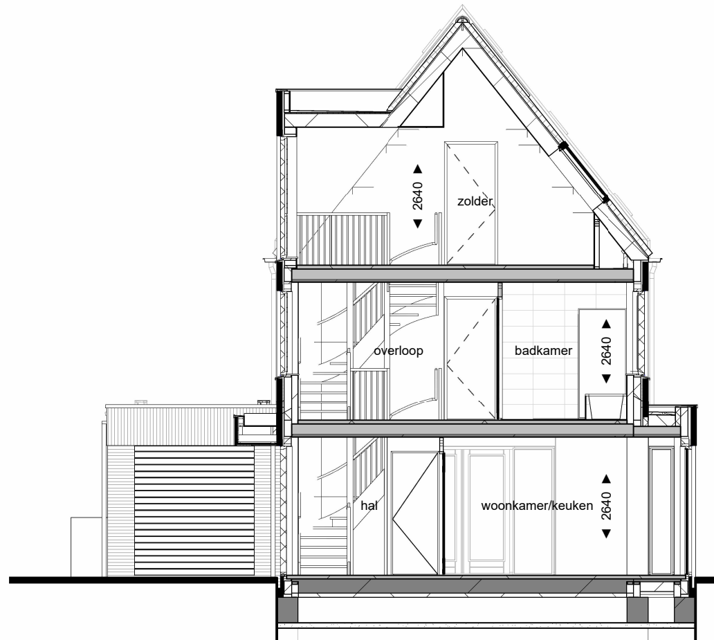
Doorsnede B-B
