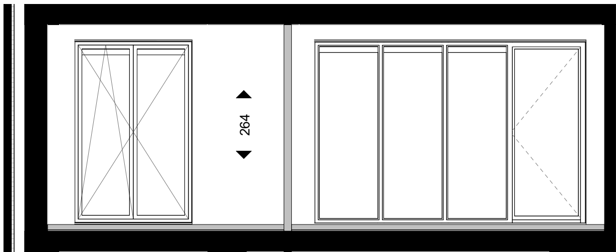
dwarsdoorsnede 1:50
