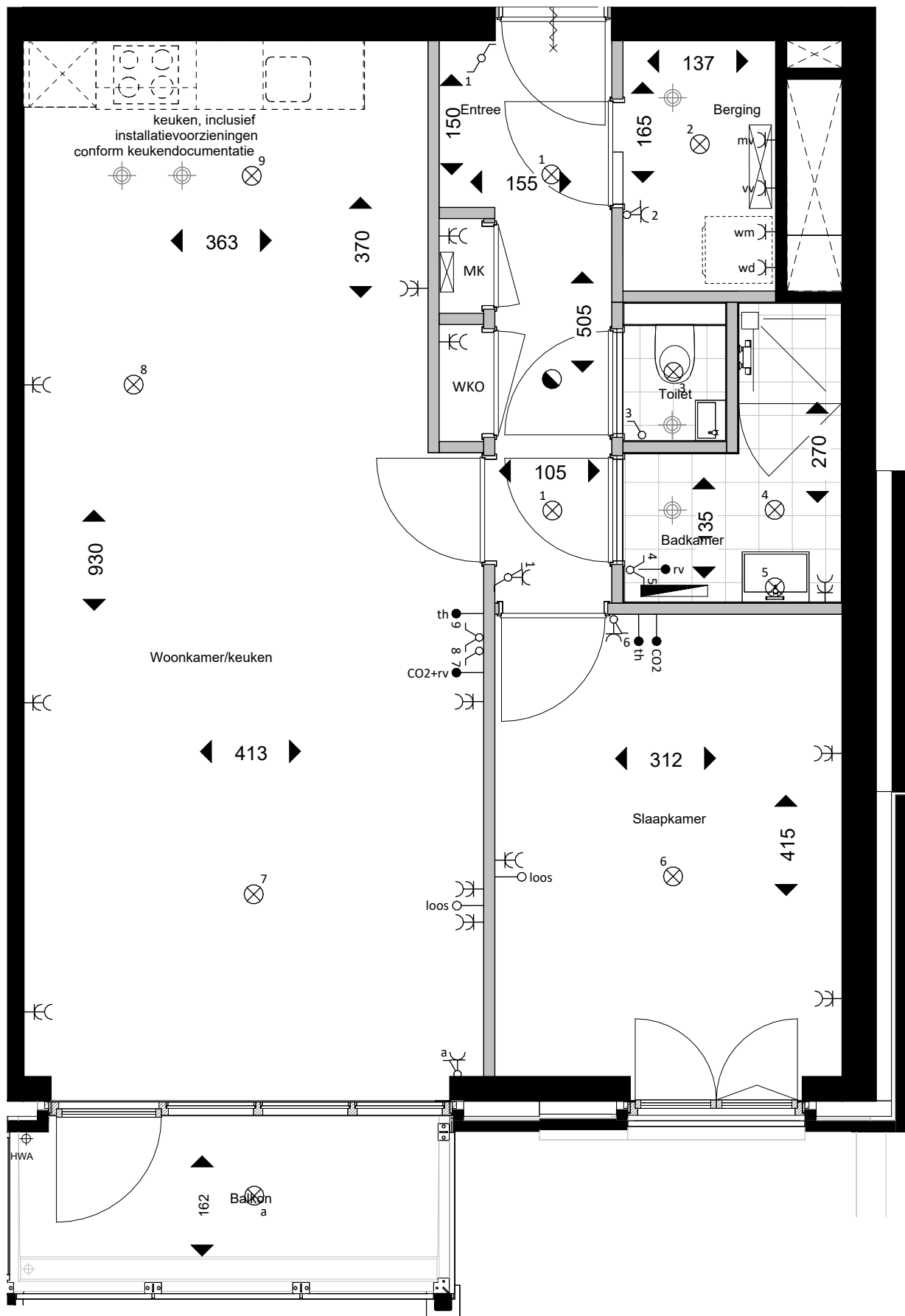
Plattegrond 1:50
