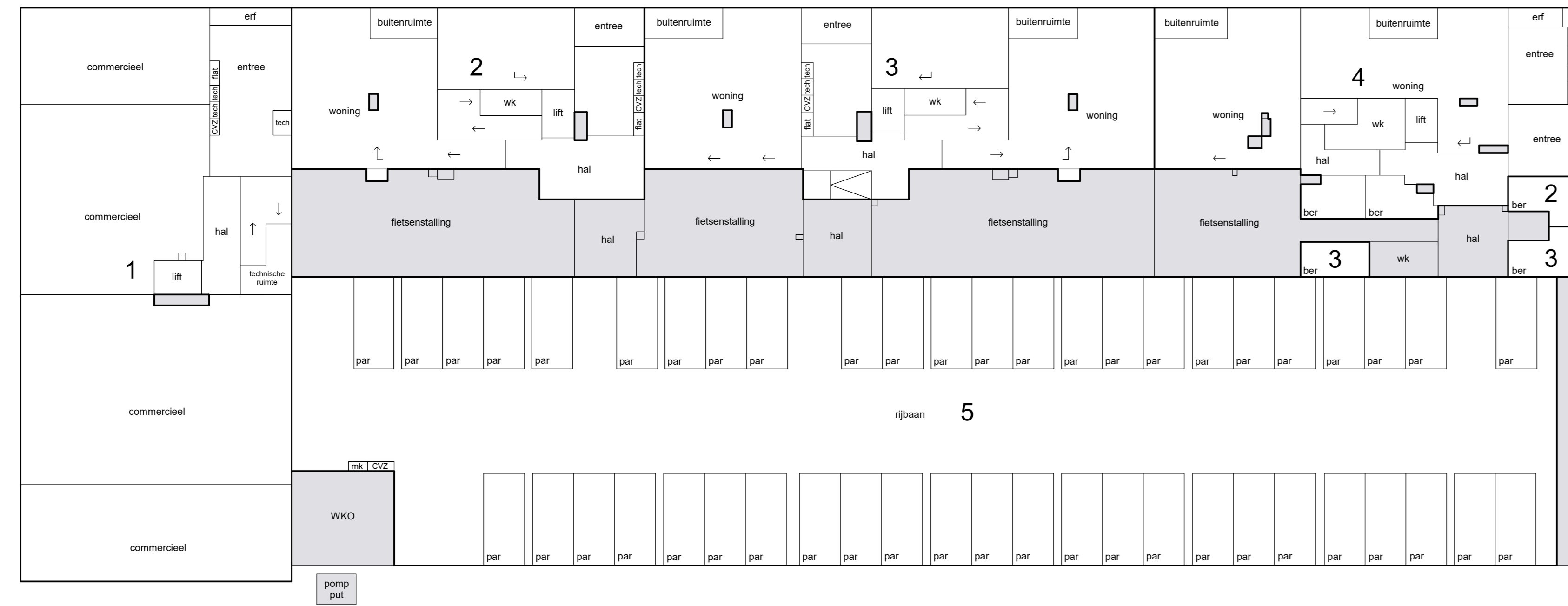
begane grond
