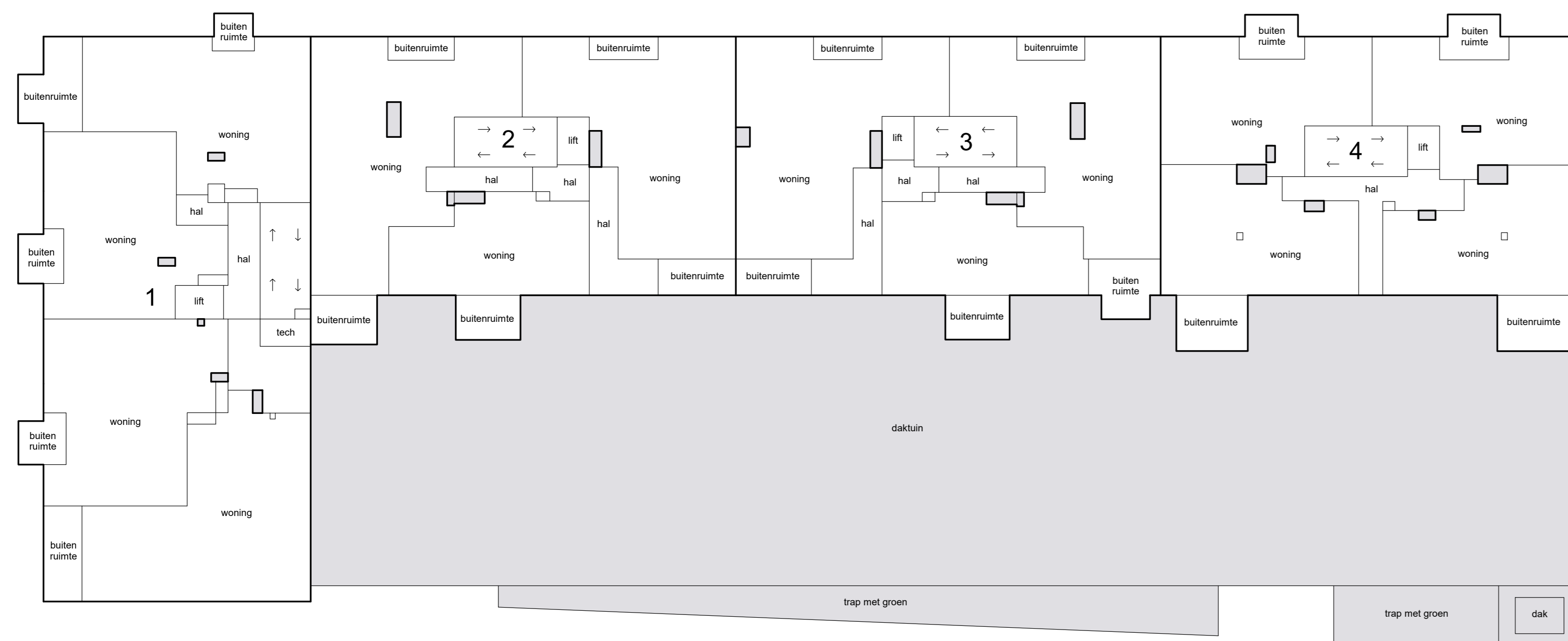
2e etage
