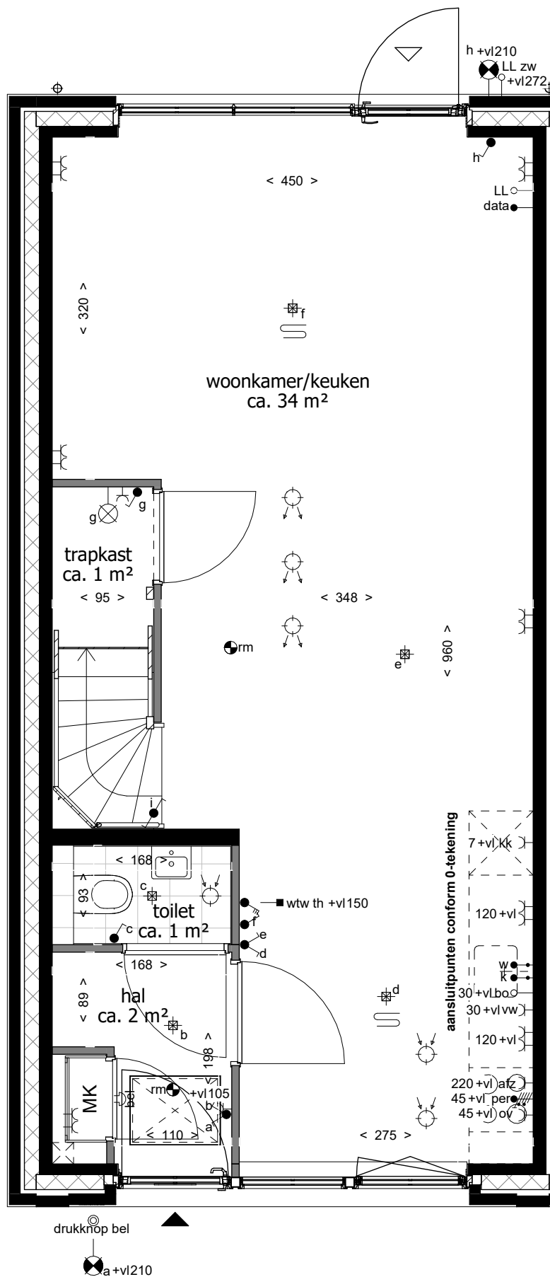
Begane grond
