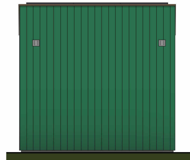
Achtergevel
