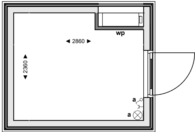
begane grond
