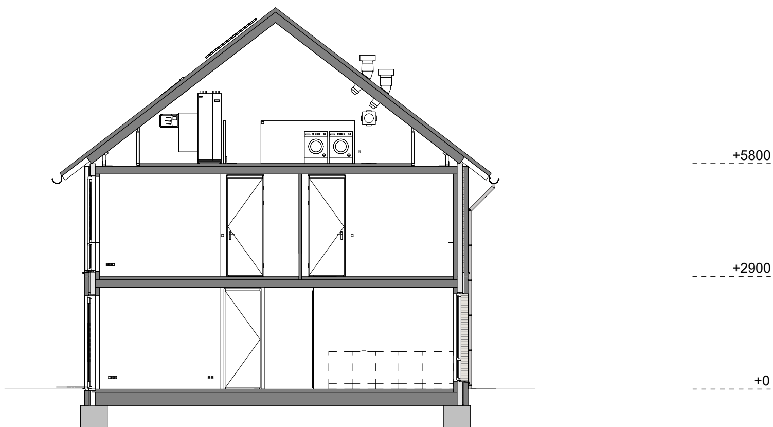
Doorsnede
