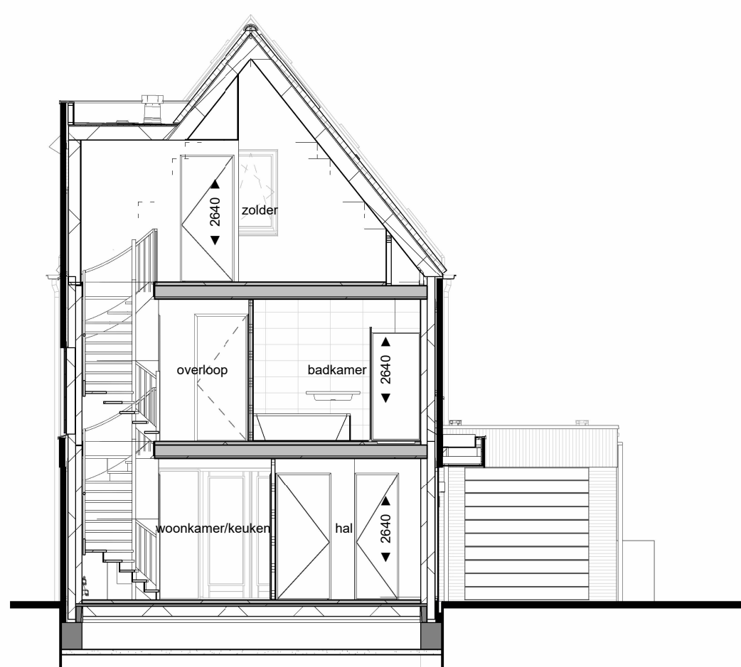
Doorsnede B-B
