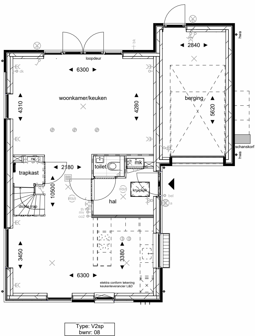
Begane grond
