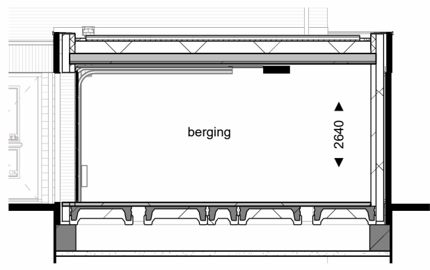
Doorsnede D-D
