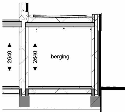
Doorsnede C-C
