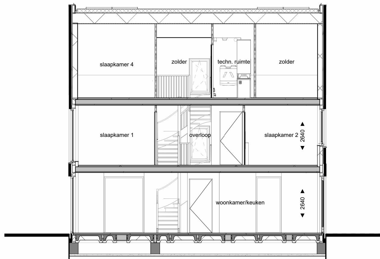
Doorsnede A-A
