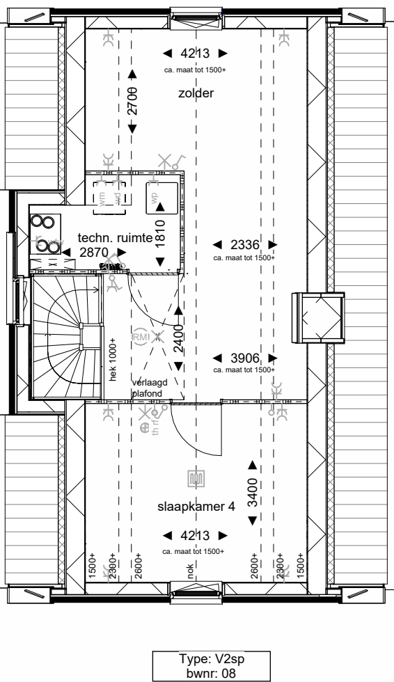
Tweede verdieping
