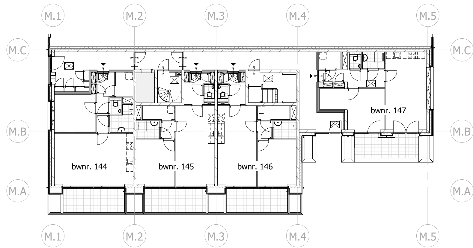
begane grond
