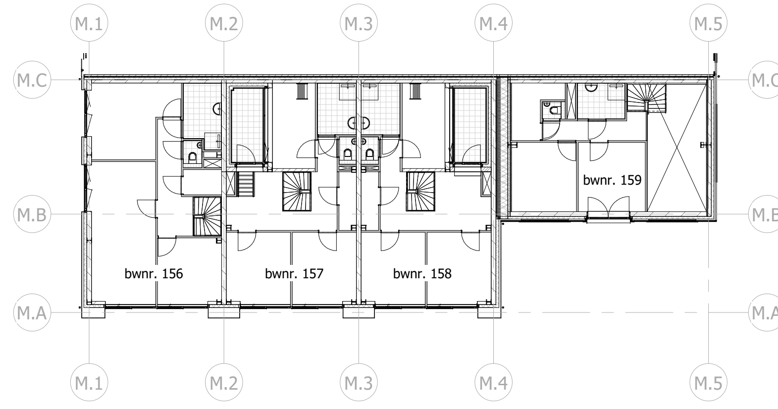
vierde verdieping
