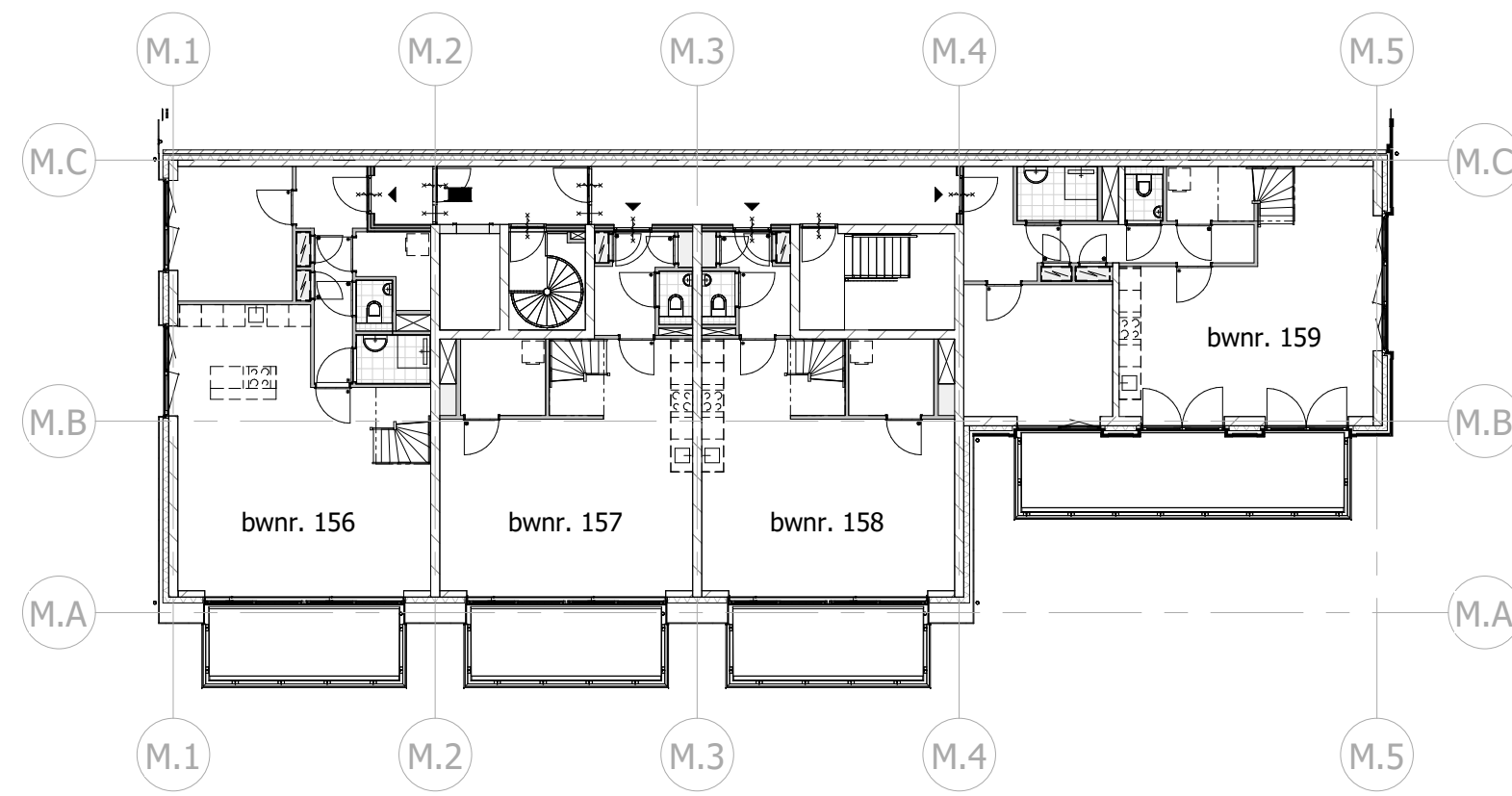
derde verdieping
