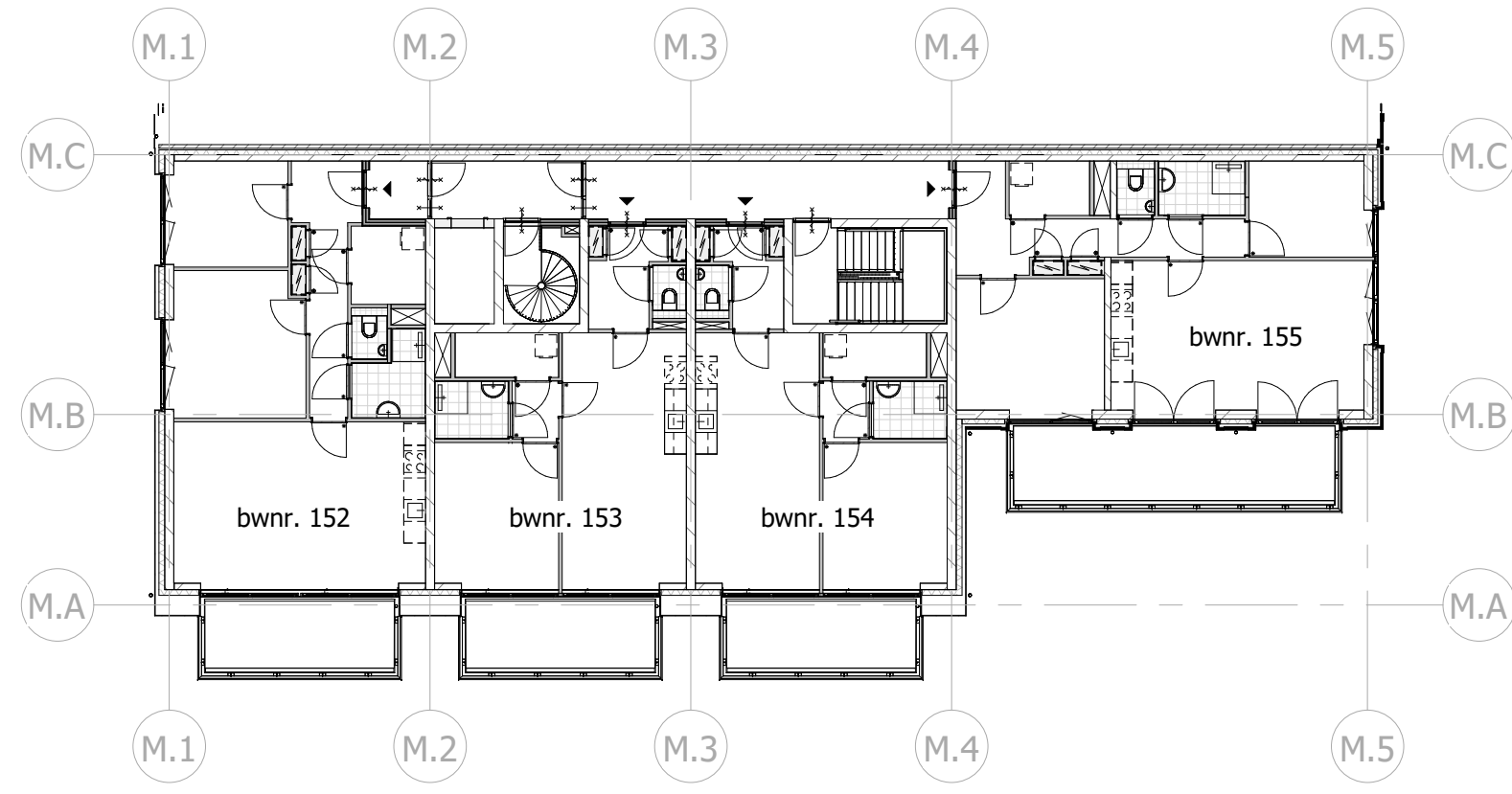
tweede verdieping
