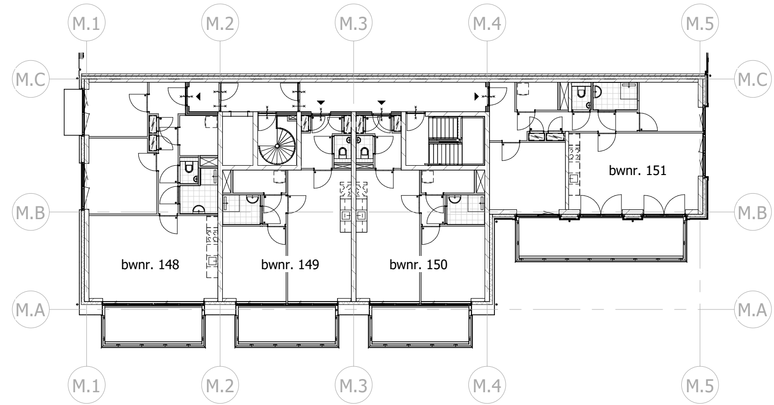
eerste verdieping
