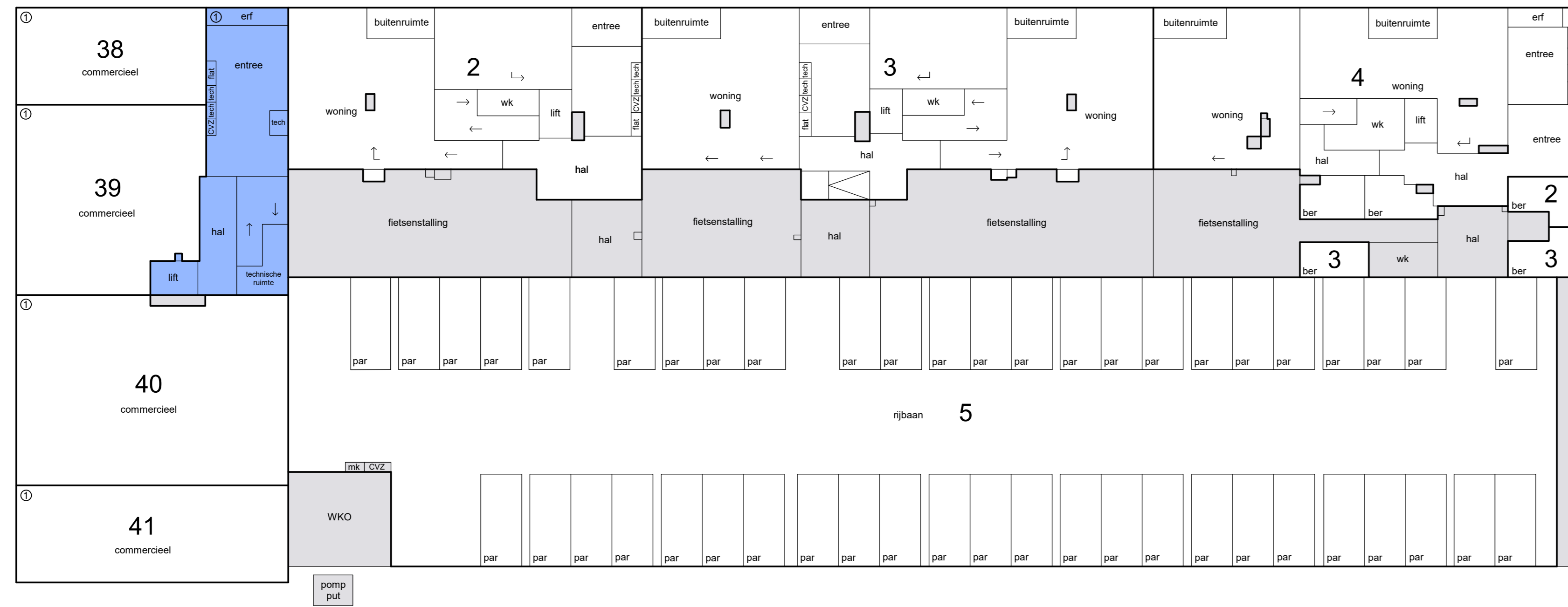
begane grond
