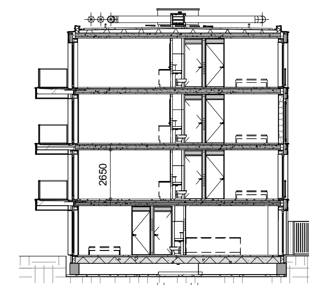
Doorsnede
