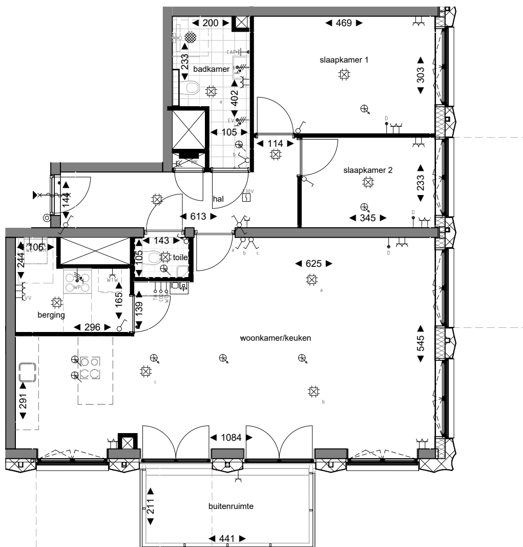
5e verdieping
