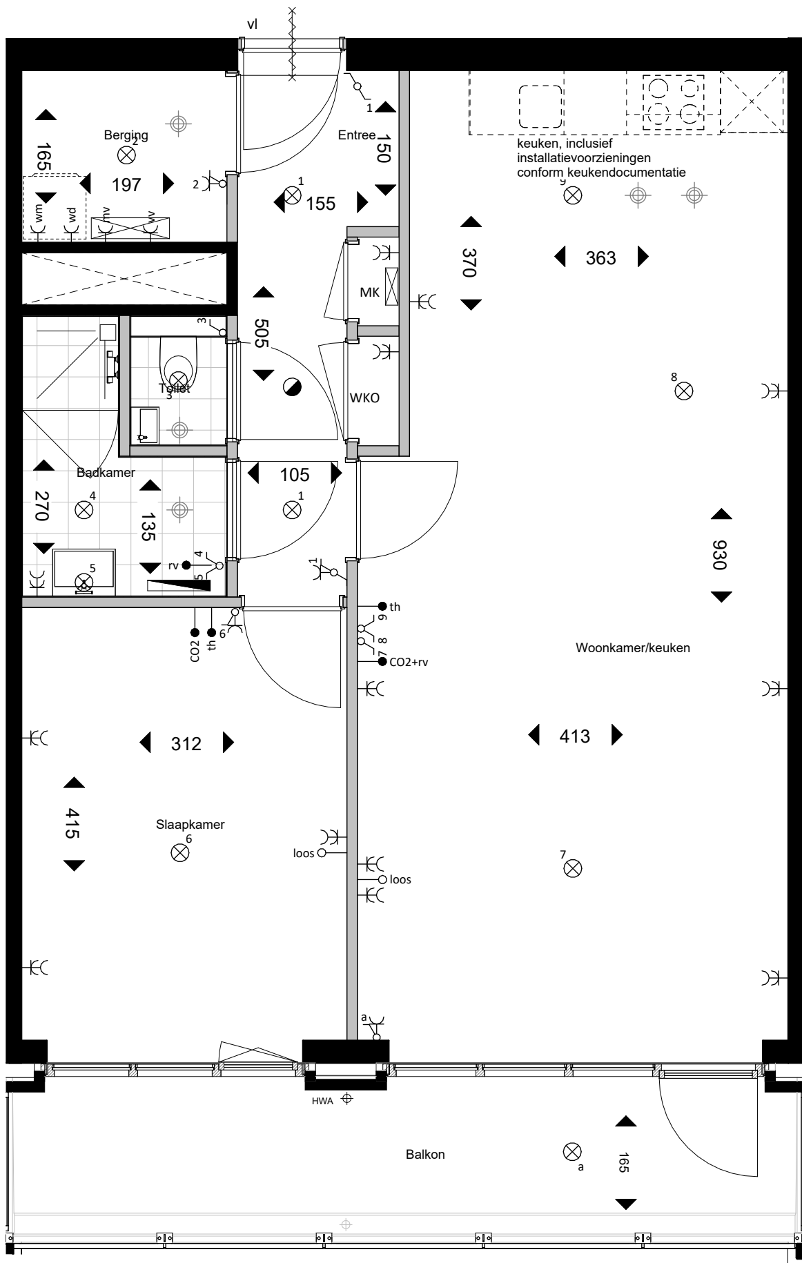
Plattegrond 1:50
