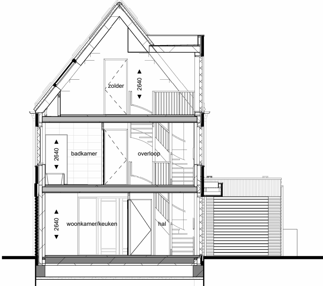
Doorsnede B-B
