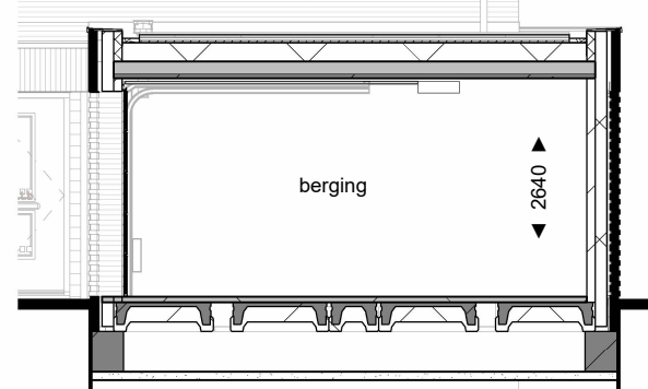
Doorsnede D-D
