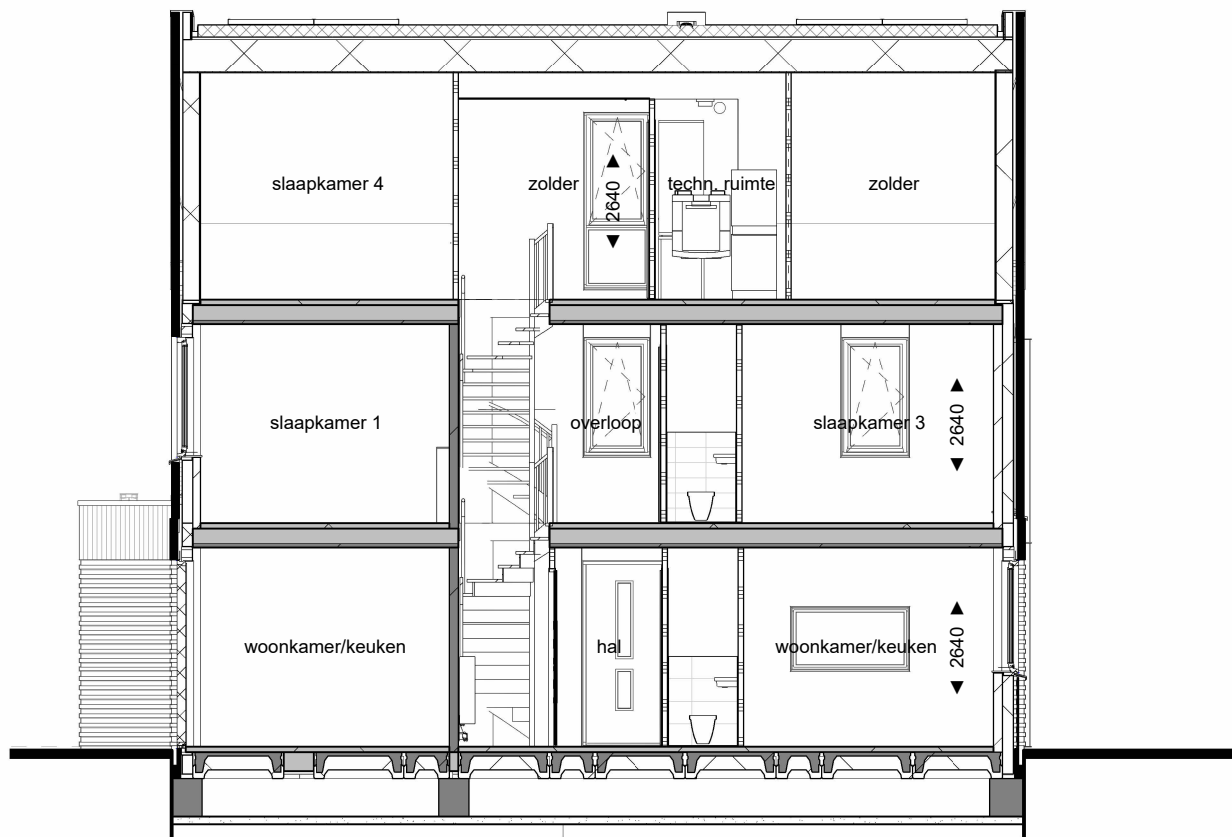
Doorsnede A-A
