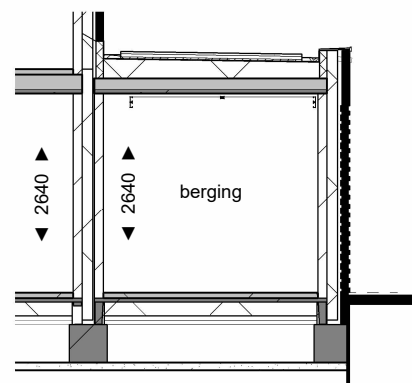
Doorsnede C-C
