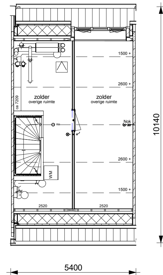
Optie 0555 + 0560: dakkapel en variant 1 scheidingswand op zolder
