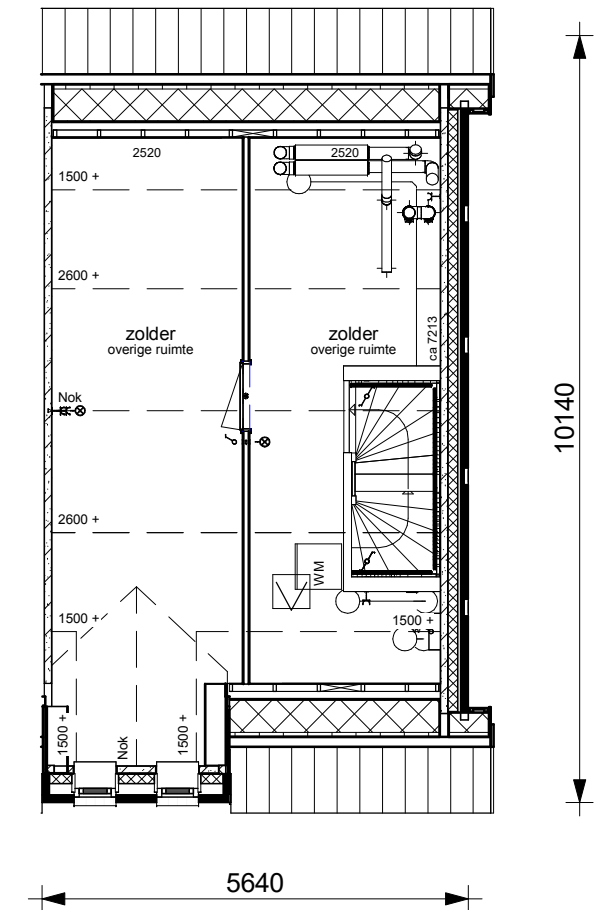
Optie 0560: variant 1 scheidingswand op zolder
