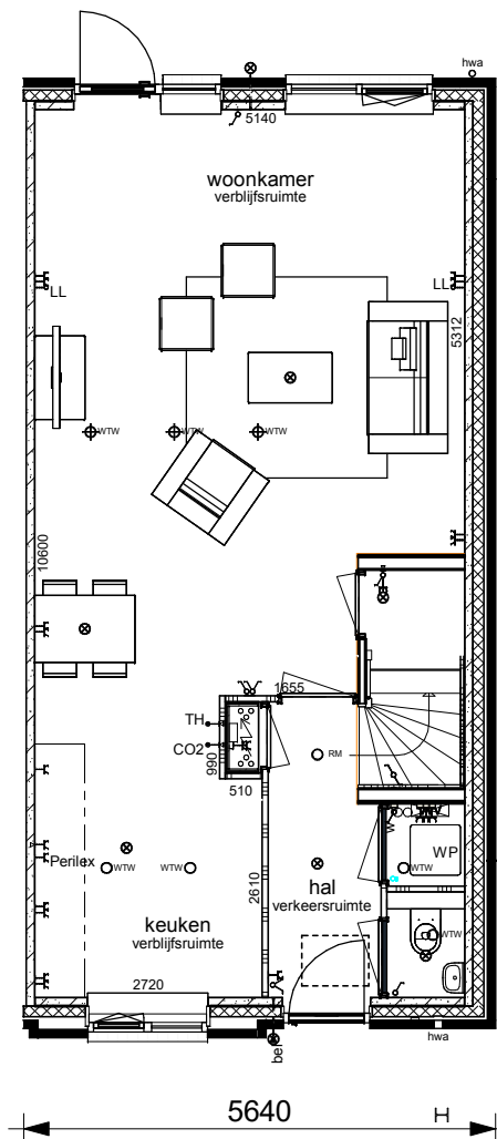
Optie 0305: 1200mm verlenging
