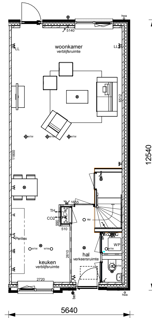
Optie 0310: 2400mm verlenging
