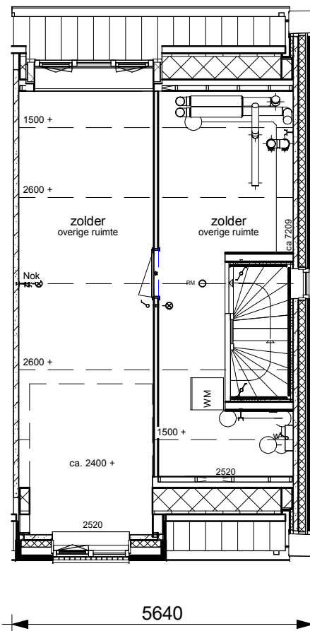
0555 + 0560: dakkapel en variant 1 scheidingswand op zolder
