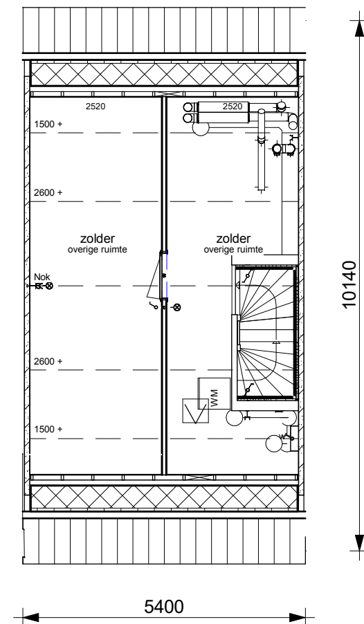
Optie 0560: variant 1 scheidingswand op zolder
