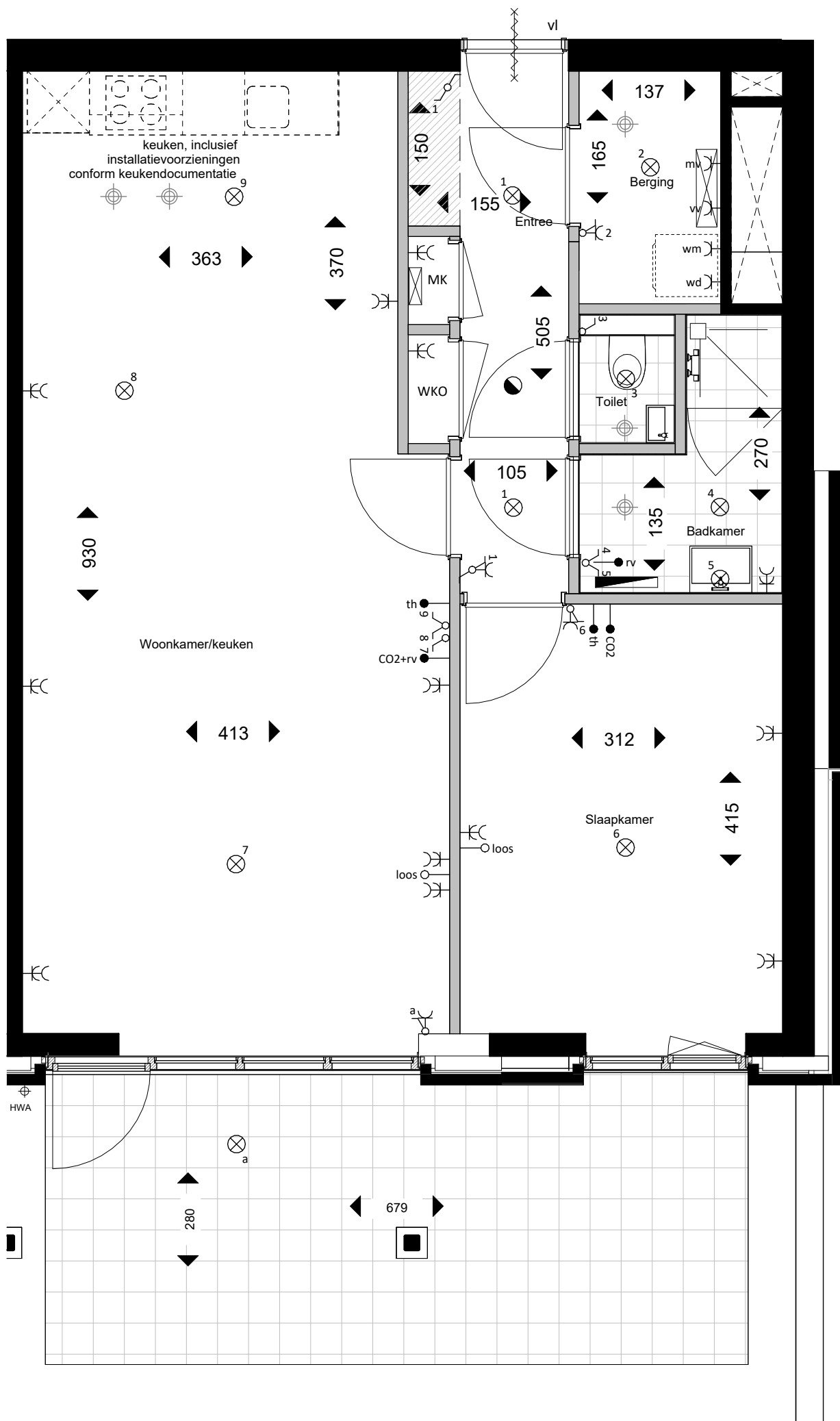
Plattegrond 1:50
