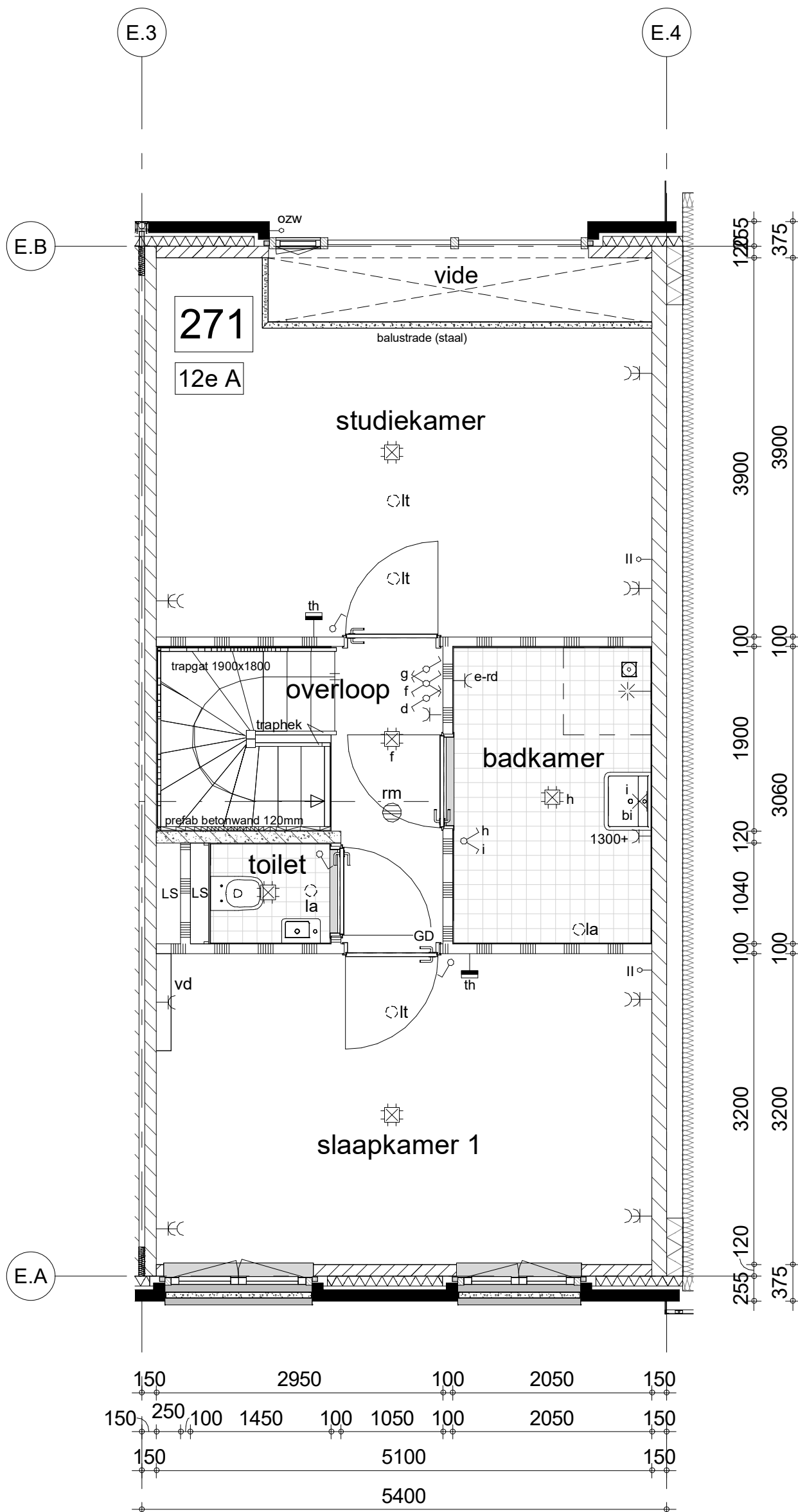
eerste verdieping
