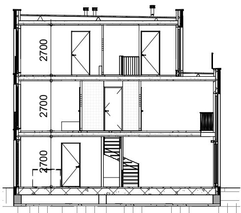
Doorsnede
