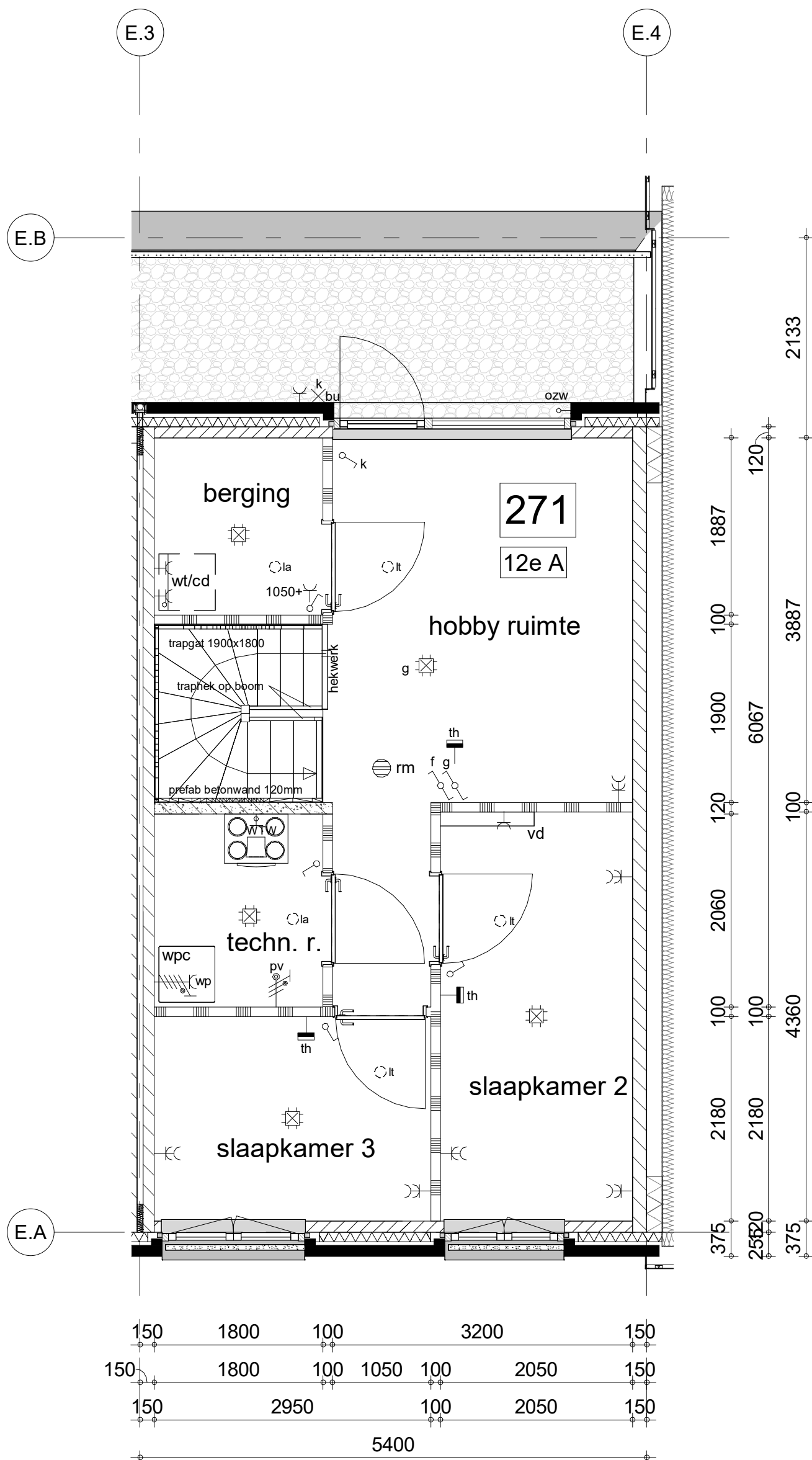
tweede verdieping
