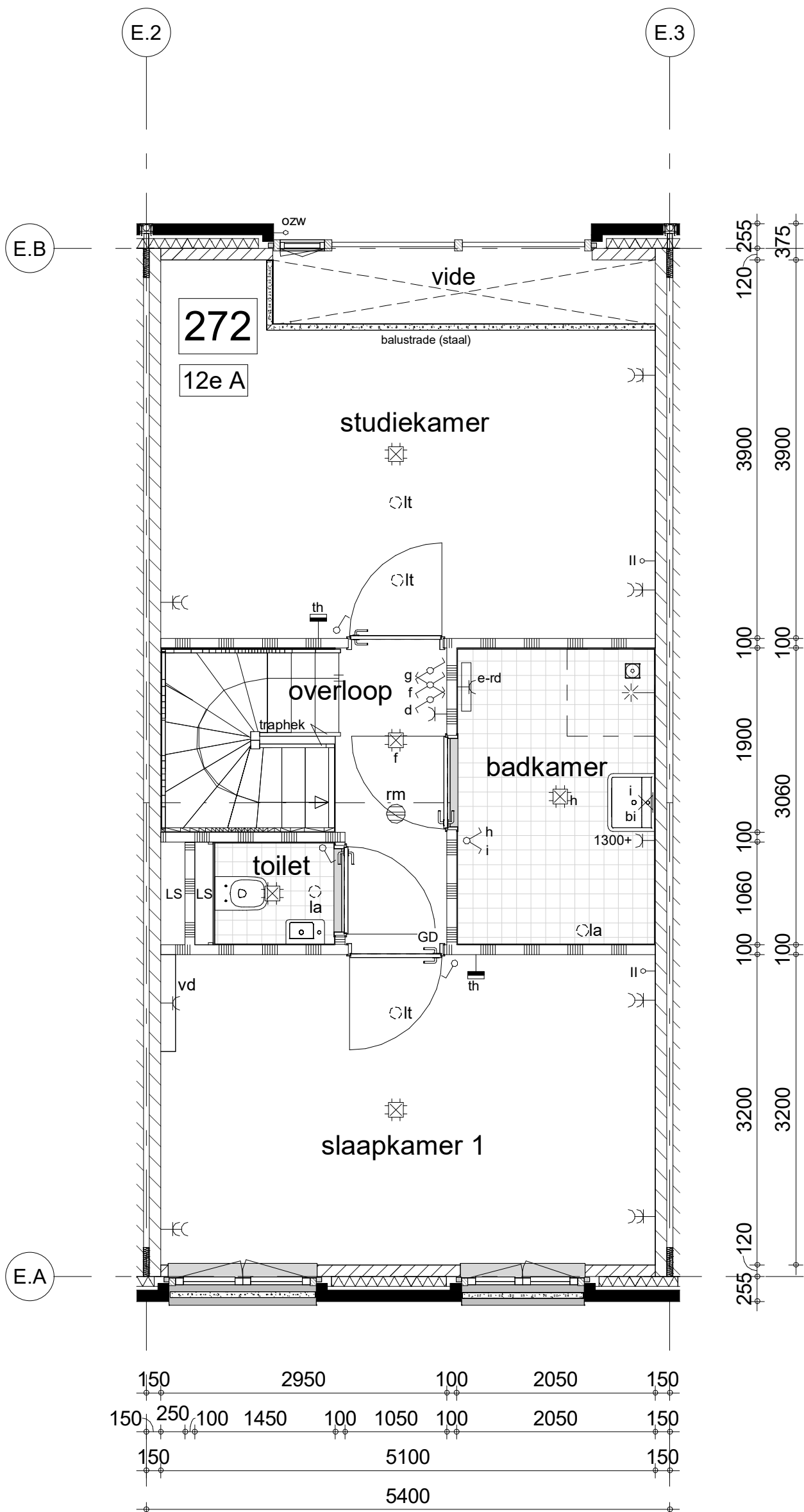
eerste verdieping
