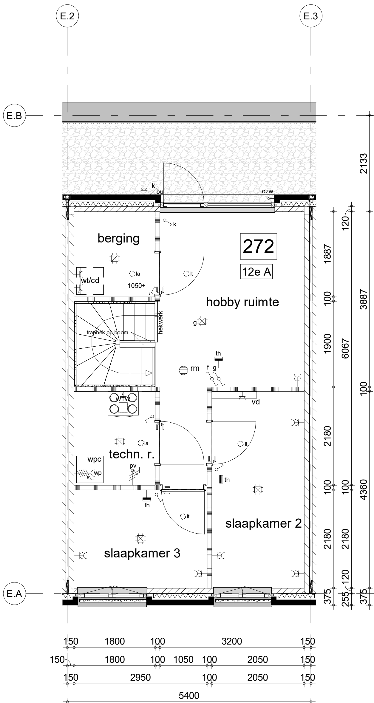
tweede verdieping
