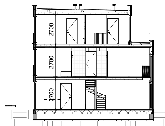
Doorsnede
