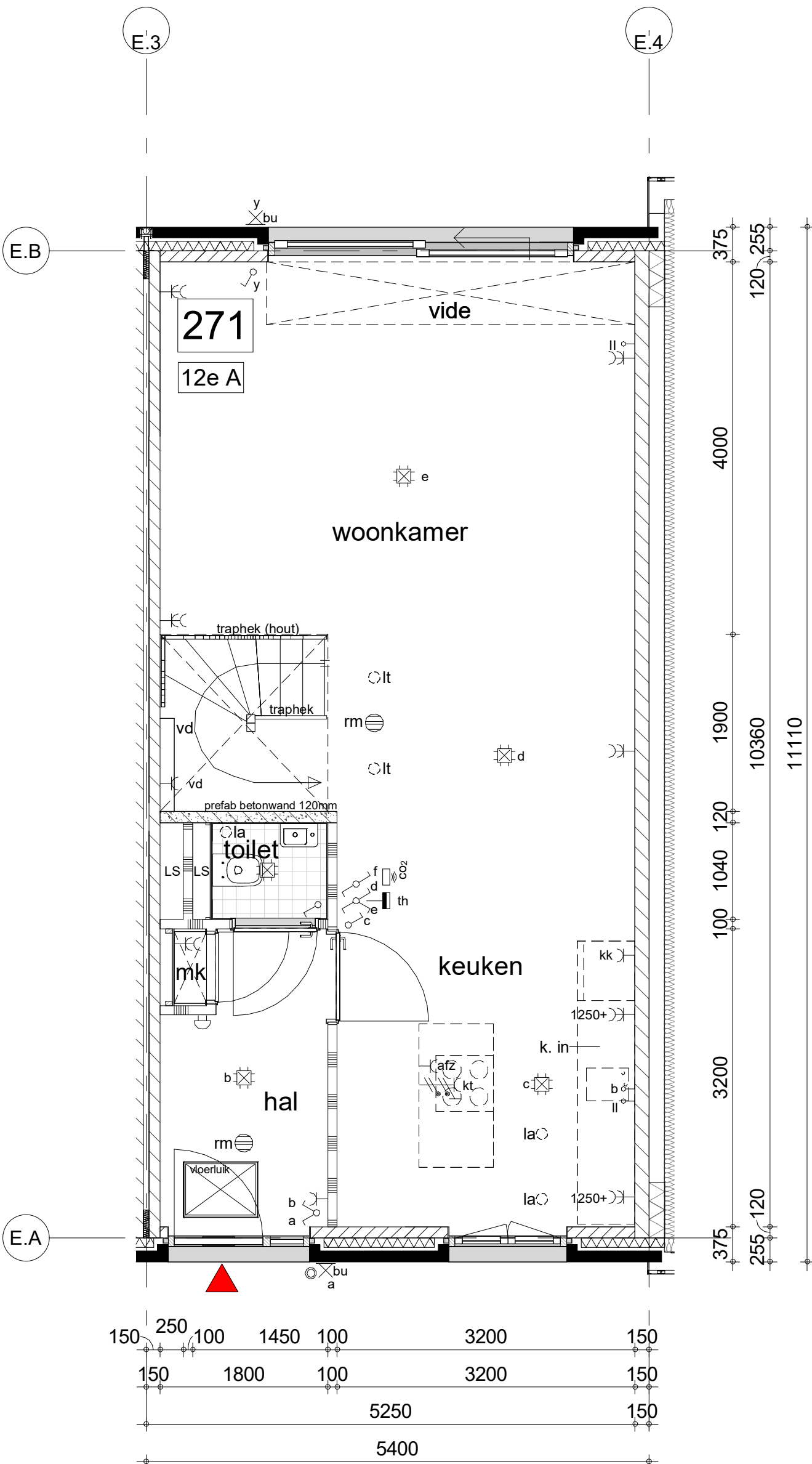
begane grond
