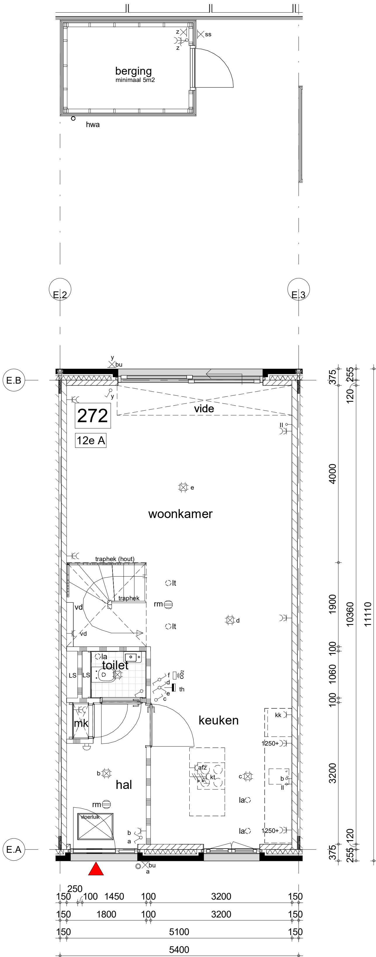
begane grond
