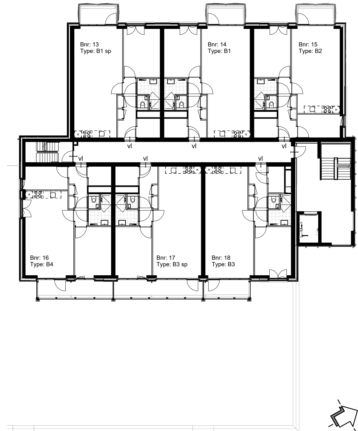
Derde verdieping 1:200
