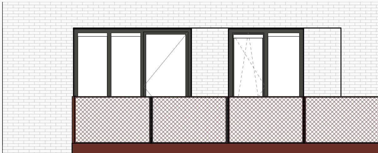
Gevelfragment Zuidoostgevel 1:50
