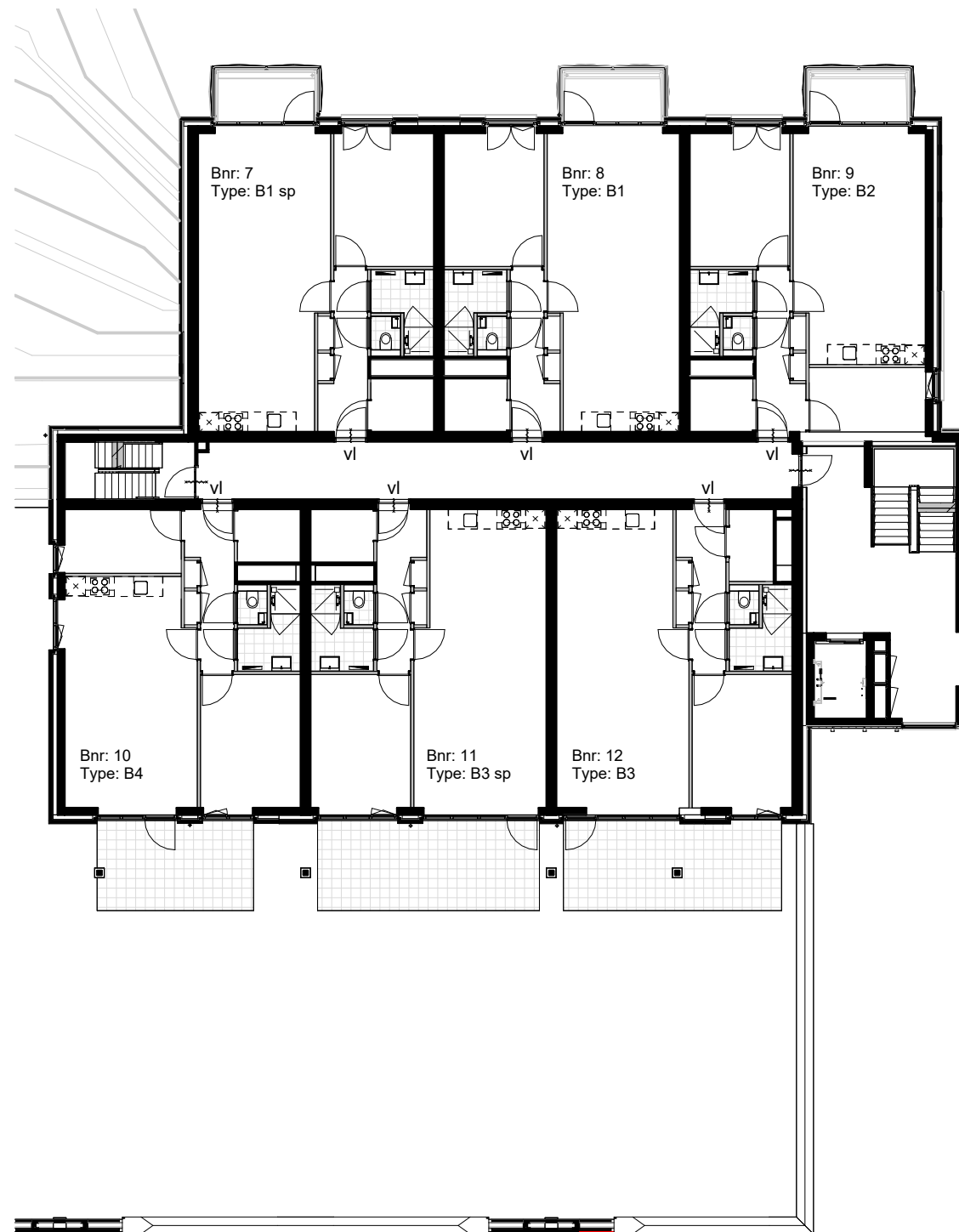
Tweede verdieping 1:200
