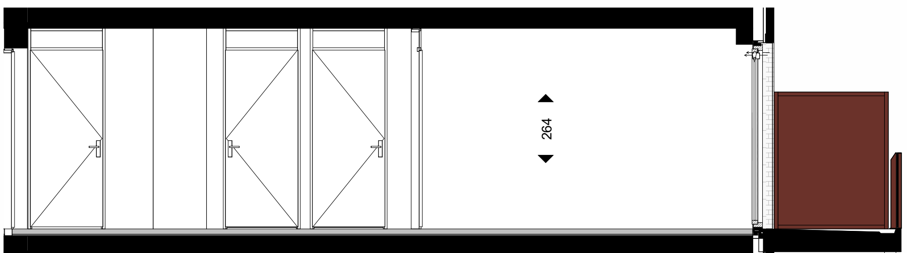
lengtedoorsnede 1:50
