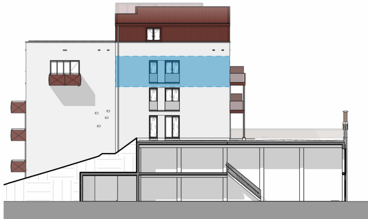
Zuidwestgevel 1:400
