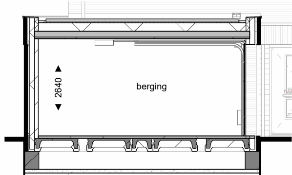
Doorsnede D-D
