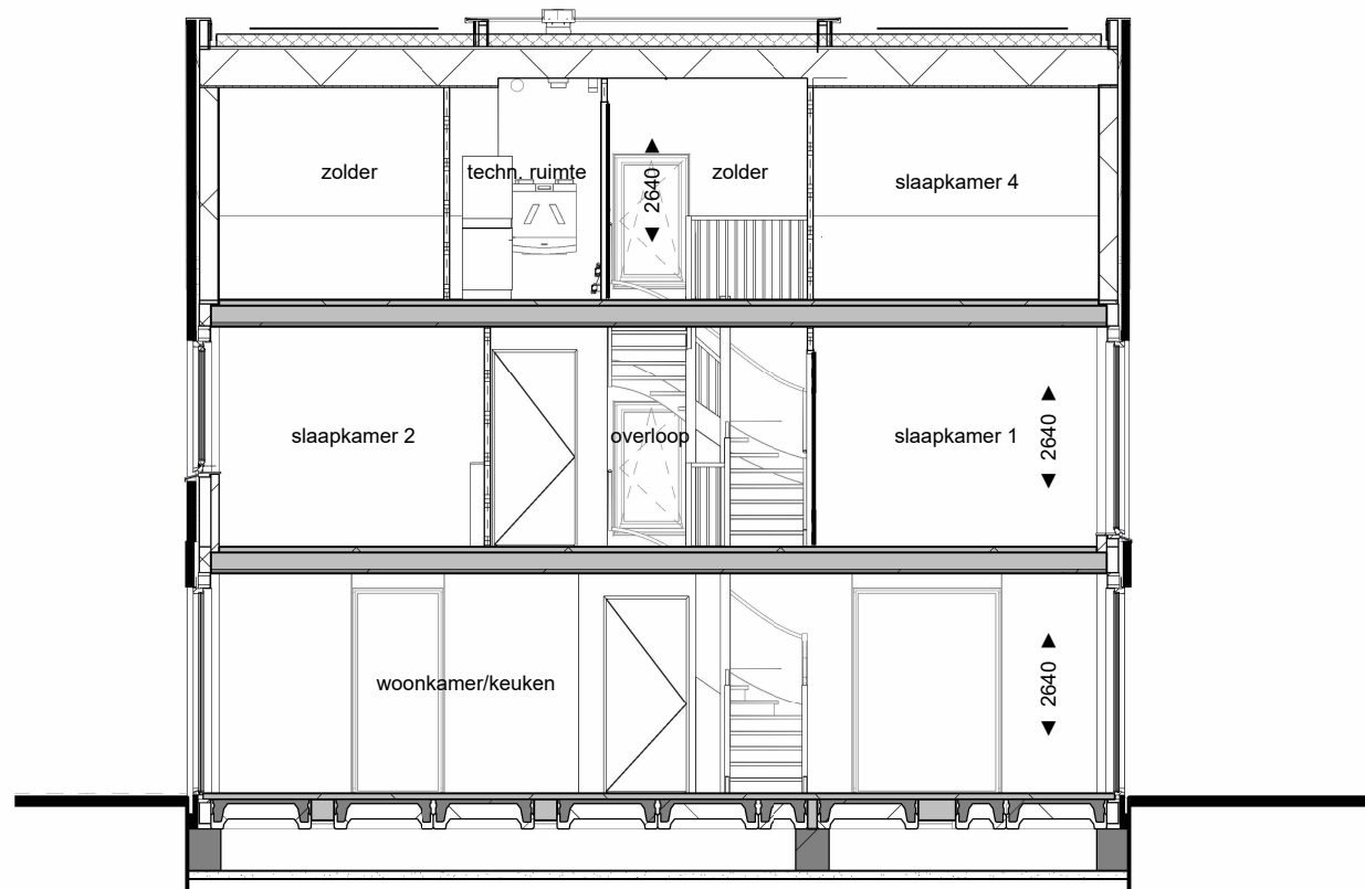
Doorsnede A-A
