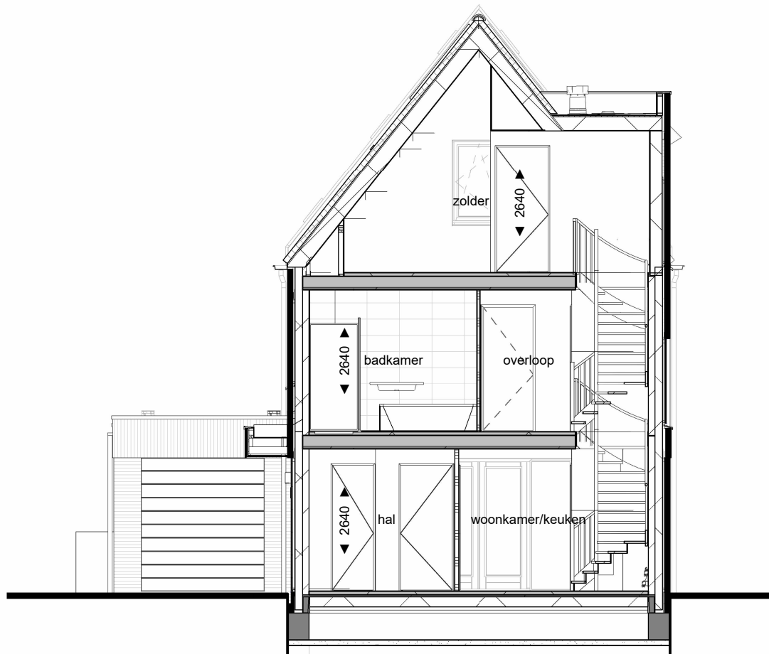
Doorsnede B-B
