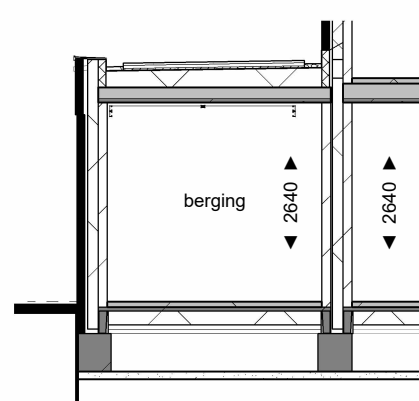
Doorsnede C-C
