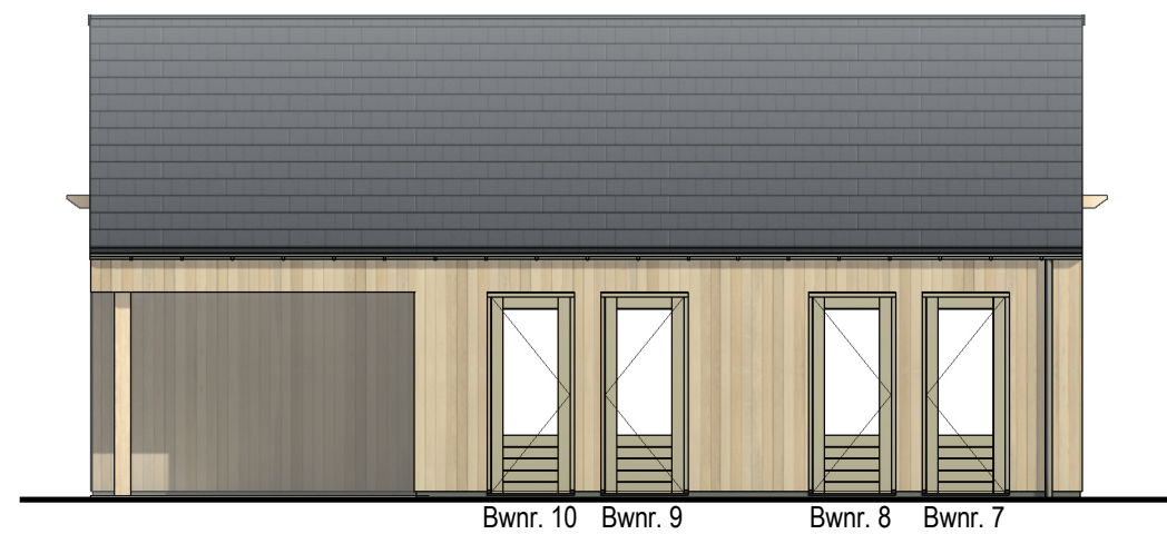
Voorgevel Bergingblok
