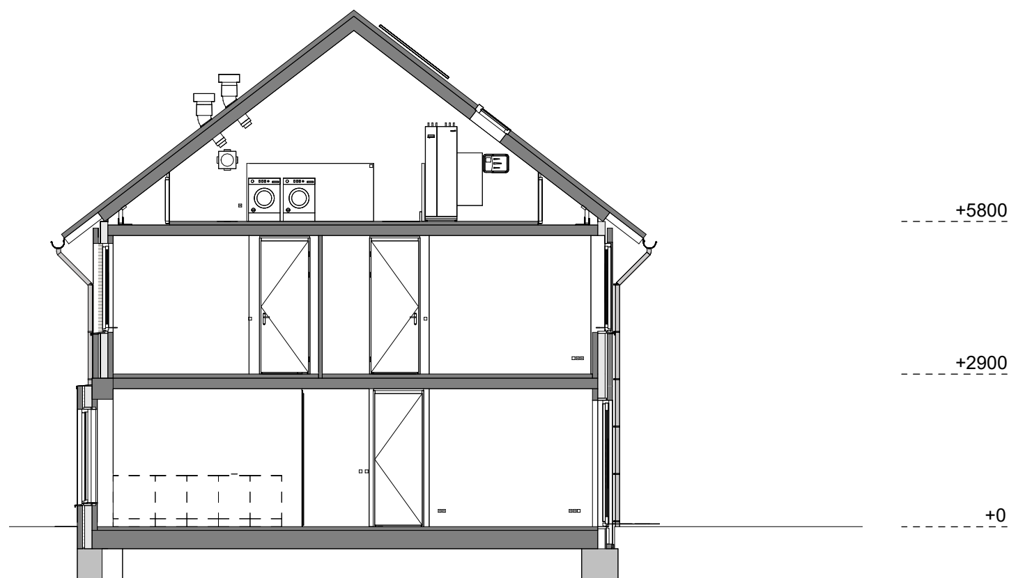
Doorsnede
