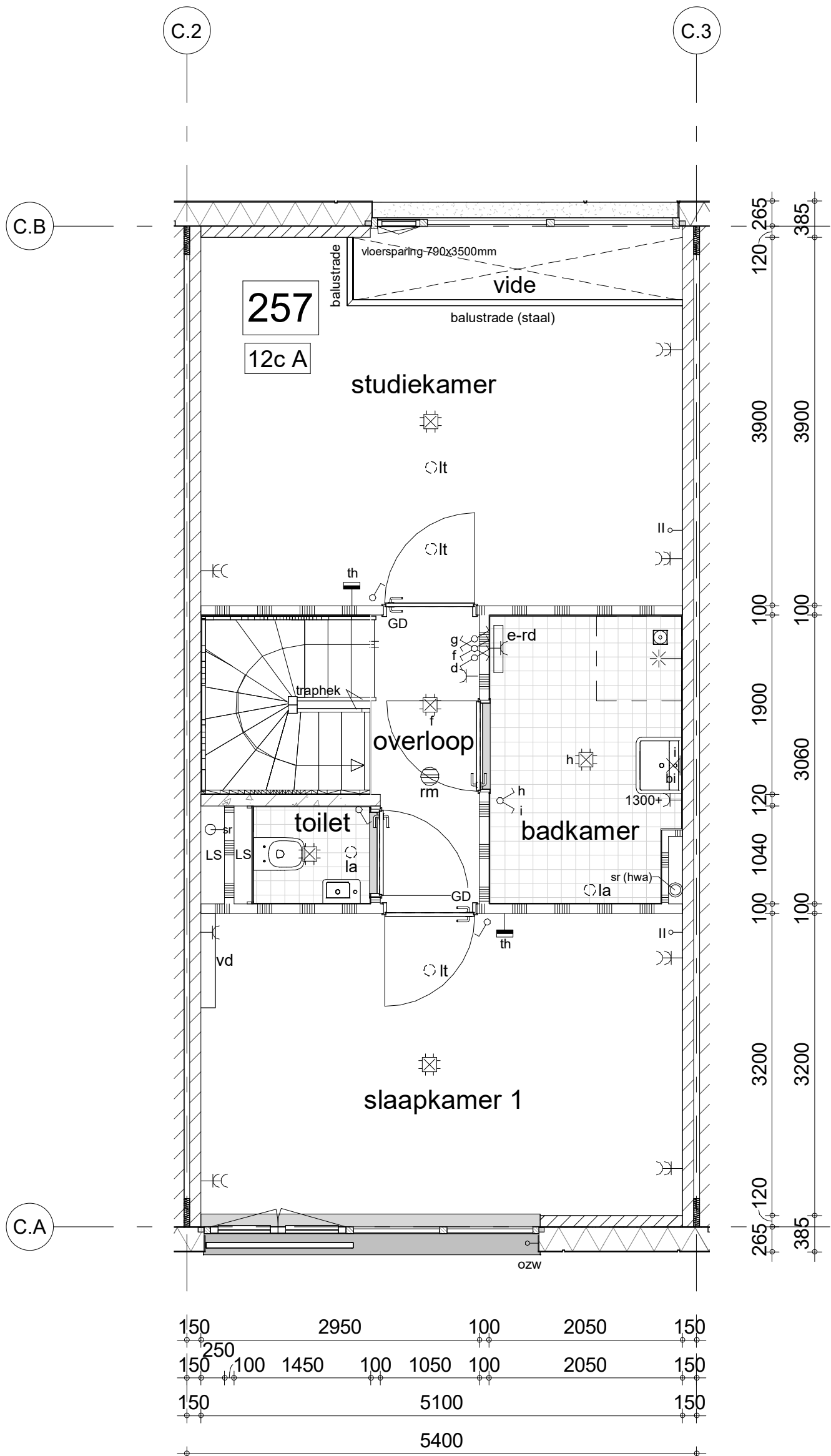
eerste verdieping
