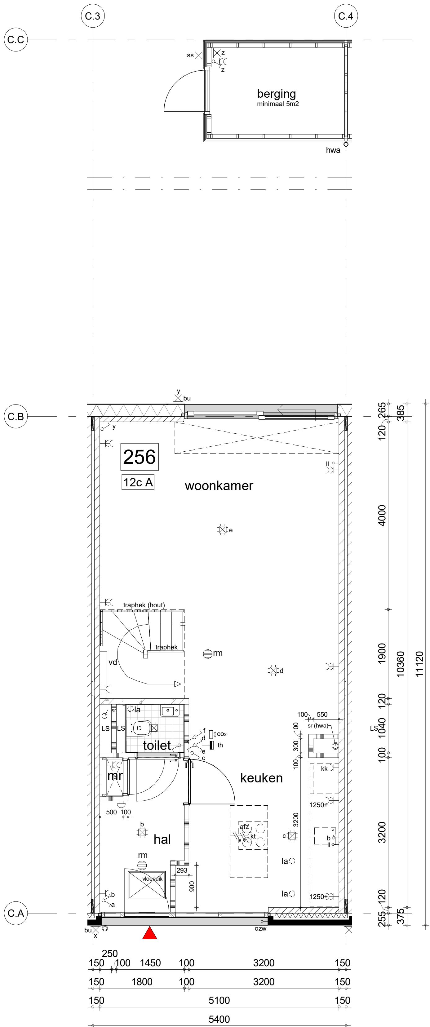
begane grond
