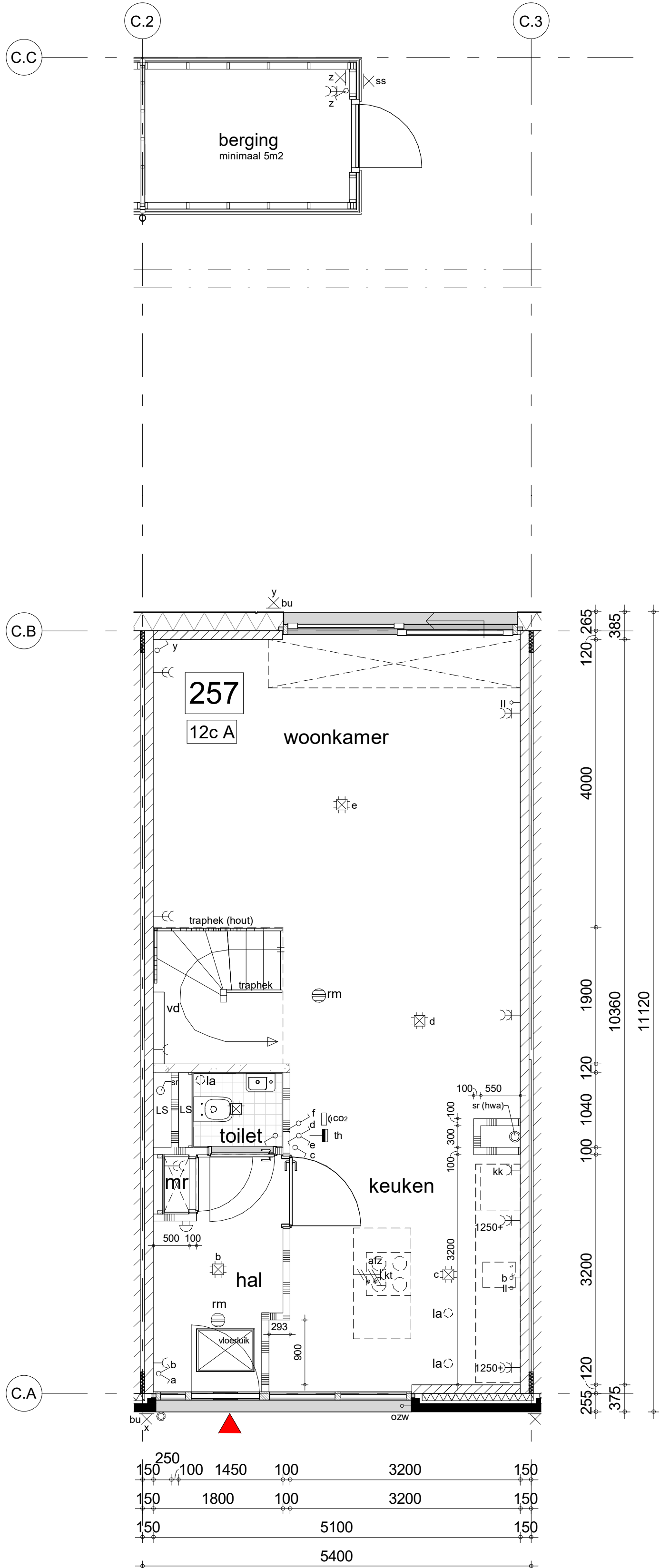
begane grond
