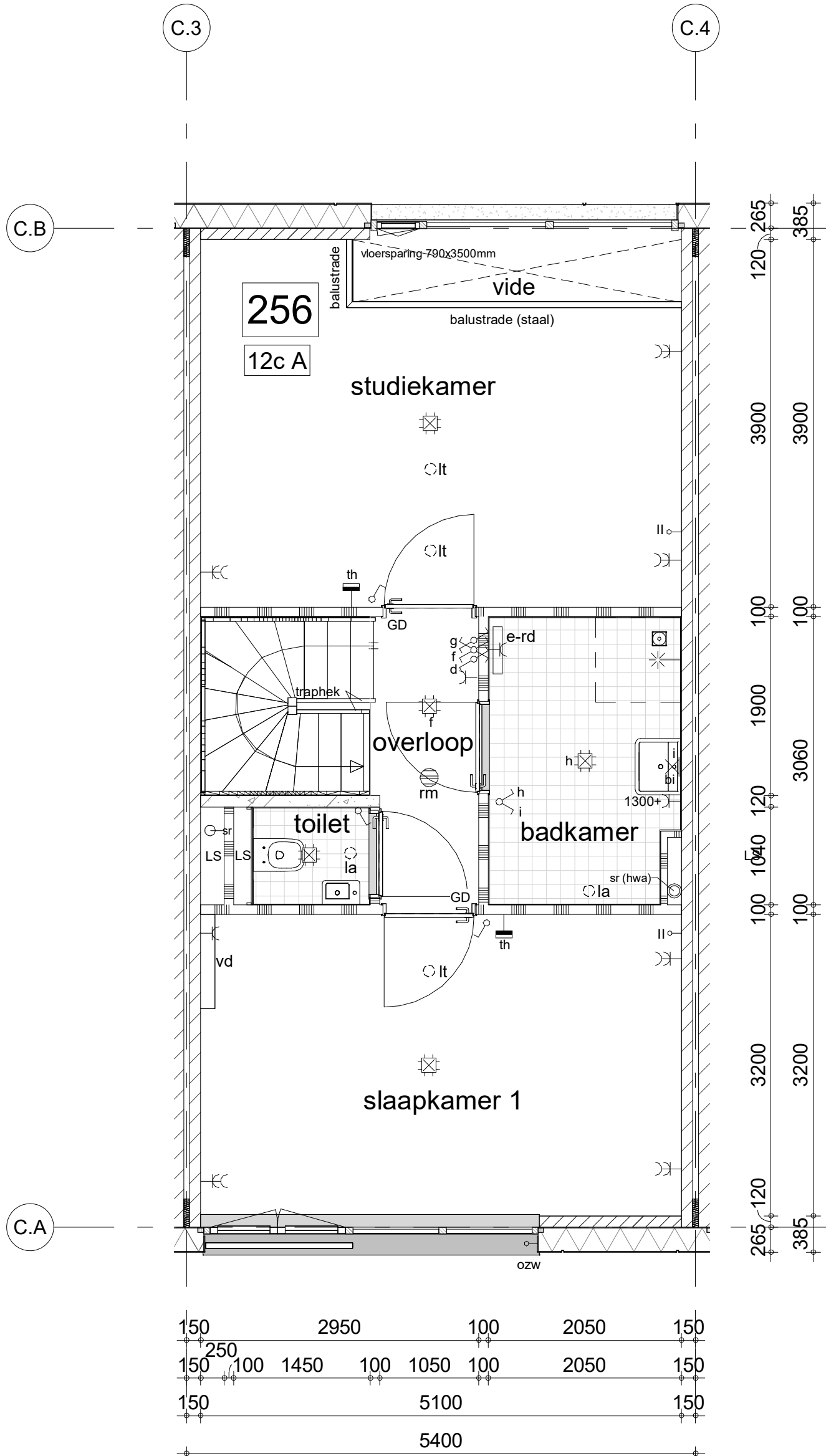
eerste verdieping
