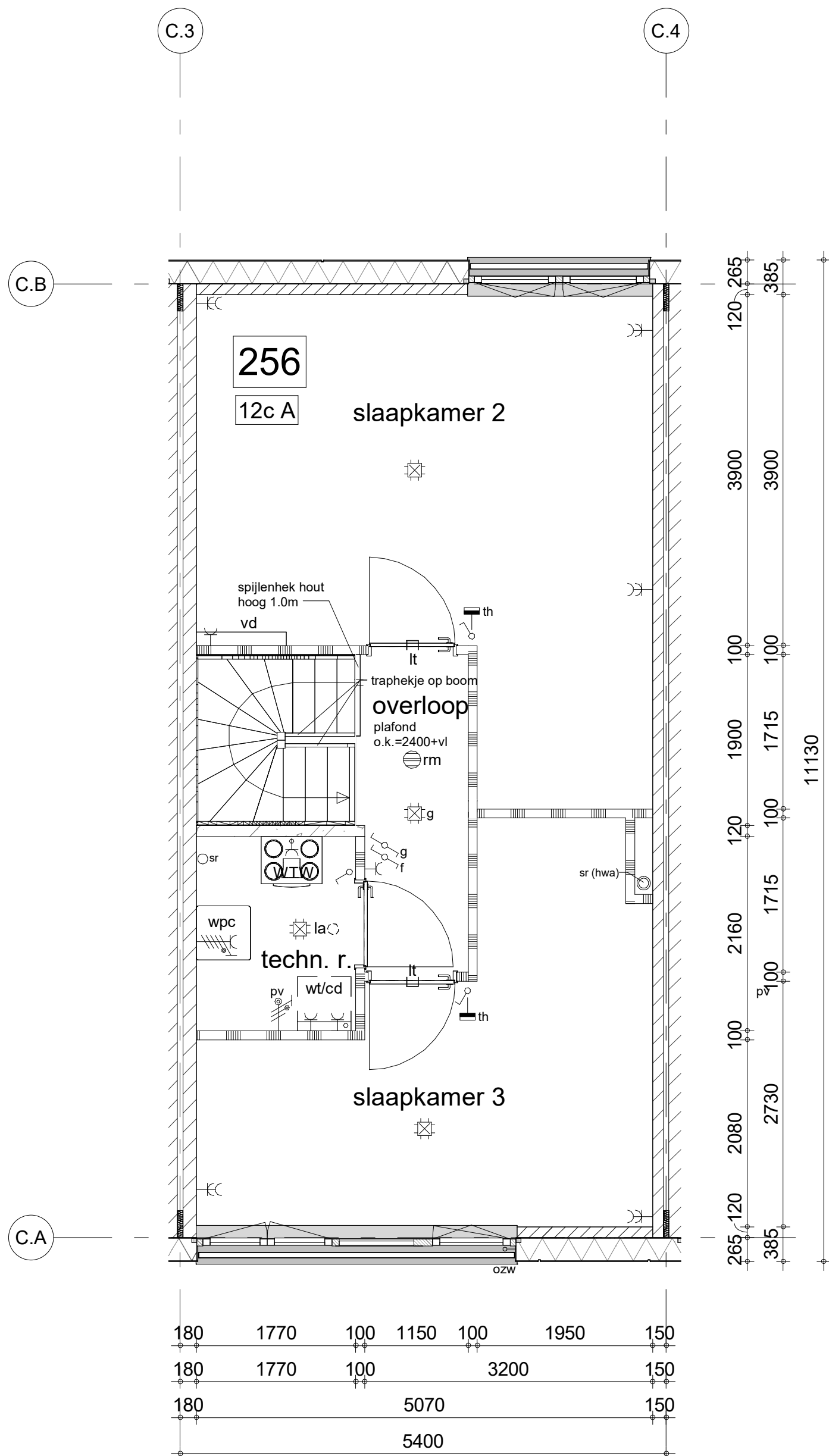
tweede verdieping
