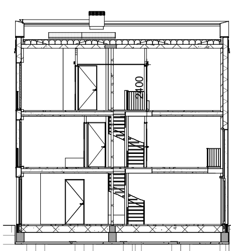
Doorsnede
