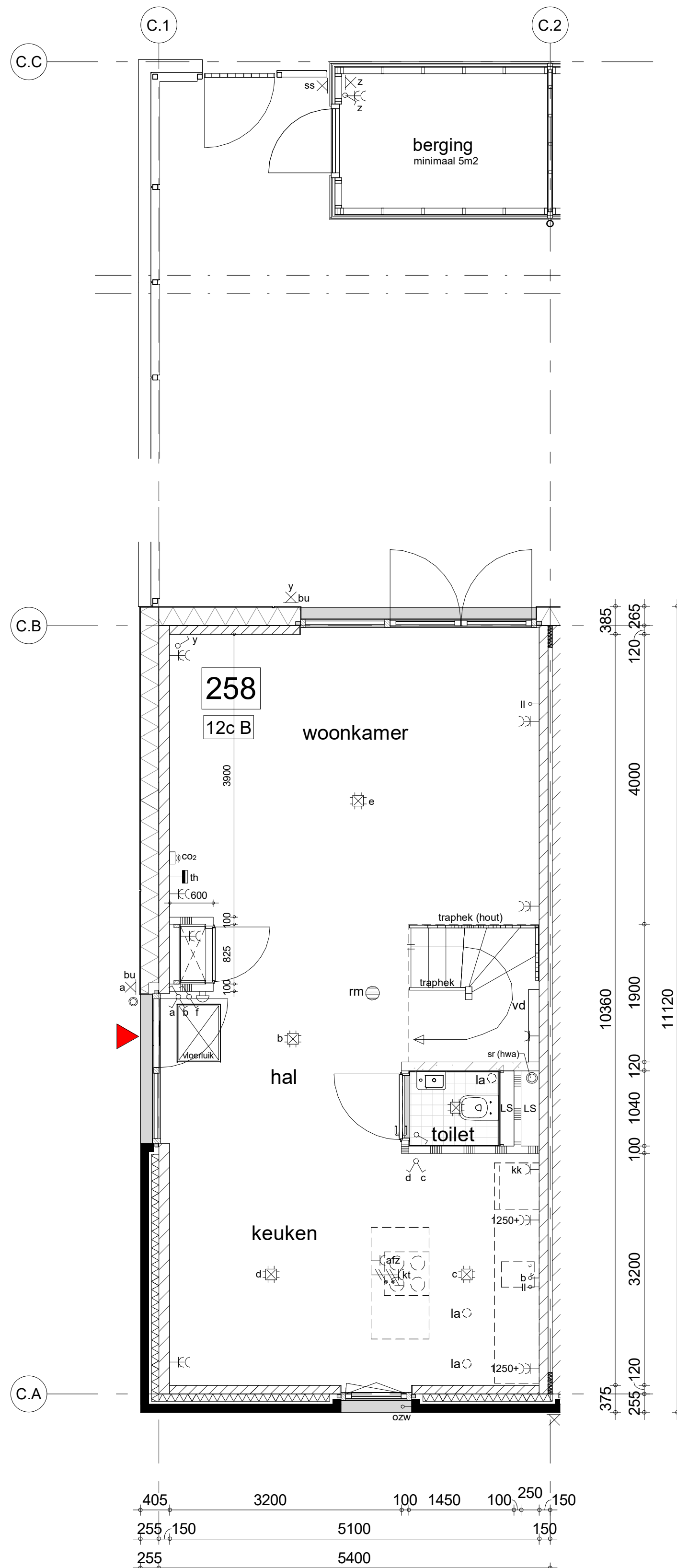
begane grond
