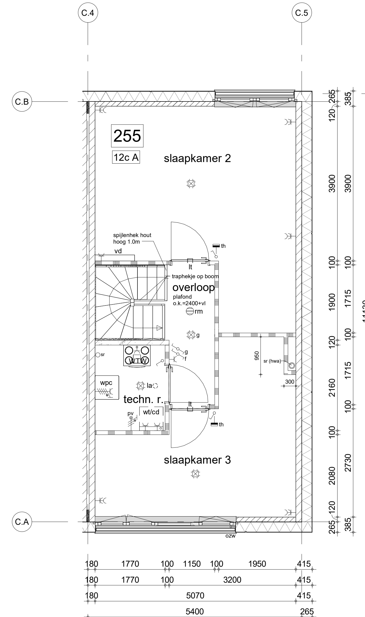
tweede verdieping
