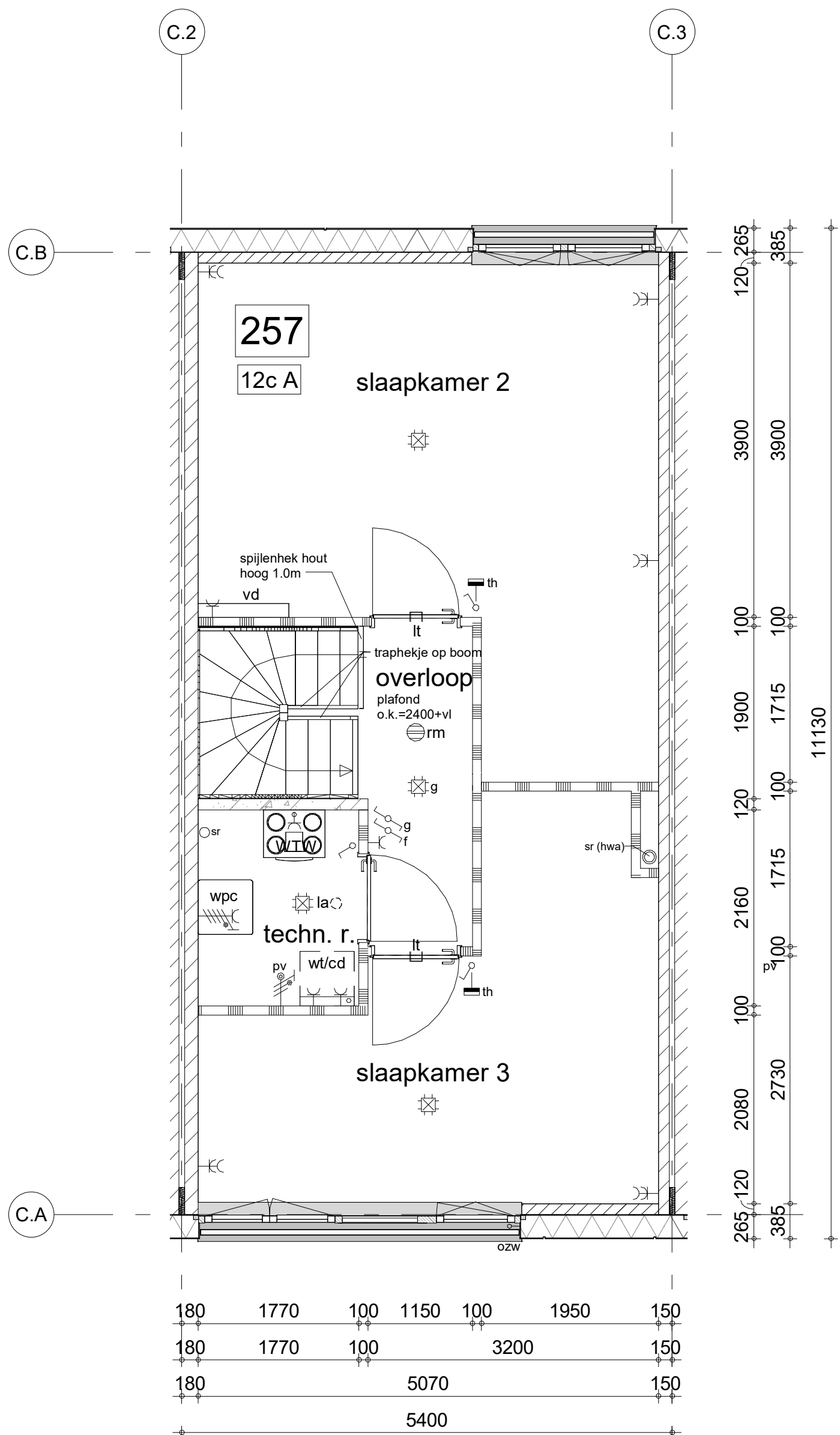
tweede verdieping
