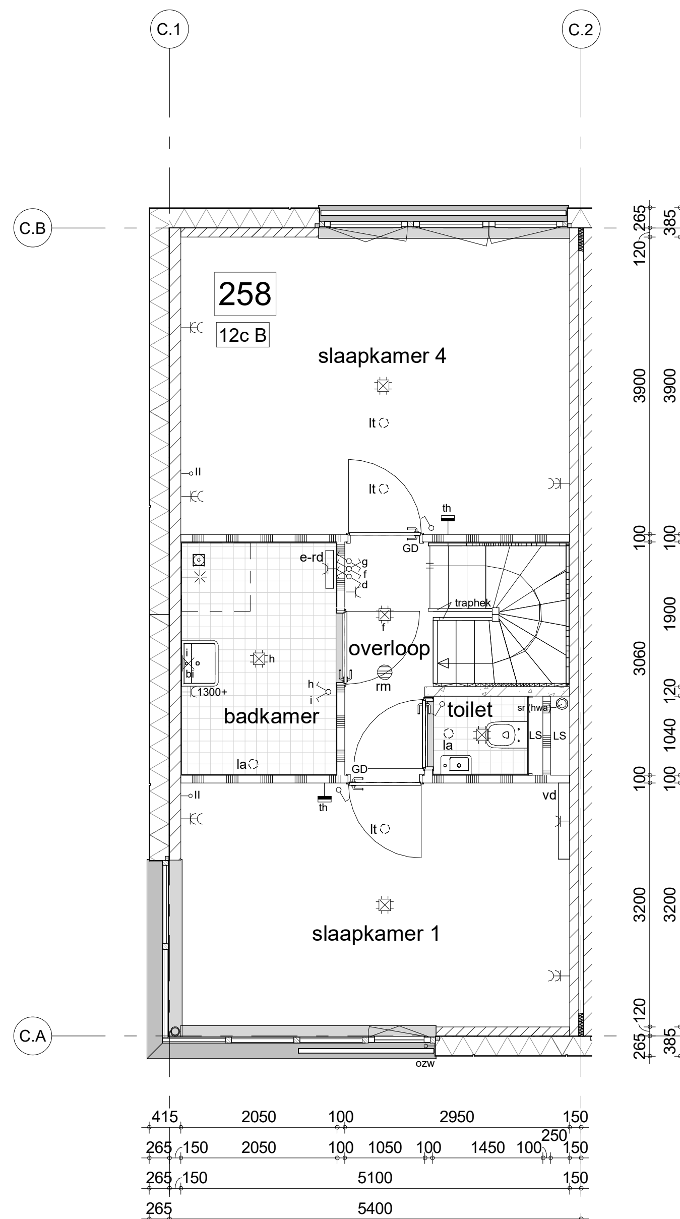
eerste verdieping
