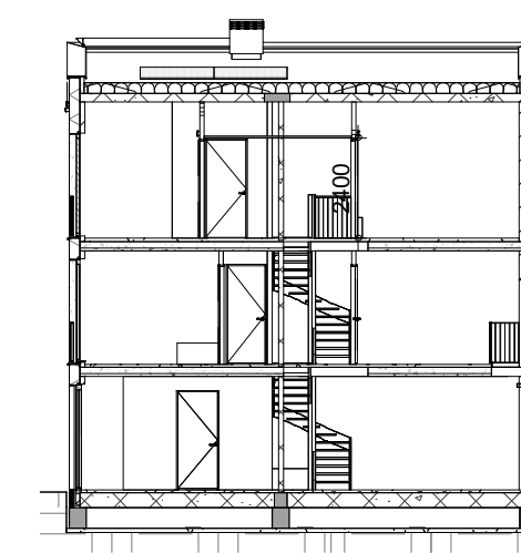
Doorsnede
