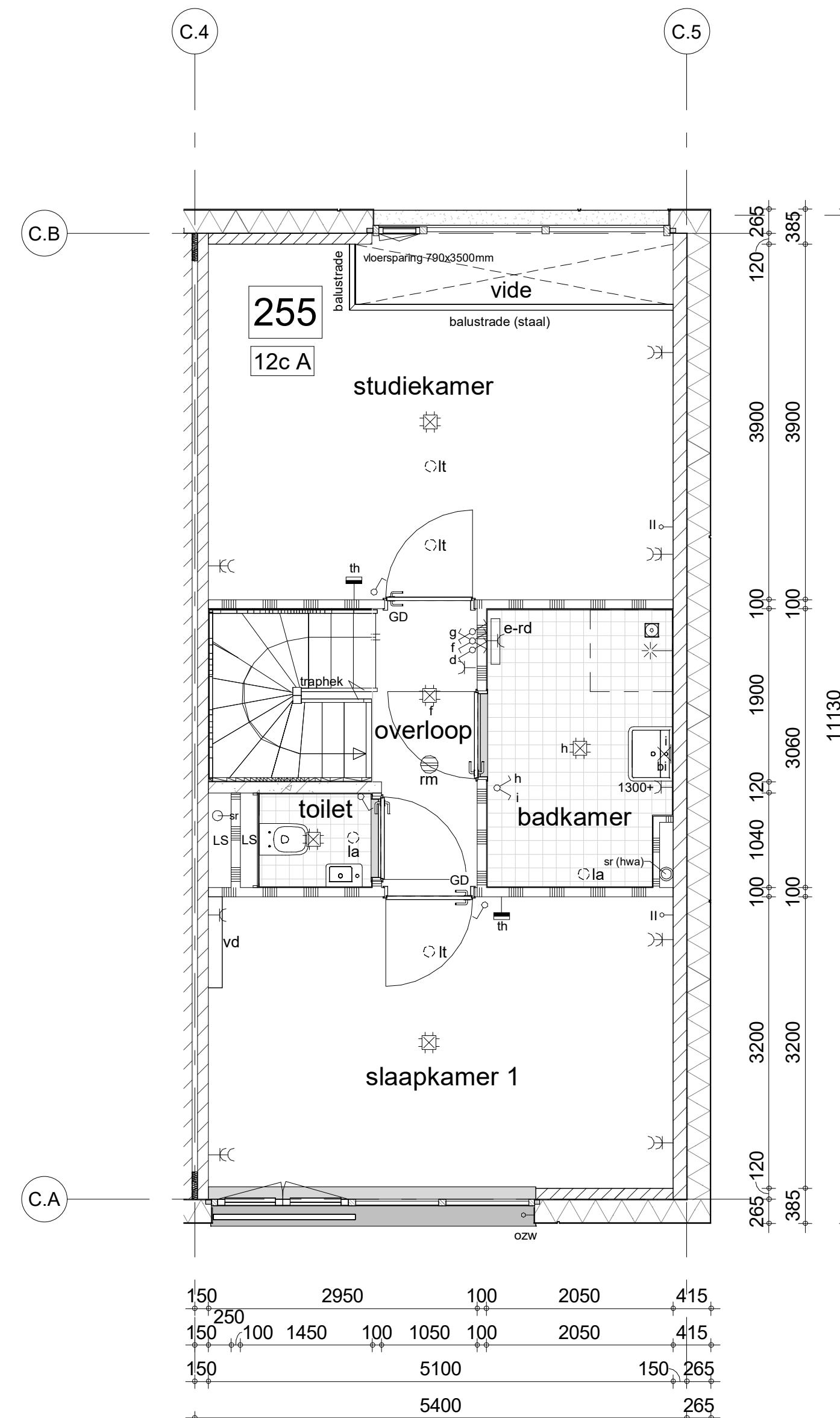
eerste verdieping
