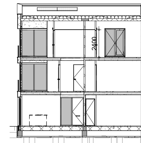
Doorsnede
