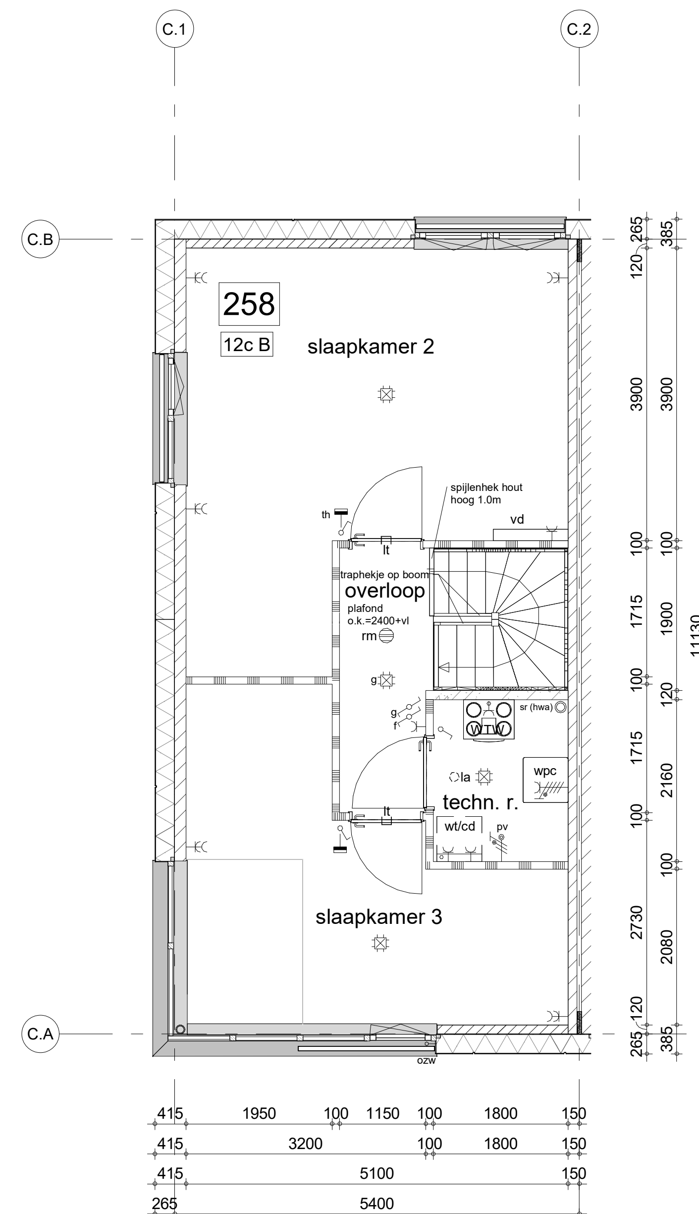
tweede verdieping
