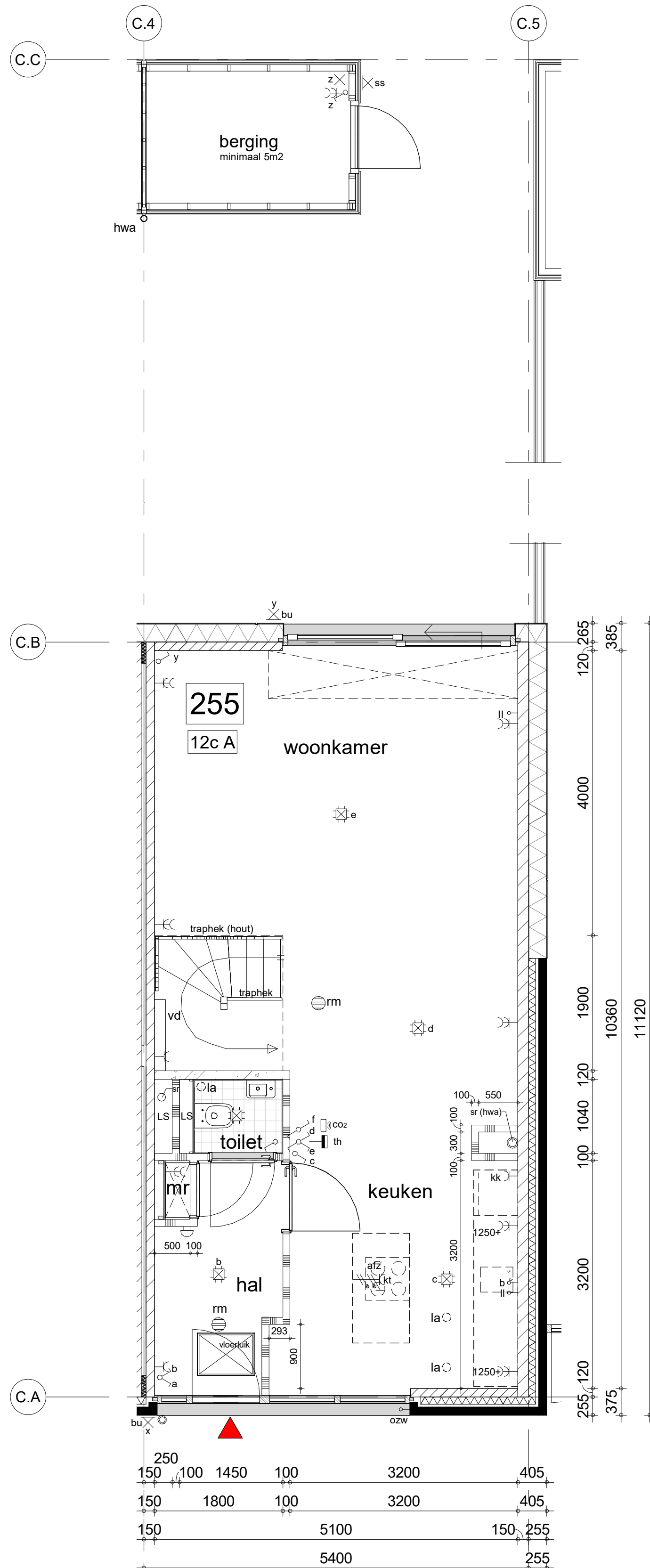
begane grond
