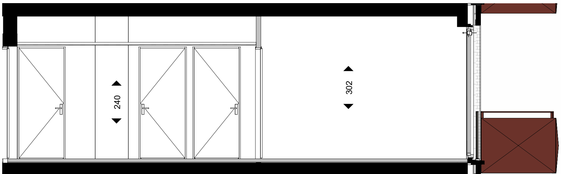
Lengtedoorsnede 1:50
