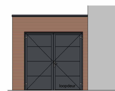
Voorgevel schaal 1:100
