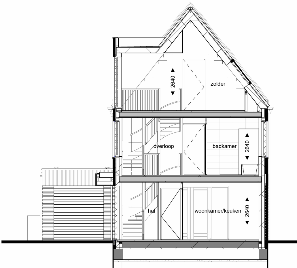
Doorsnede B-B
