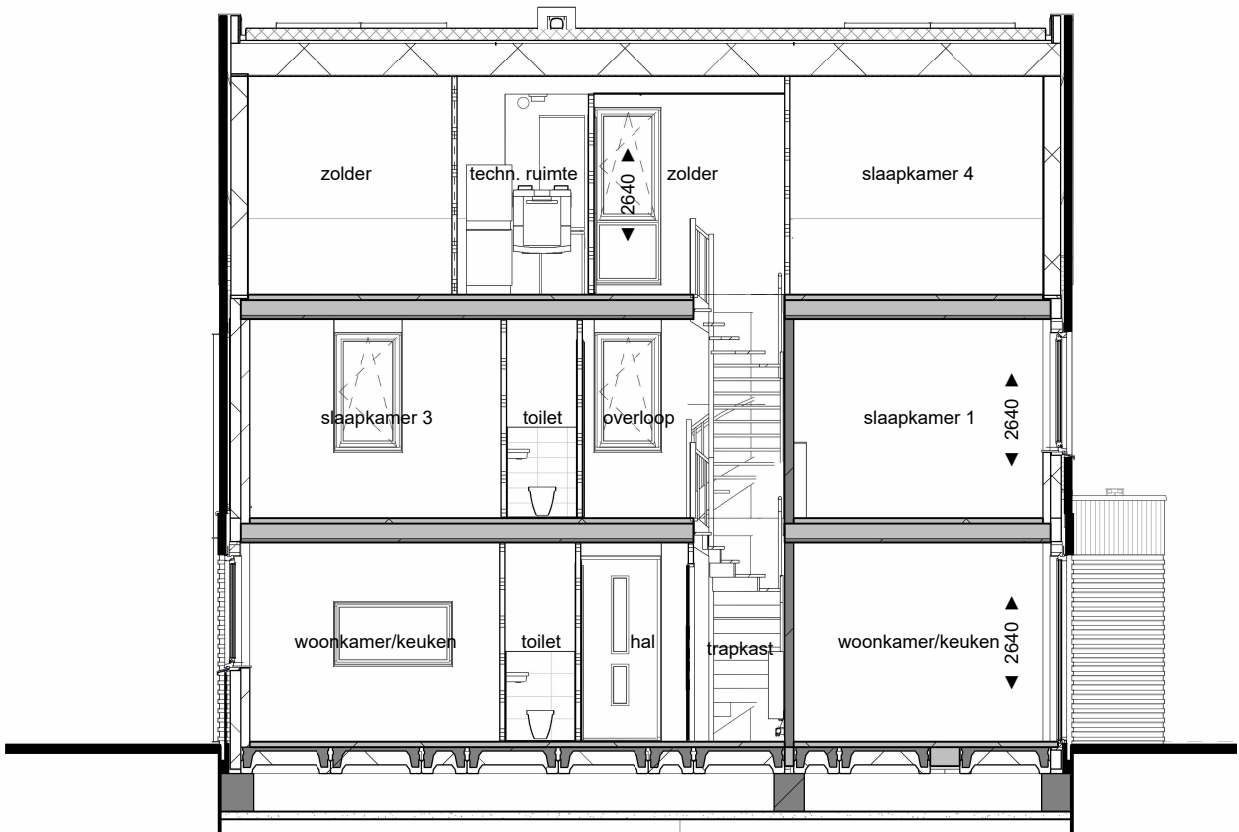
Doorsnede A-A
