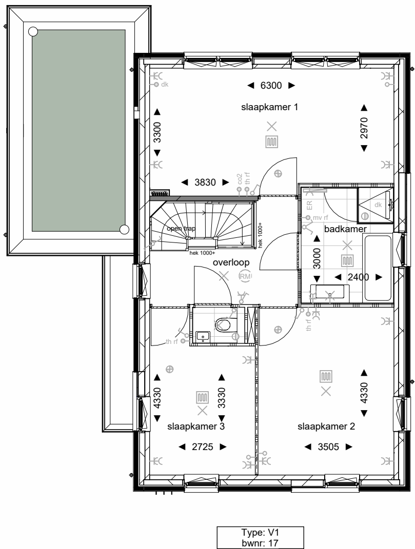
Eerste verdieping
