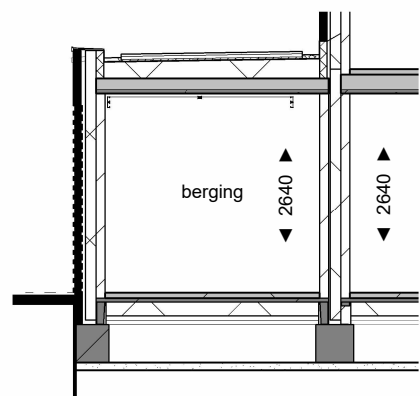
Doorsnede C-C
