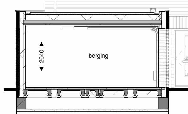
Doorsnede D-D
