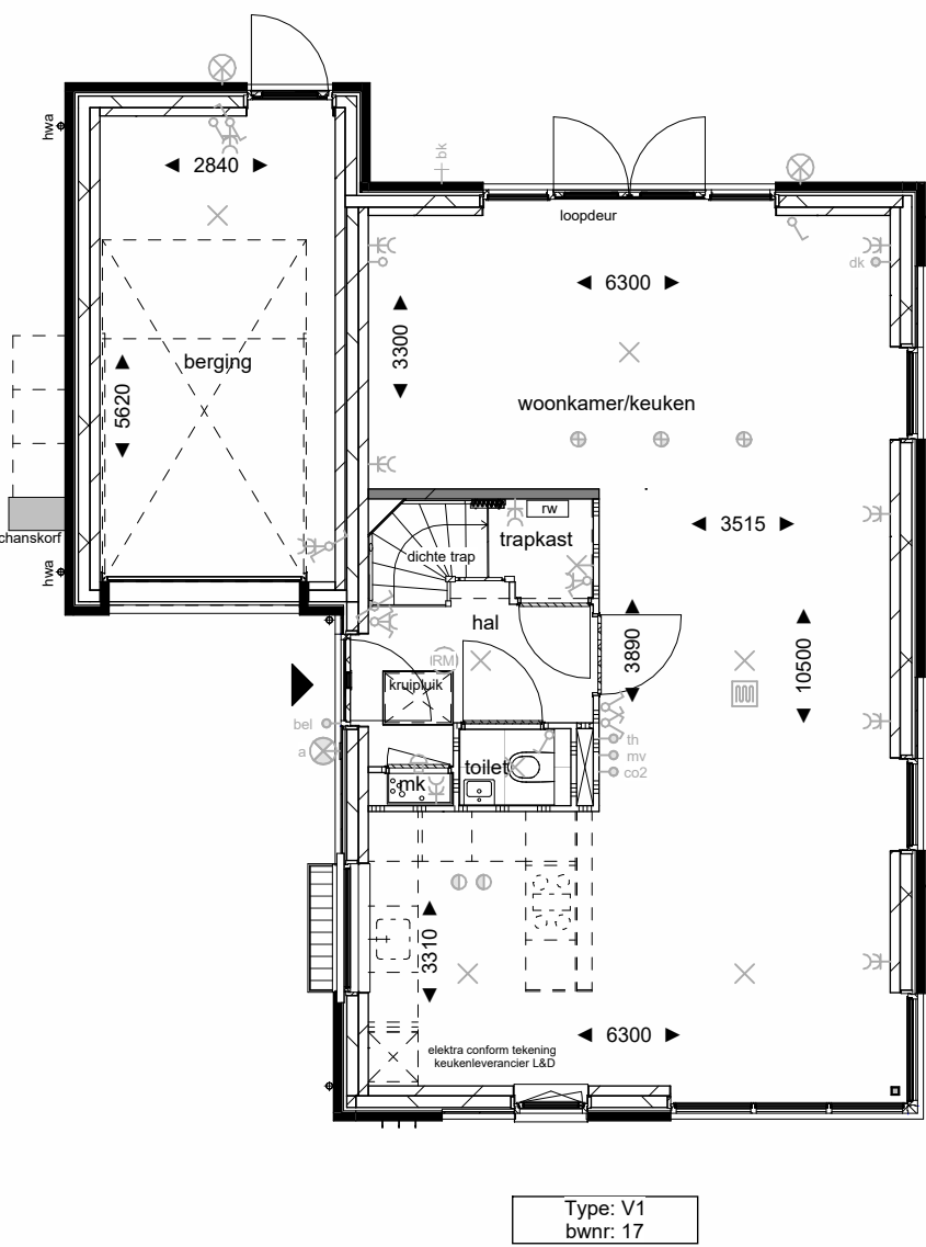
Begane grond
