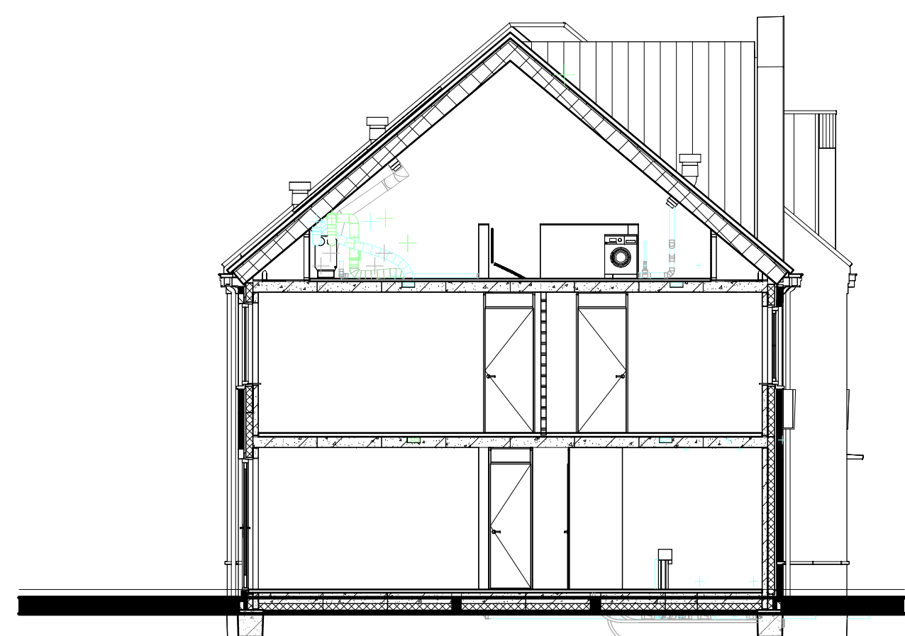
Doorsnede A1-A1
