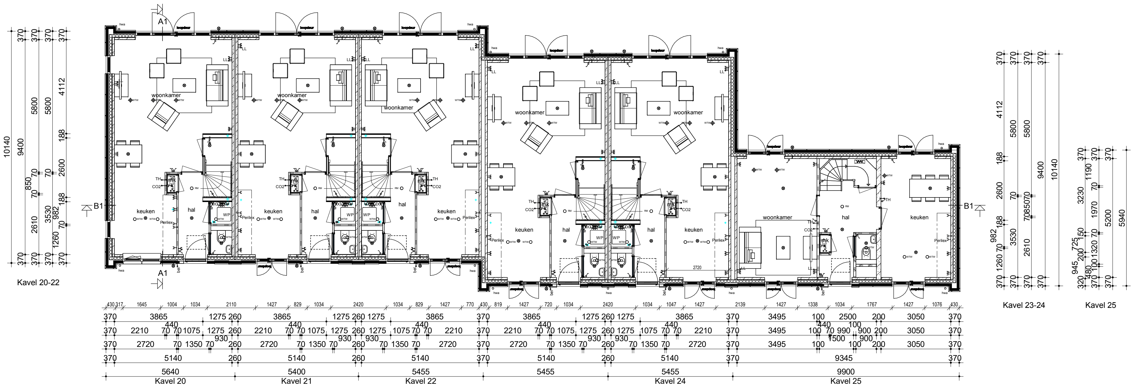
Begane grond
