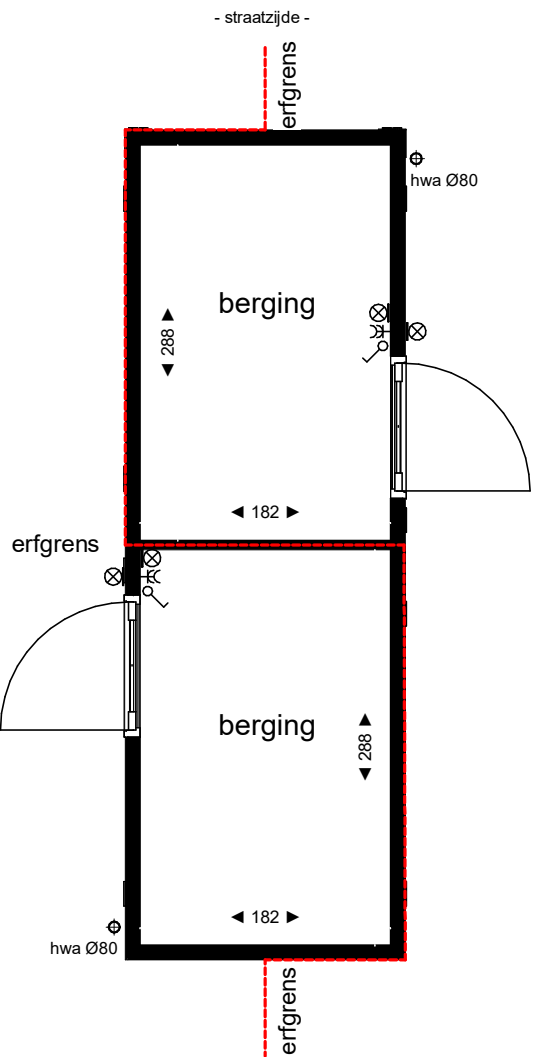
principe tekening - geschakeld korte zijde -
