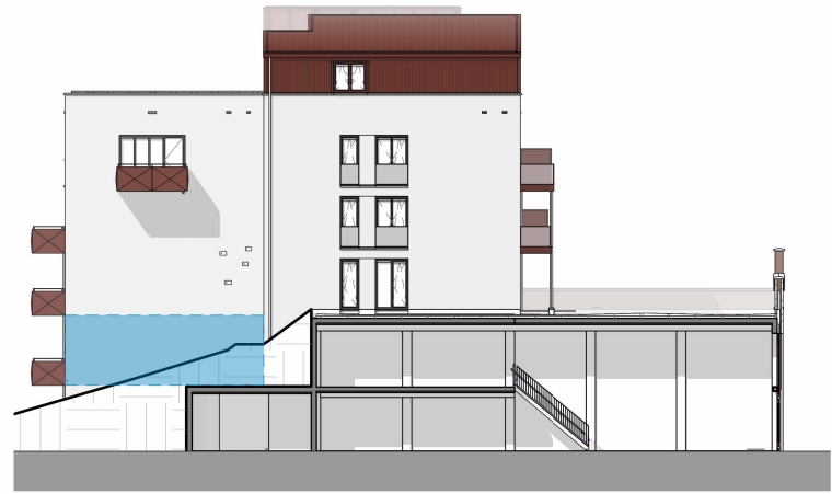
Zuidwestgevel 1:400
