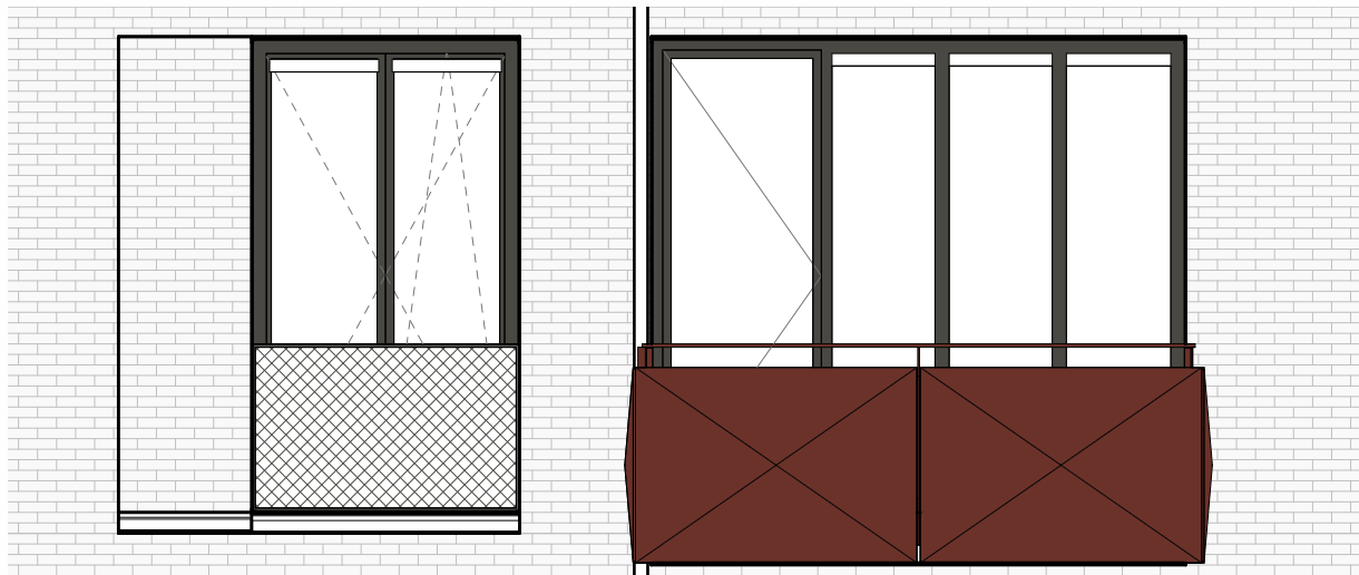
Gevelfragment Noordwestgevel 1:50
