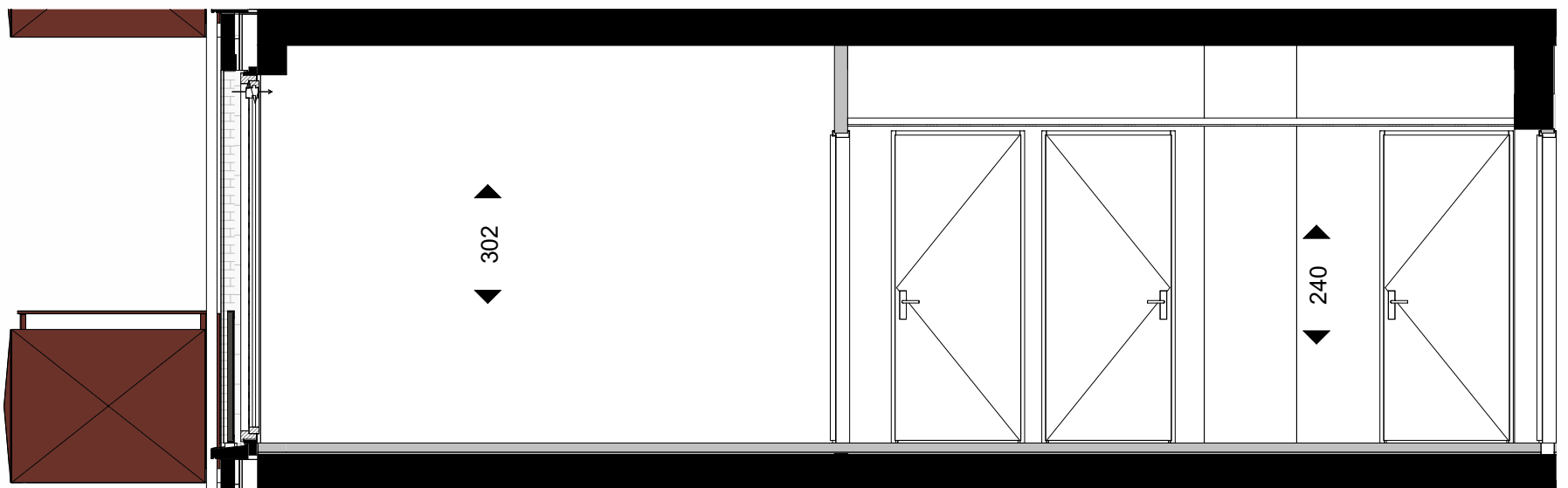
Lengtedoorsnede 1:50
