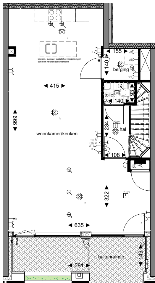
Begane grond
