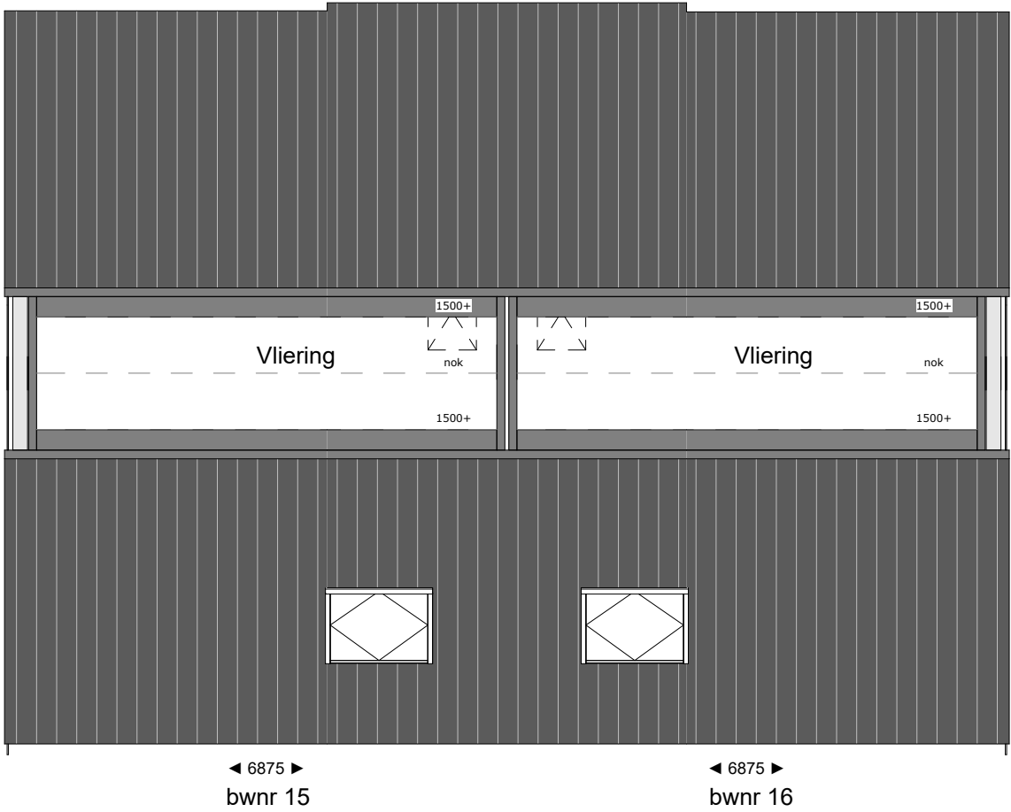
tweede verdieping
