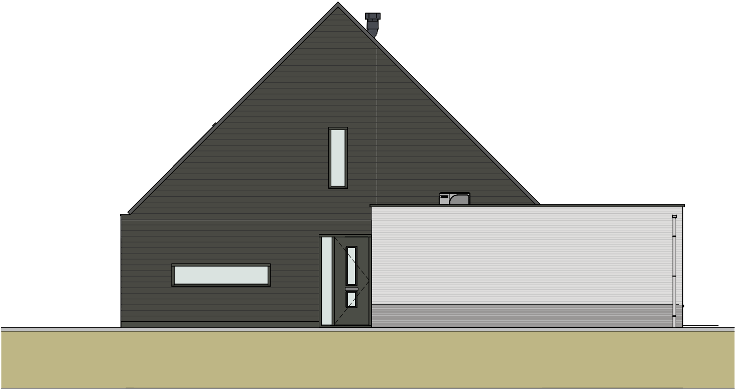
rechtergevel
