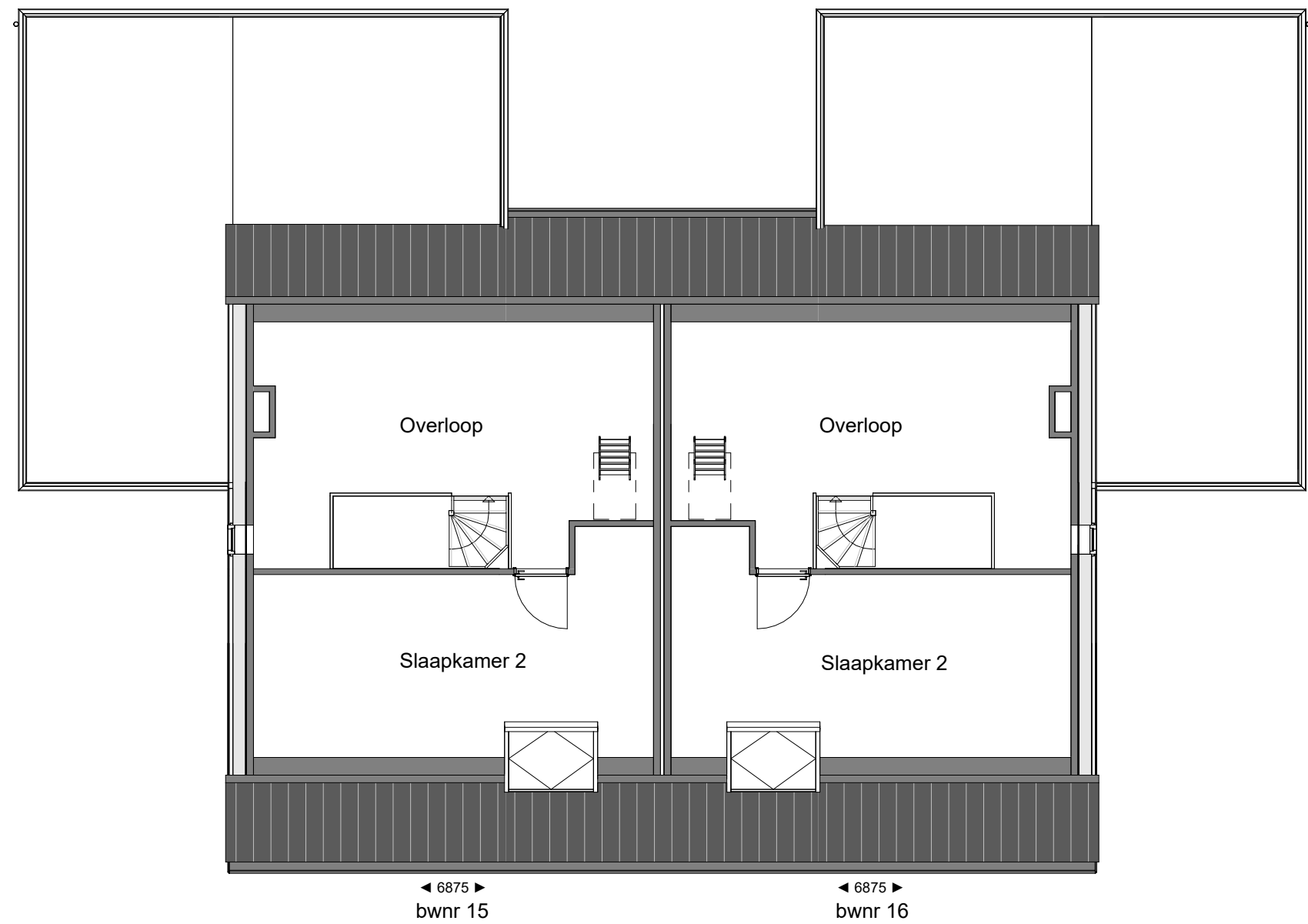
eerste verdieping
