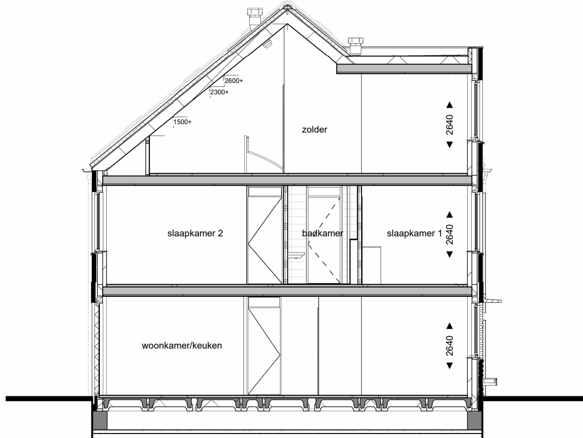
Doorsnede C-C
