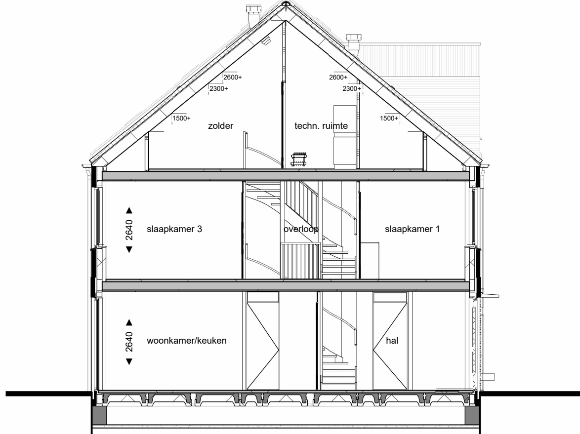
Doorsnede A-A
