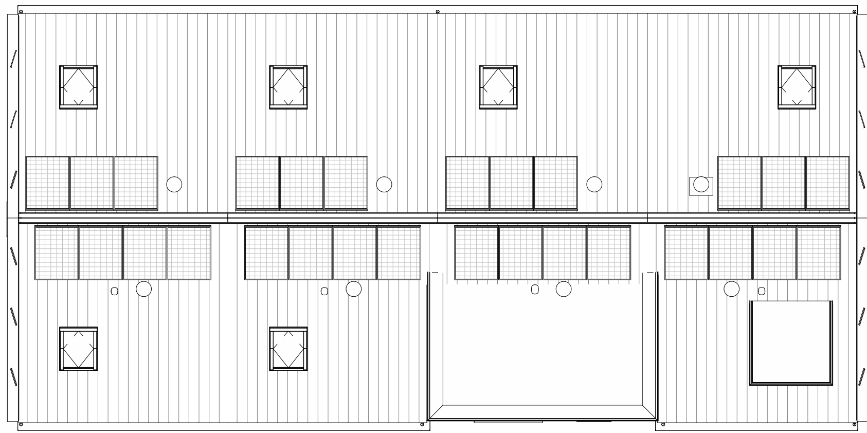
Dakaanzicht
