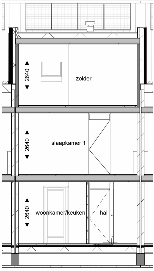
Doorsnede B-B
