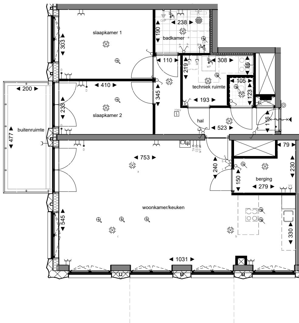
5e verdieping
