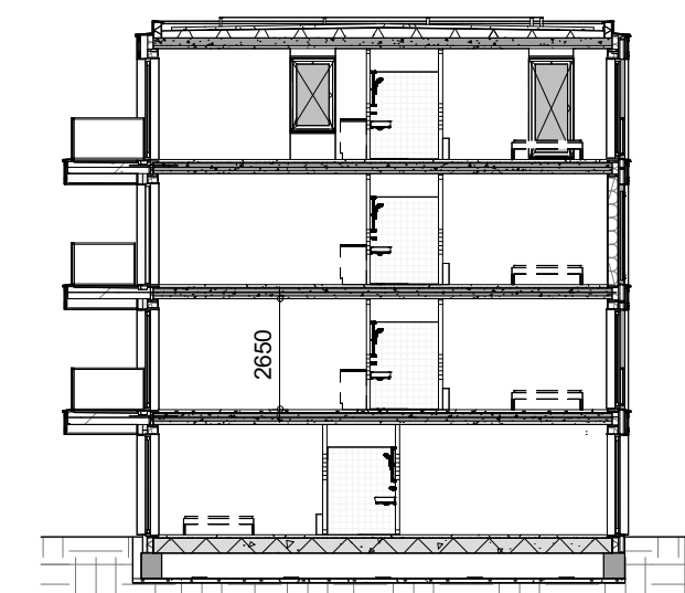
Doorsnede
