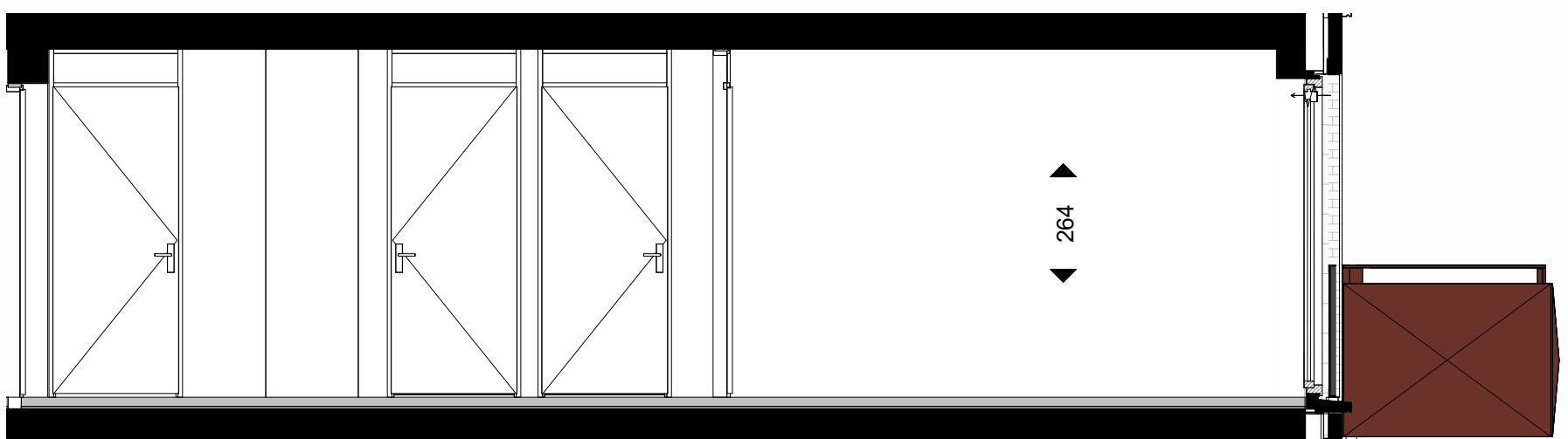
Lengtedoorsnede 1:50
