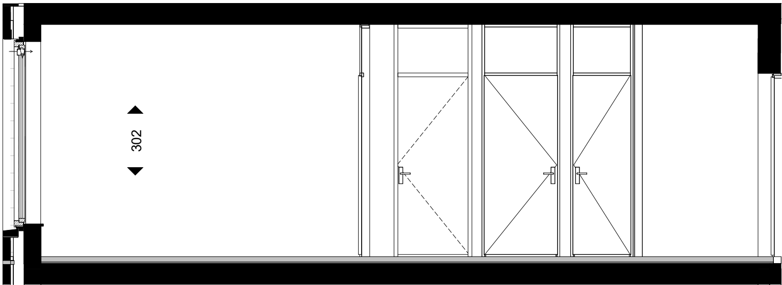
Lengtedoorsnede 1:50
