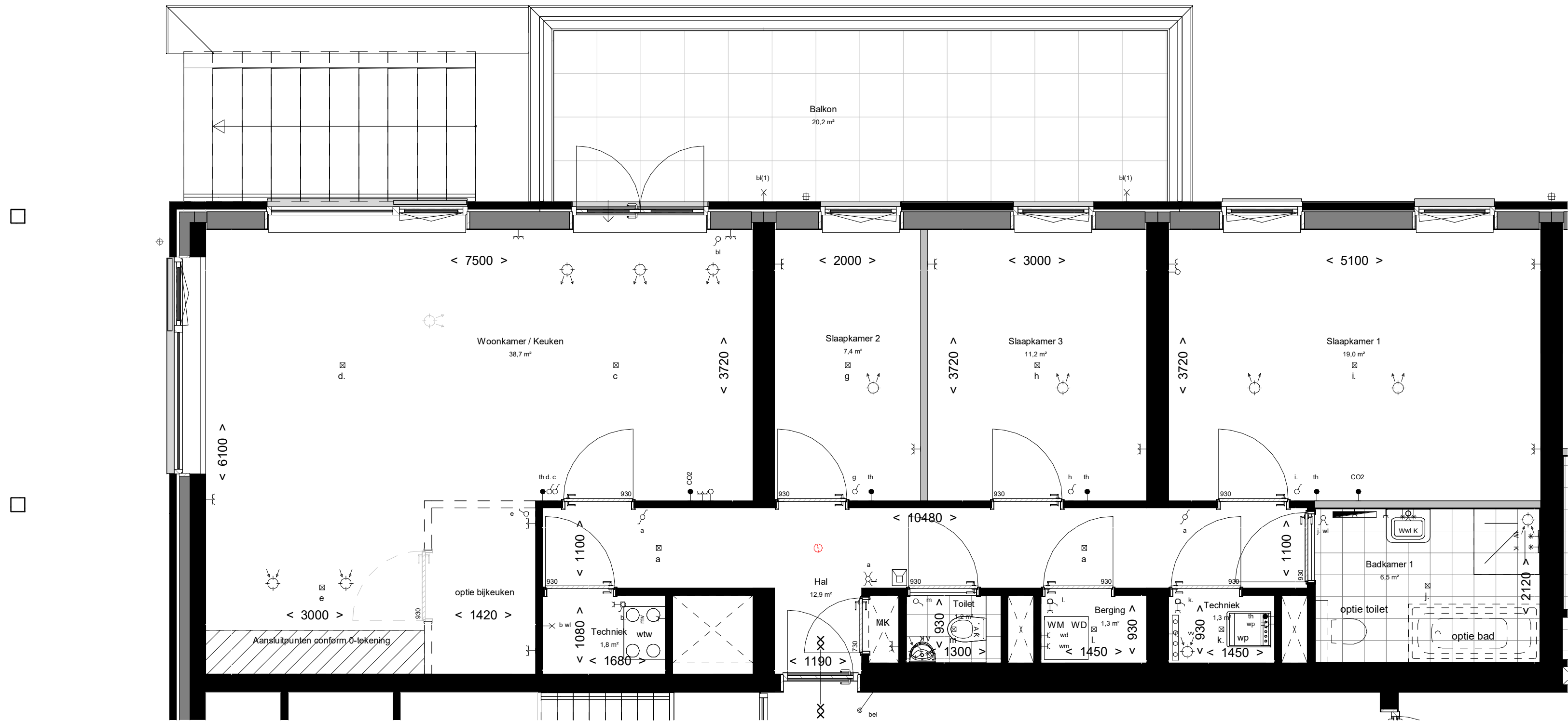
Begane grond BNR 75
