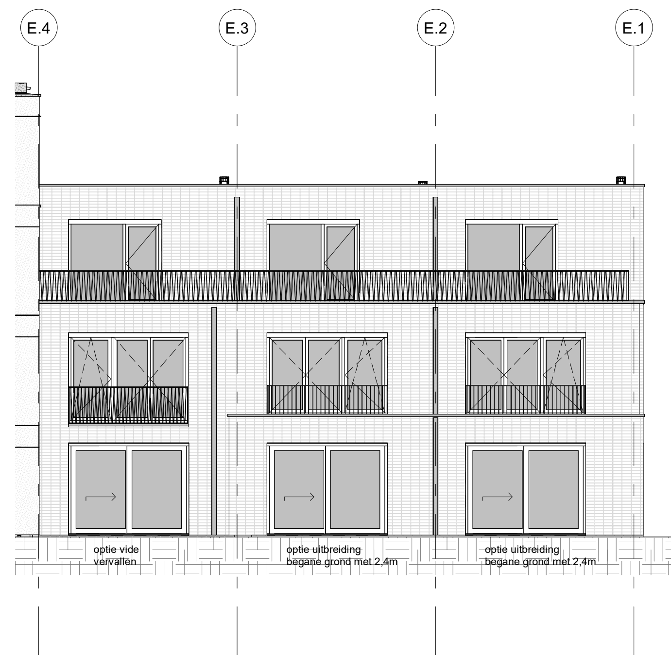
achtergevel blok 12e (Zuid-West) opties
