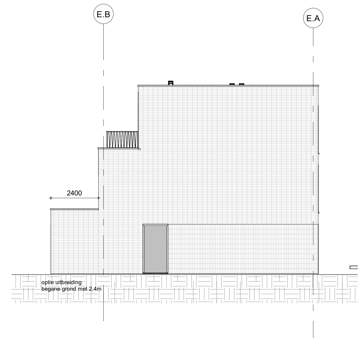
linker zijgevel blok 12e (Zuid-Oost) opties
