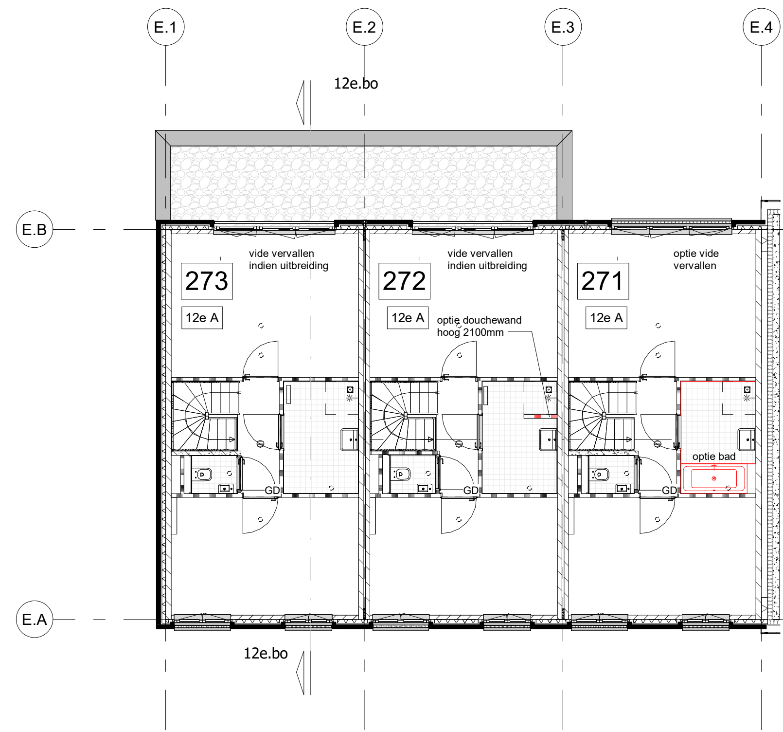
eerste verdieping blok 12e opties
