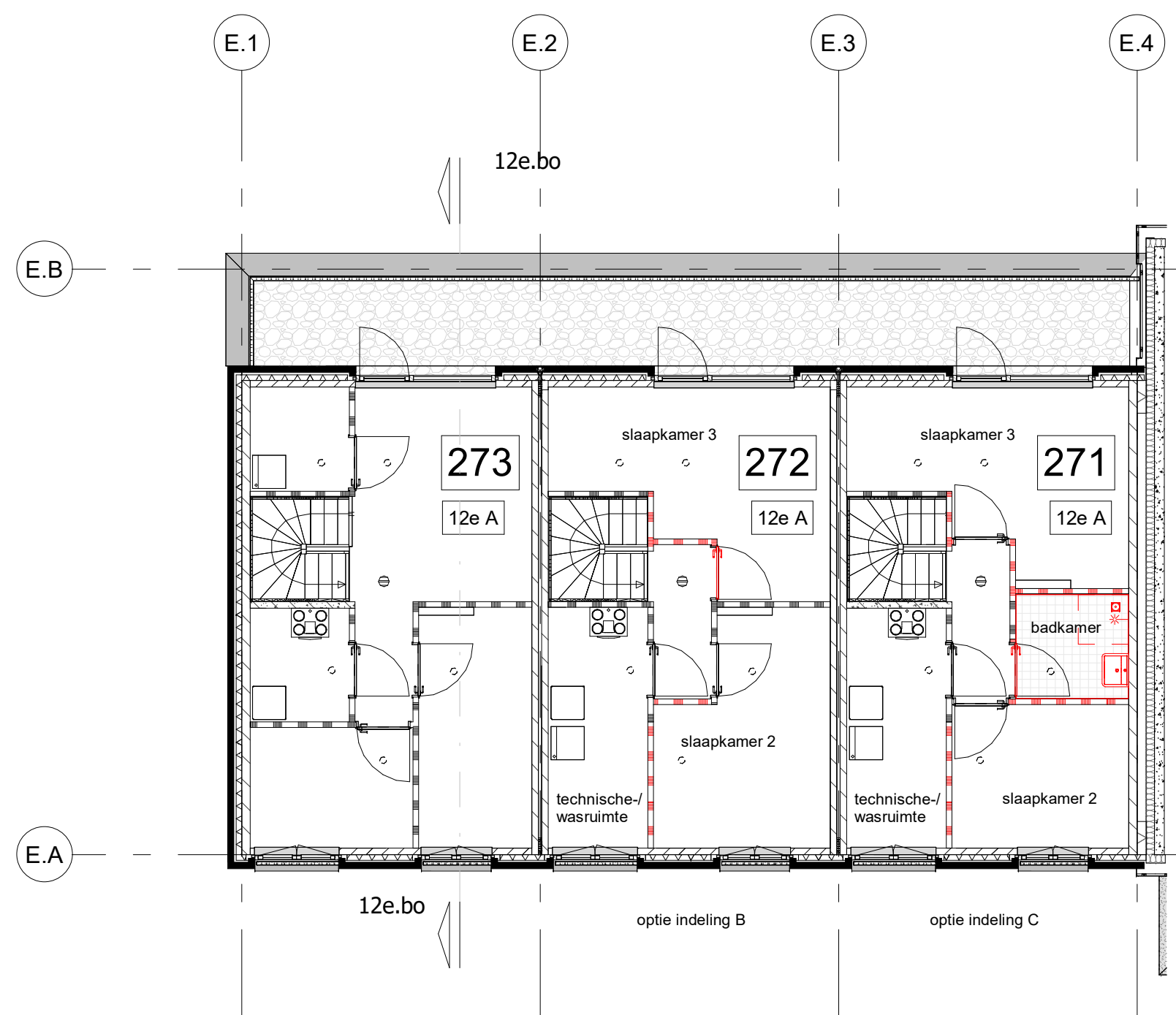
tweede verdieping blok 12e opties
