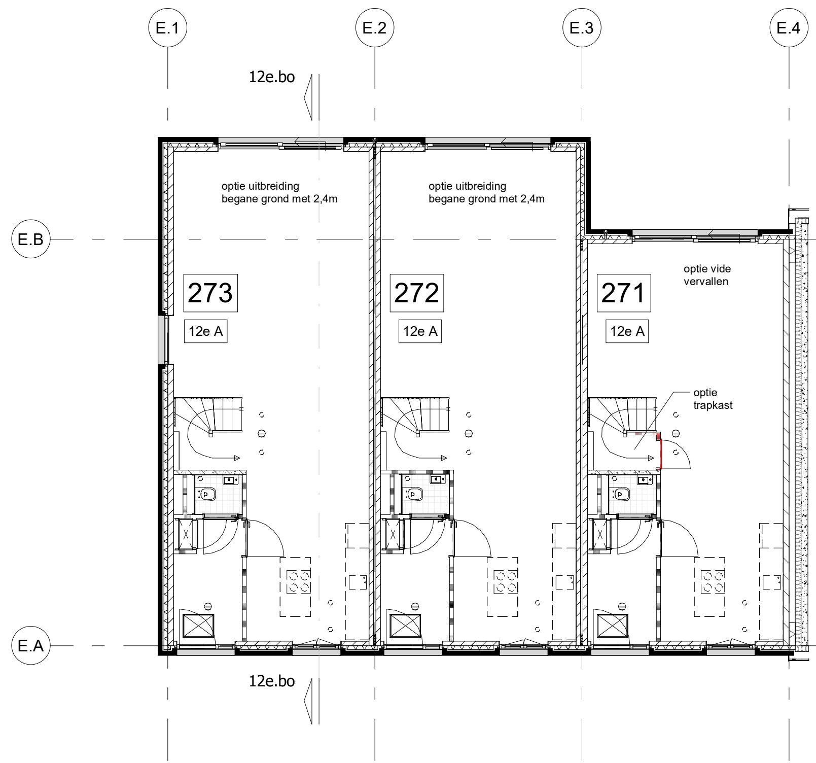
begane grond blok 12e opties
