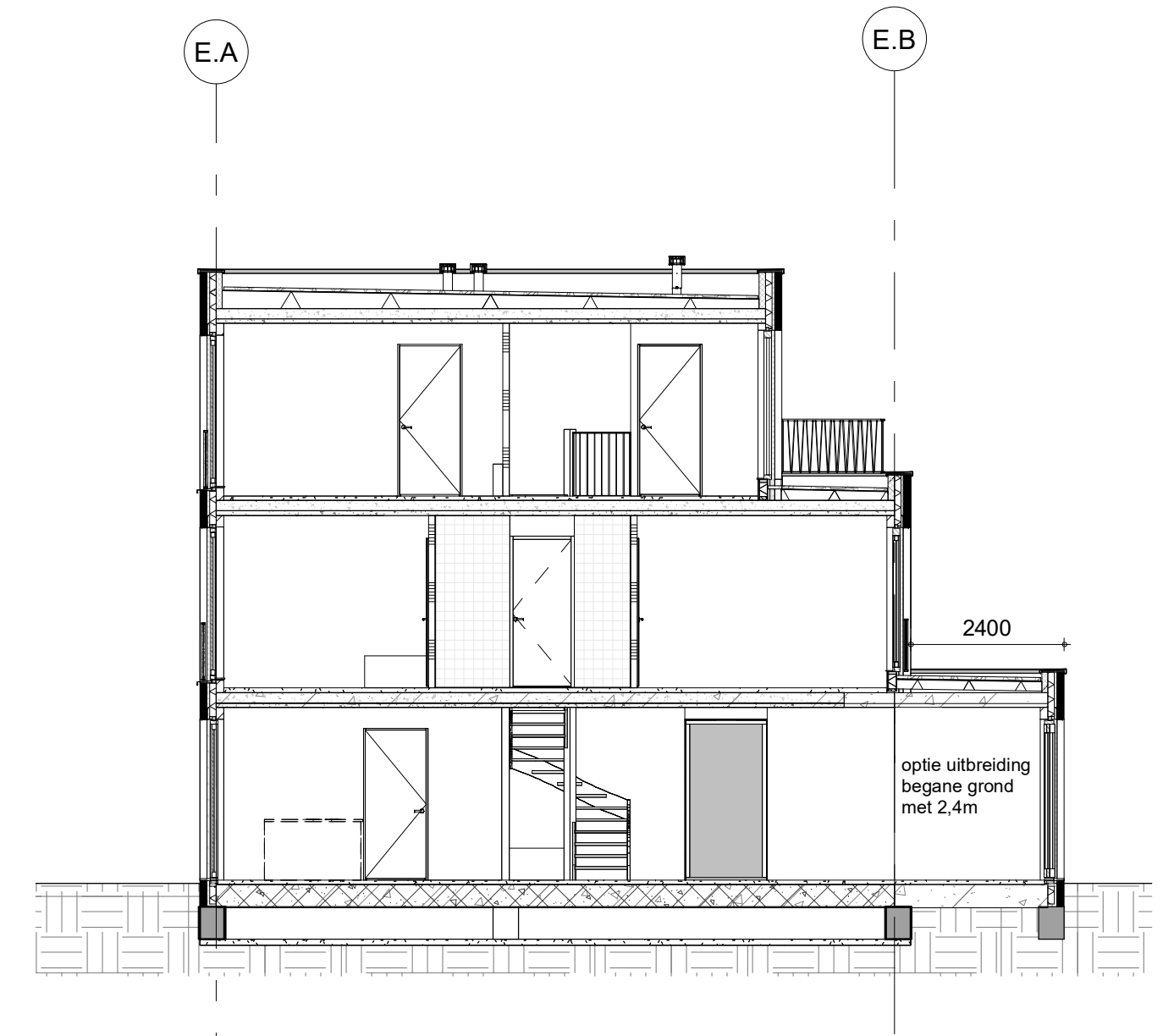
Doorsnede 12e.bo
