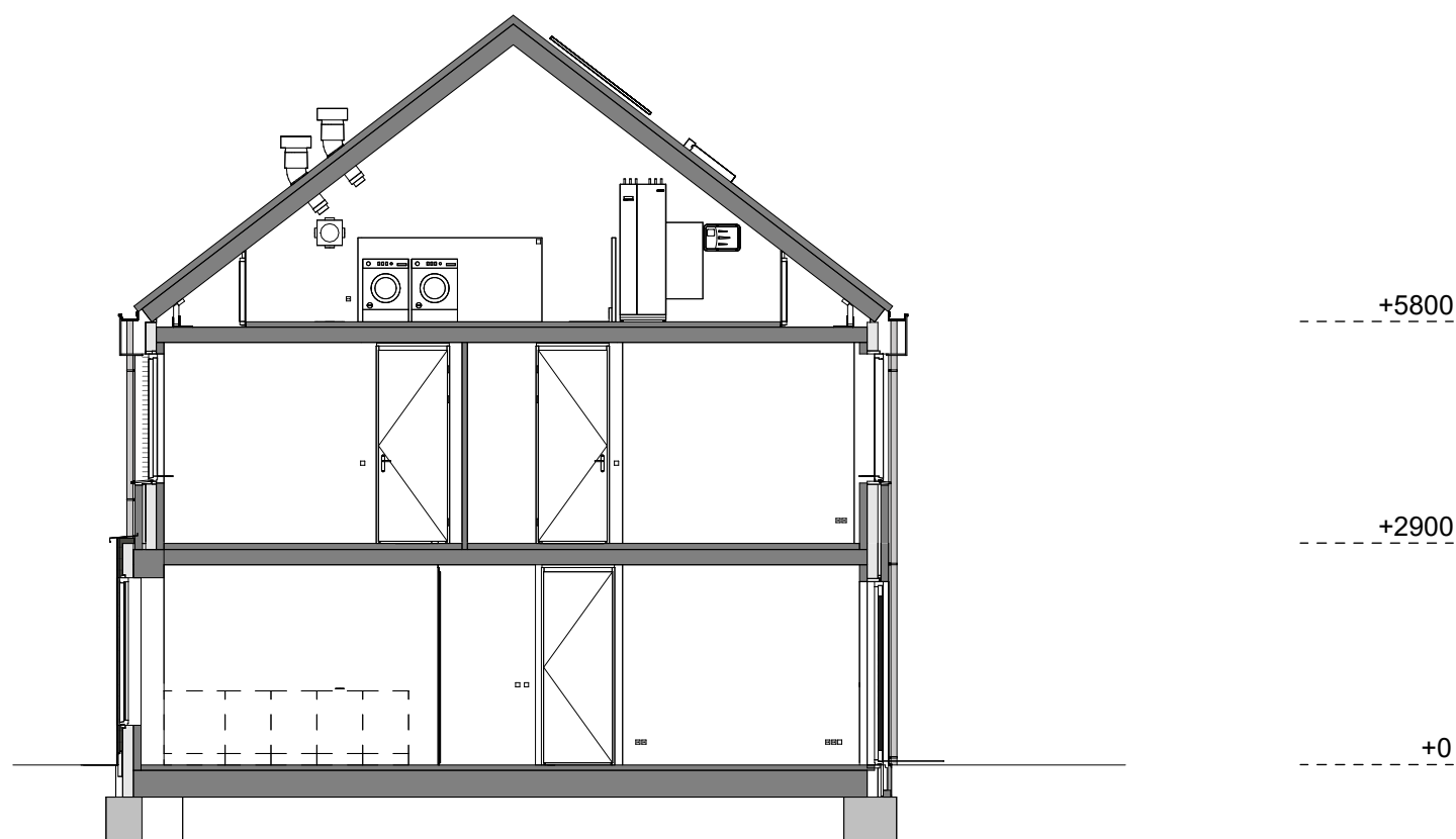
Doorsnede
