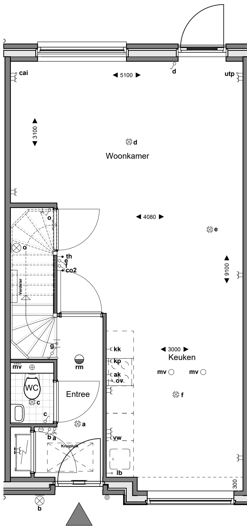
begane grond
