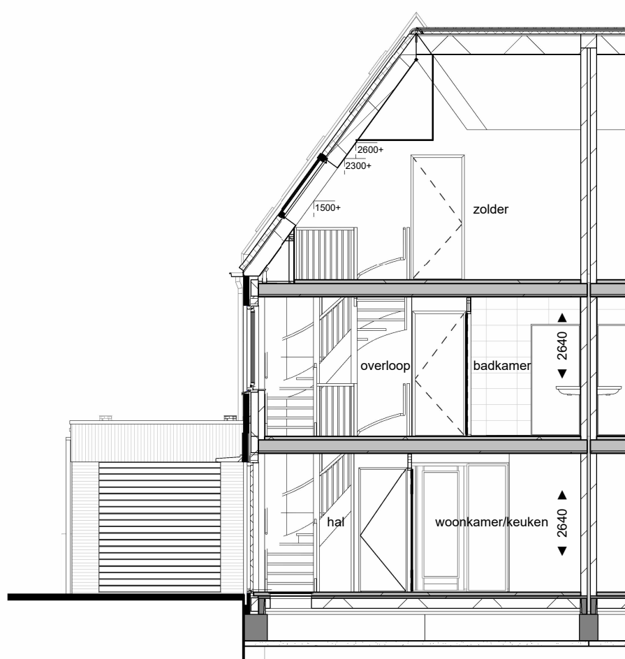
Doorsnede B-B
