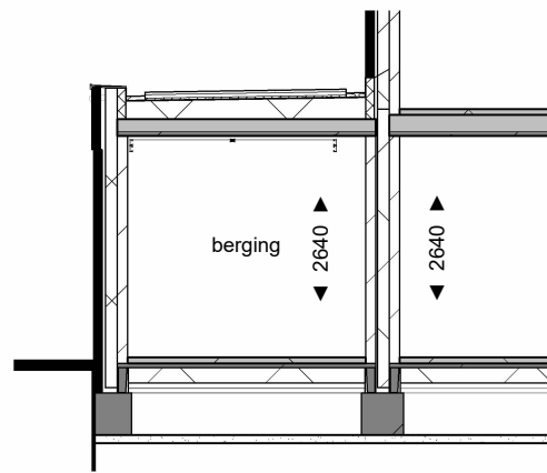
Doorsnede C-C
