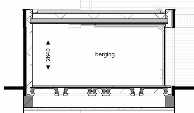
Doorsnede D-D
