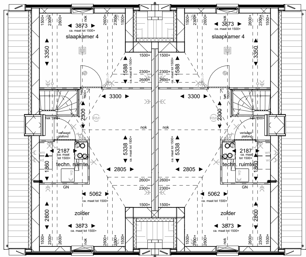
Tweede verdieping
