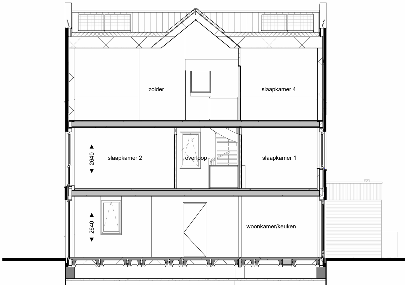
Doorsnede A-A
