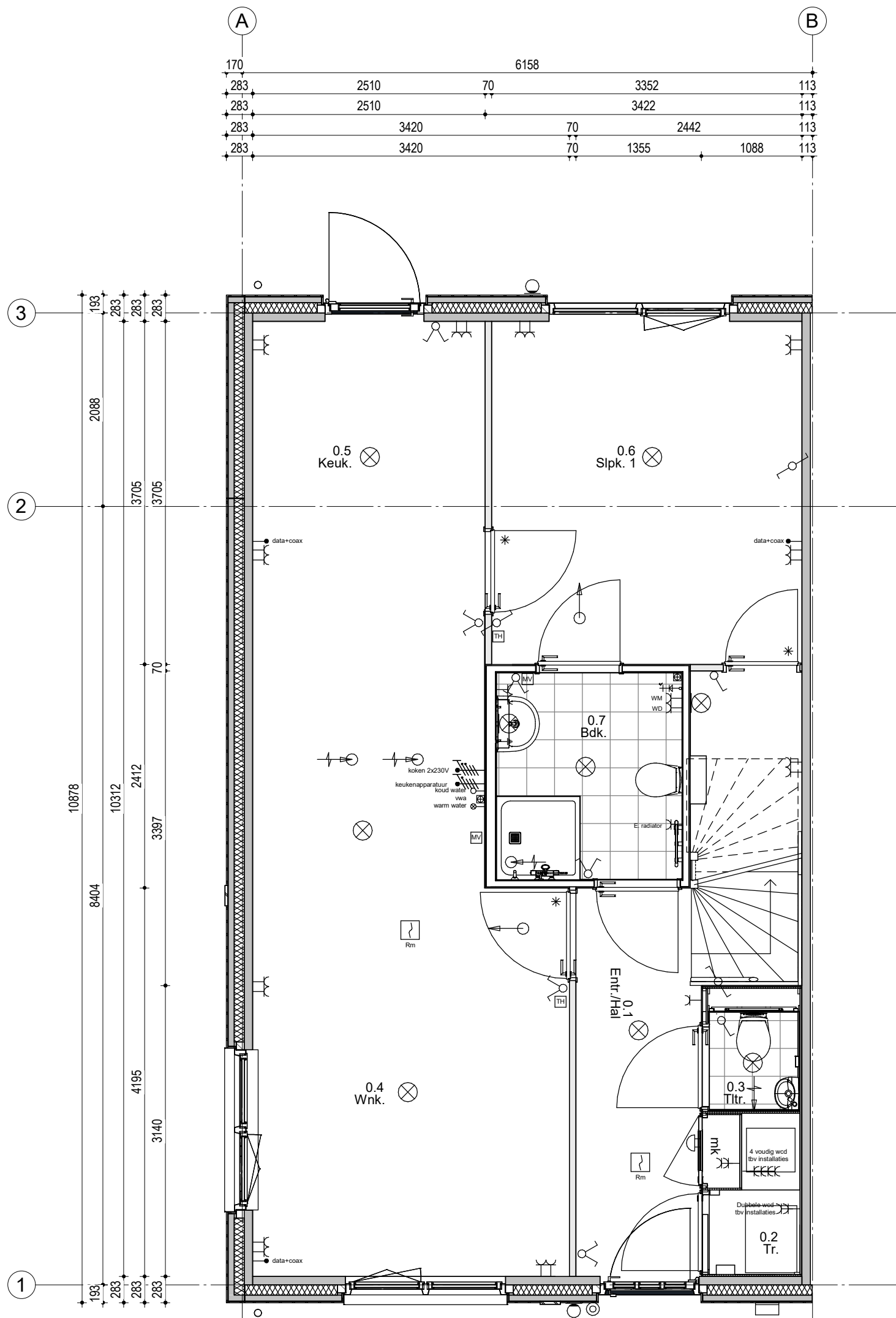
Woningtype 101 - 6158 Bouwnummer 201
