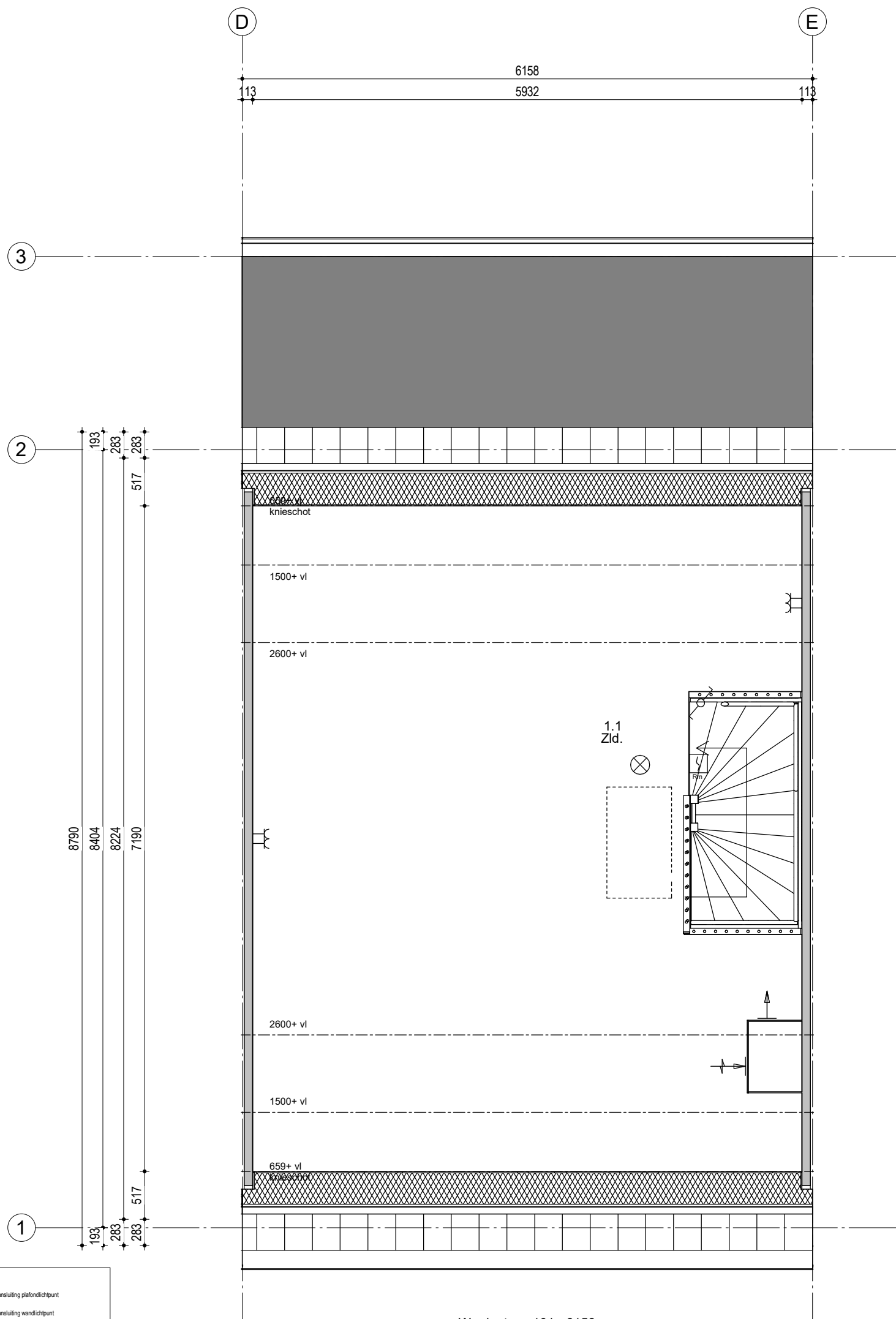
Woningtype 101 - 6158 Bouwnummer 204
