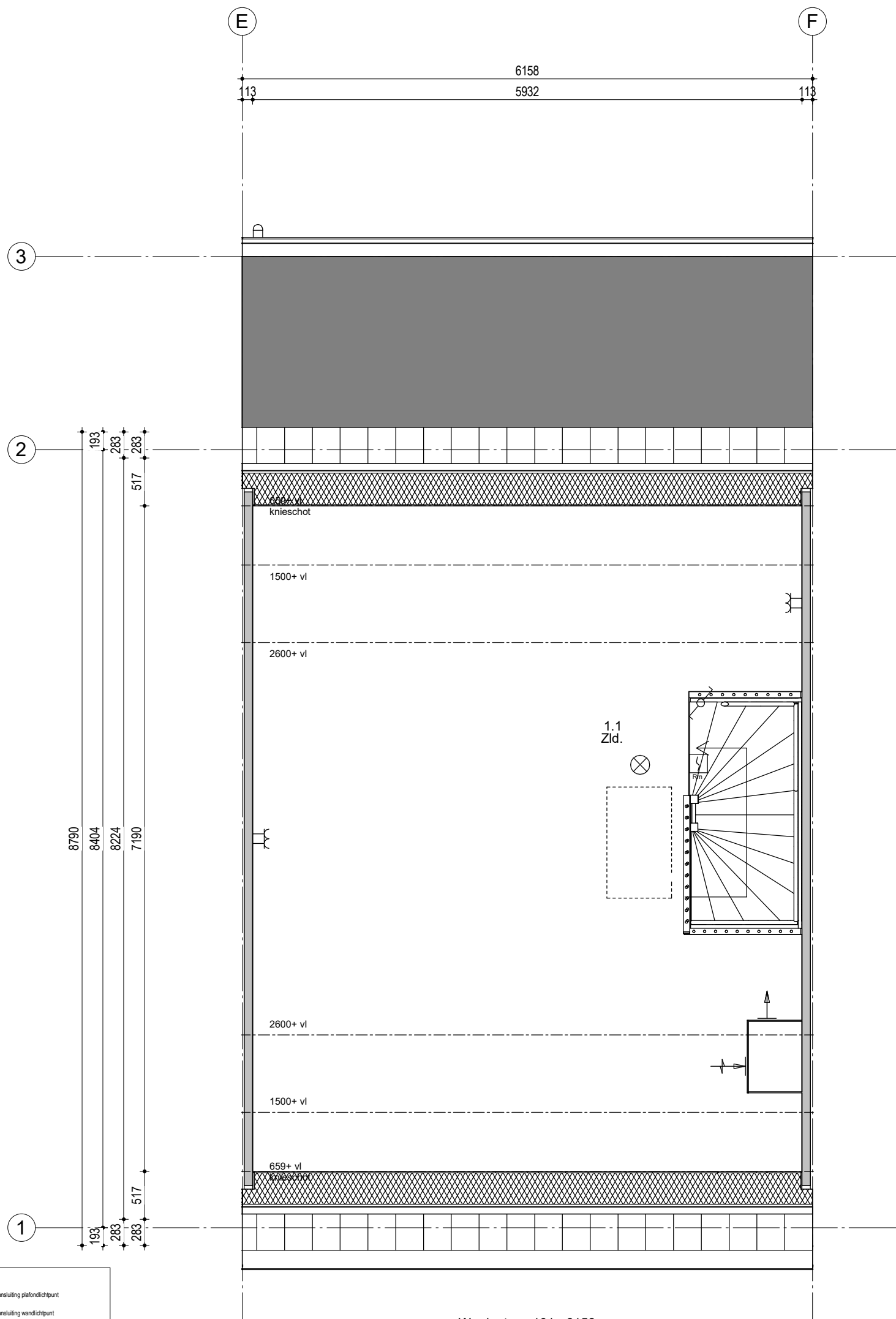
Woningtype 101 - 6158 Bouwnummer 205
