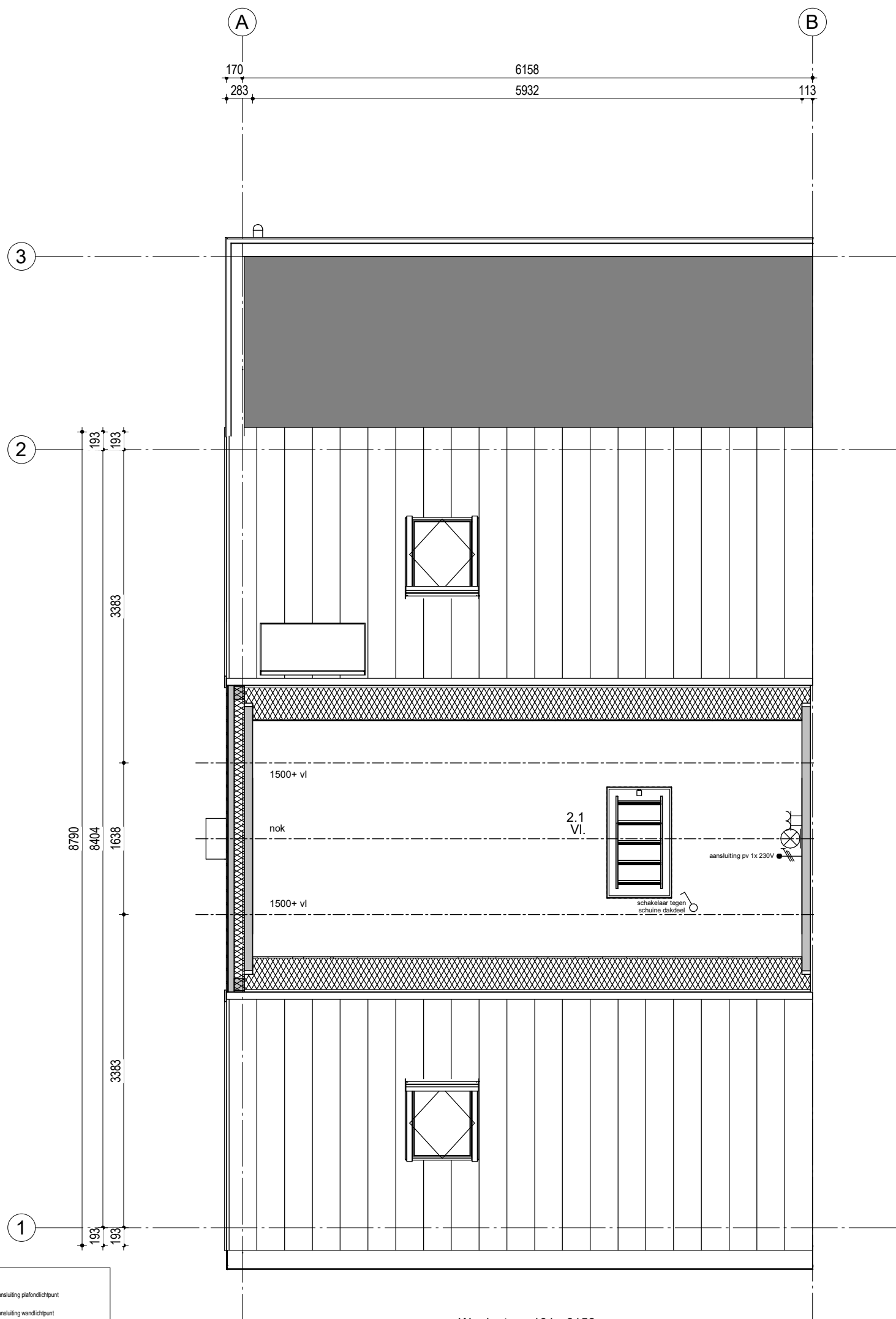
Woningtype 101 - 6158 Bouwnummer 201
