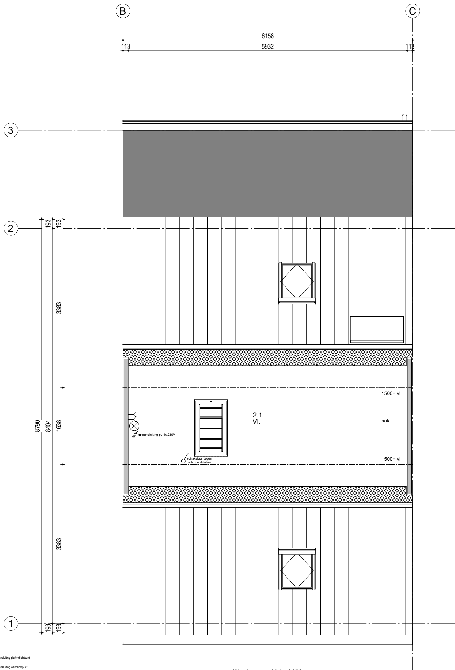
Woningtype 101 - 6158 Bouwnummer 202
