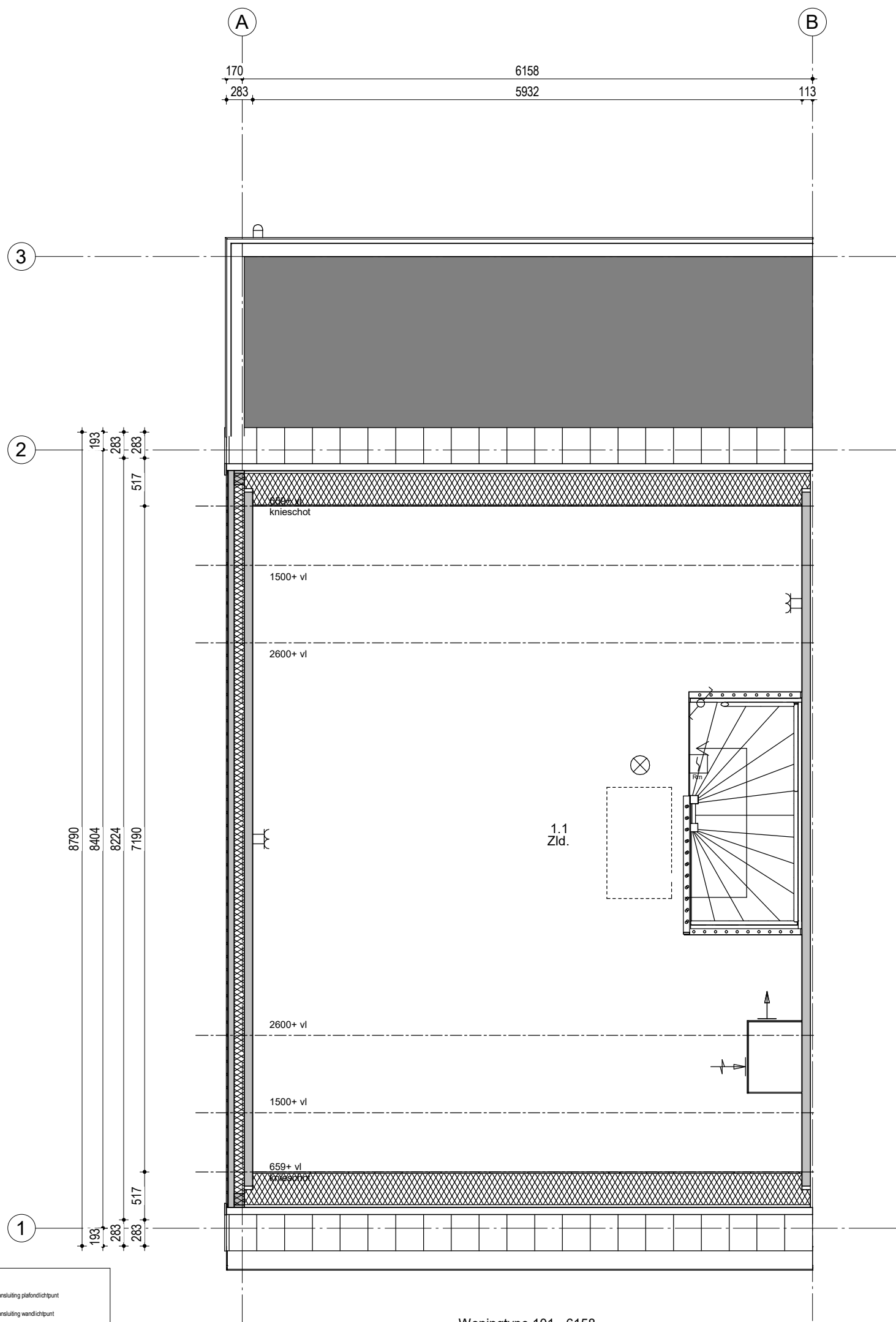
Woningtype 101 - 6158 Bouwnummer 201
