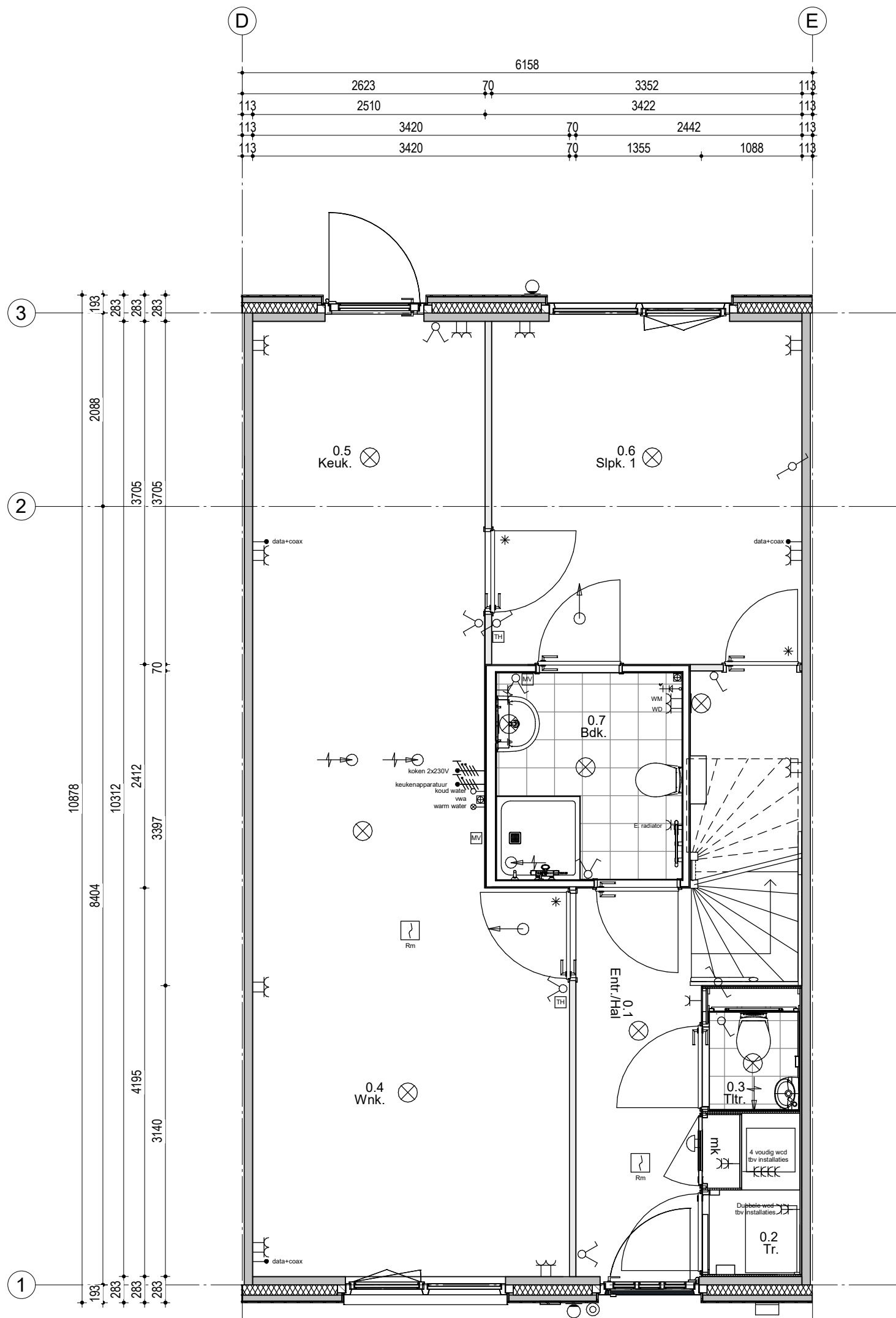
Woningtype 101 - 6158 Bouwnummer 204
