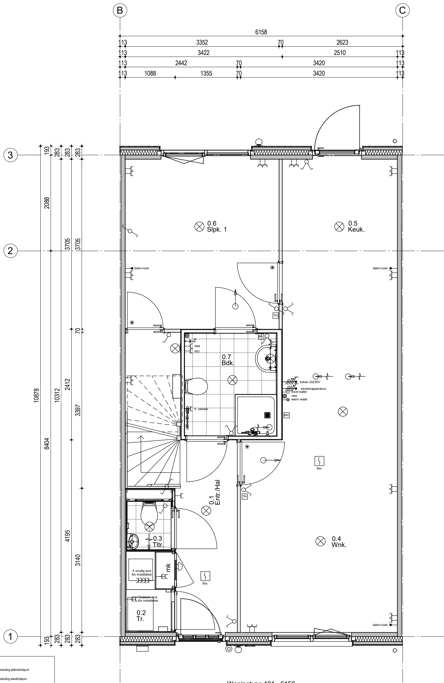
Woningtype 101 - 6158 Bouwnummer 202
