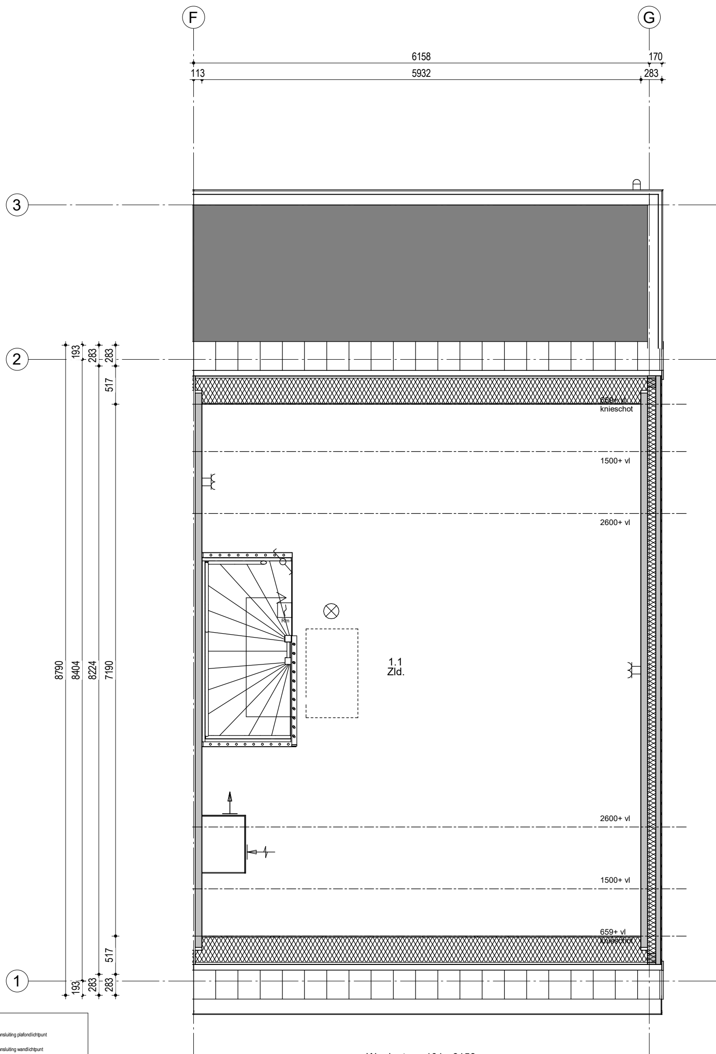
Woningtype 101 - 6158 Bouwnummer 206
