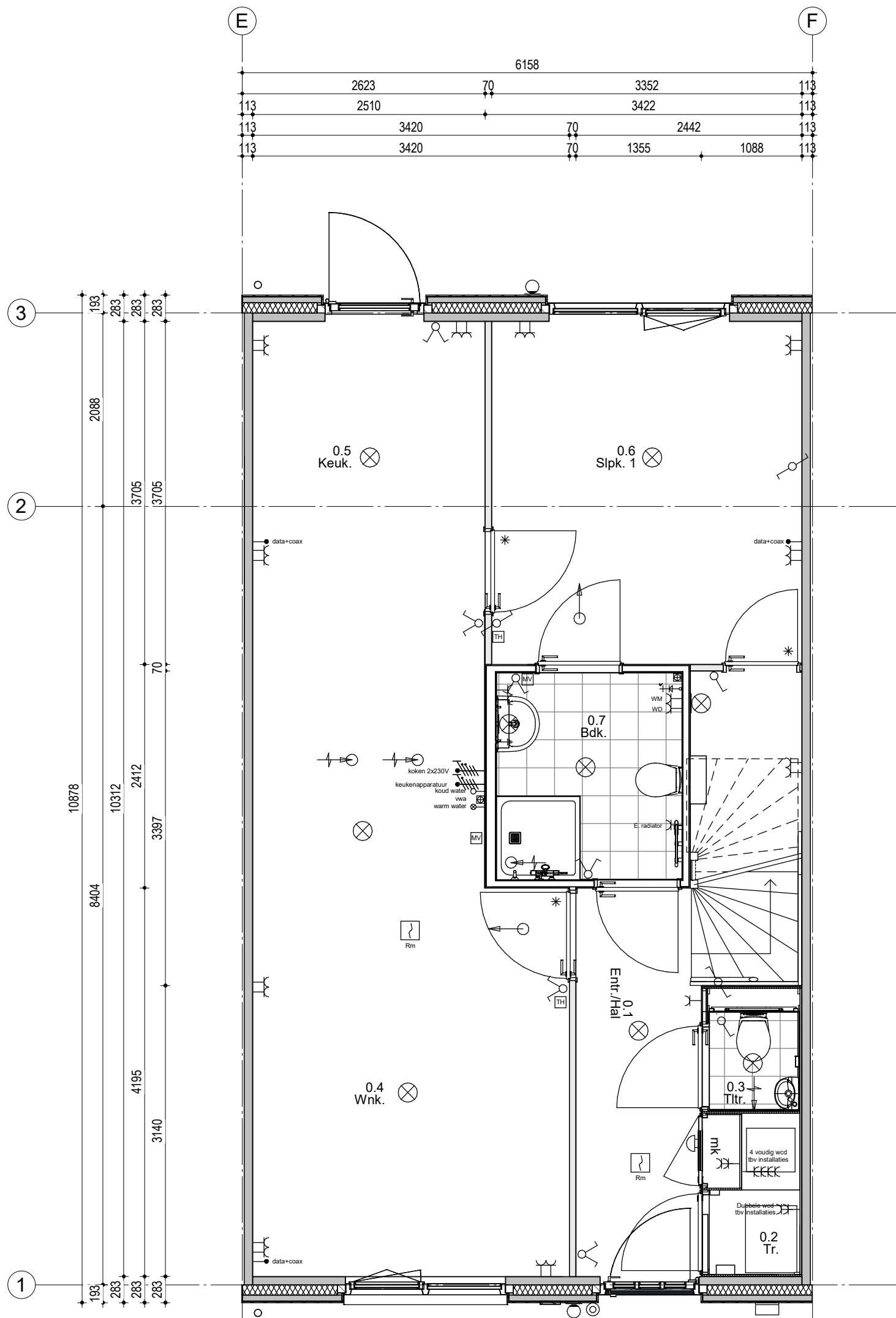
Woningtype 101 - 6158 Bouwnummer 205
