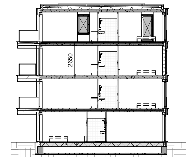
Doorsnede
