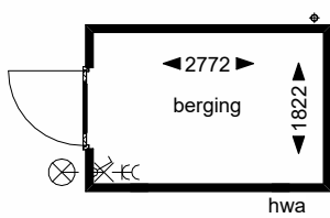
Begane grond
