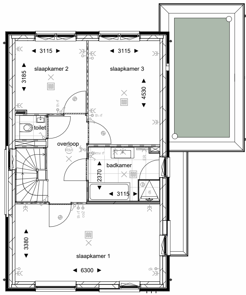
Eerste verdieping
