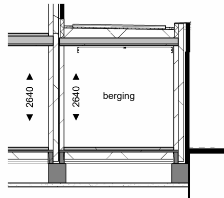
Doorsnede C-C
