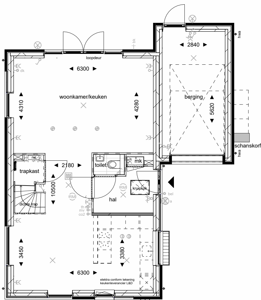
Begane grond
