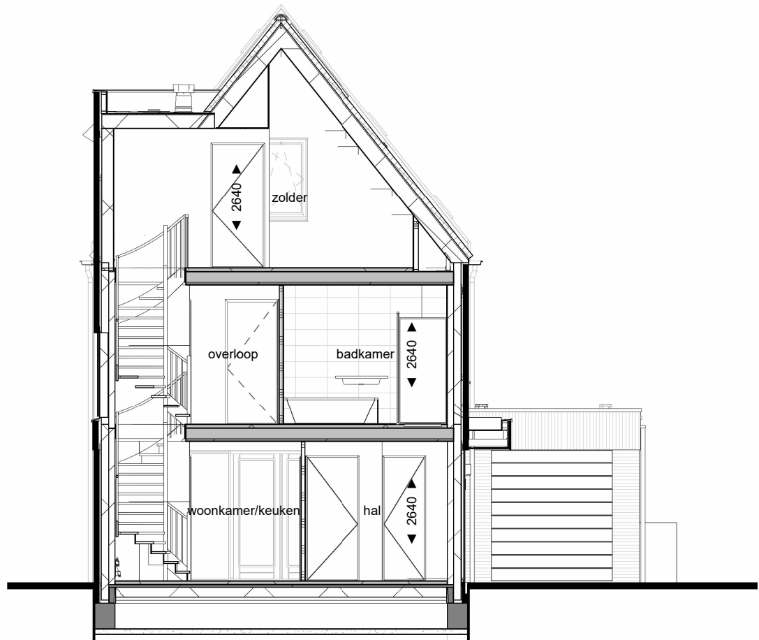
Doorsnede B-B
