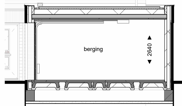
Doorsnede D-D
