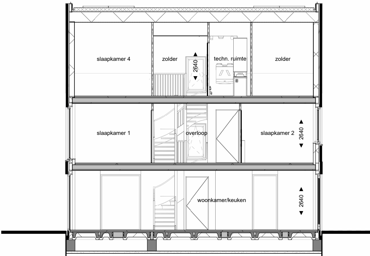
Doorsnede A-A
