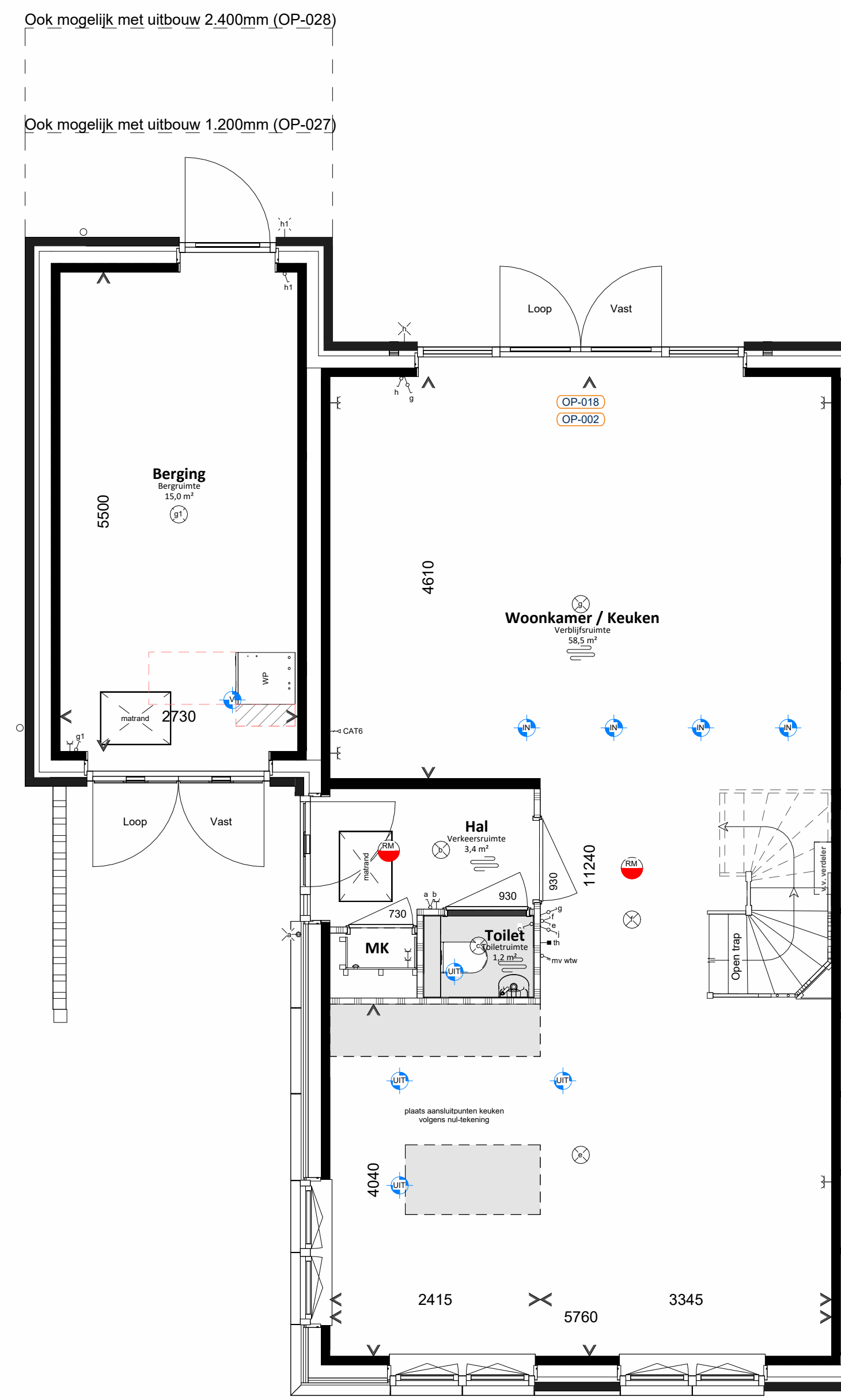
Begane grond 1:50
