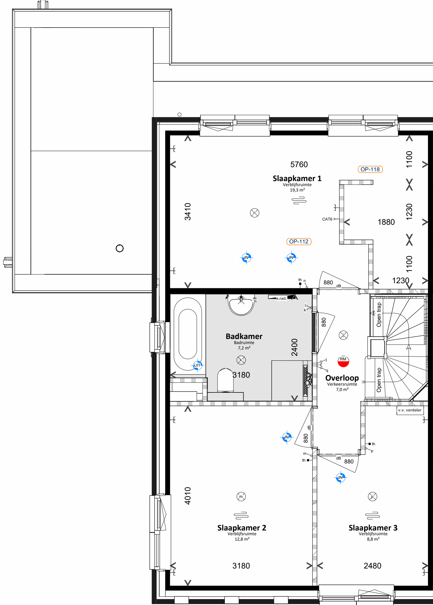
Eerste verdieping 1:50
