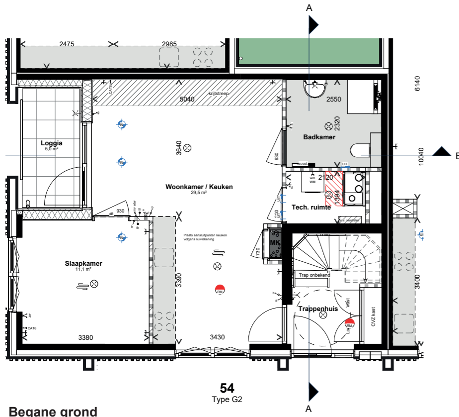
Begane grond
