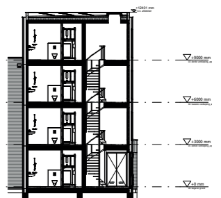
Doorsnede
